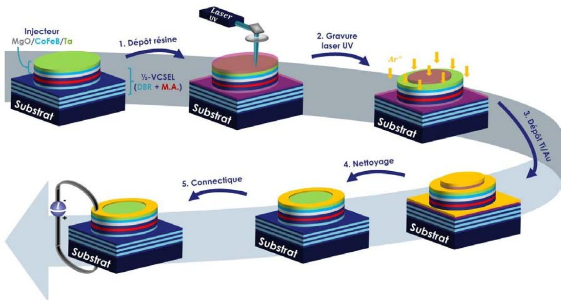
Figure 32 : 2 e partie de la fabrication des 1/2-VCSELs : étapes de métallisation et de lithographie optique. Notations : DBR : Réseau de Bragg, MA : milieu actif
