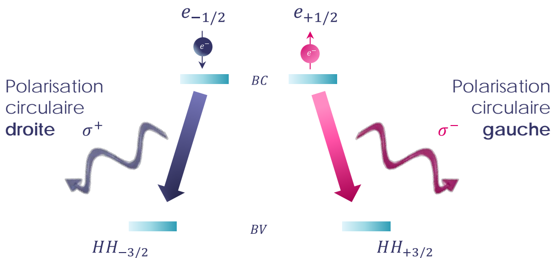
Figure 6 : Règles de sélection quantique dans un milieu confiné. Notations : \sigma^{+(\cdot)} : polarisation de la lumière en sortie de la source lumineuse, circulaire droite (gauche respectivement), LH (HH) : sous-bande des trous légers (lourd respectivement), e_{1/2} ( e_{-1/2} ) : électron de spin « up » (« down » respectivement). Les chiffres sur les flèches correspondent aux probabilités de désexcitation de l'électron de la bande de conduction vers la bande de valence (comparé à la transition CB\uparrow \rightarrow LH\downarrow )
