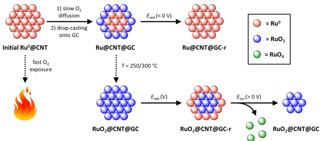
Scheme 4. Scénario proposé pour les processus d'oxydation / réduction se produisant à la surface des NPs de Ru et de RuO 2 déposées sur CNTs au cours de l'électrocatalyse
