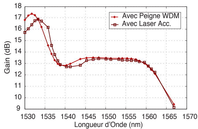
FIGURE 4.5 – Comparaison des méthodes de mesure du spectre de gain extraite de la référence [3].
