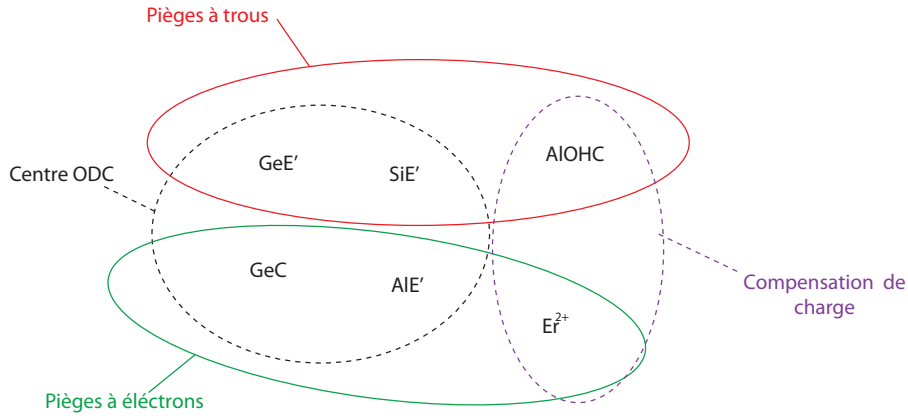
FIGURE 3.5 – Illustration des compétitions intervenant sur la présence des pièges
