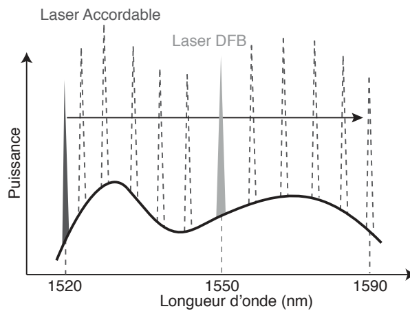
FIGURE 4.4 – Principe de la mesure de spectre de gain à l'aide de deux lasers
