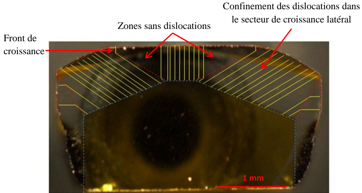
Figure 74 : Schéma du mécanisme de propagation des dislocations dans le diamant CVD intrinsèque avec un angle \theta égal à 38^\circ .
