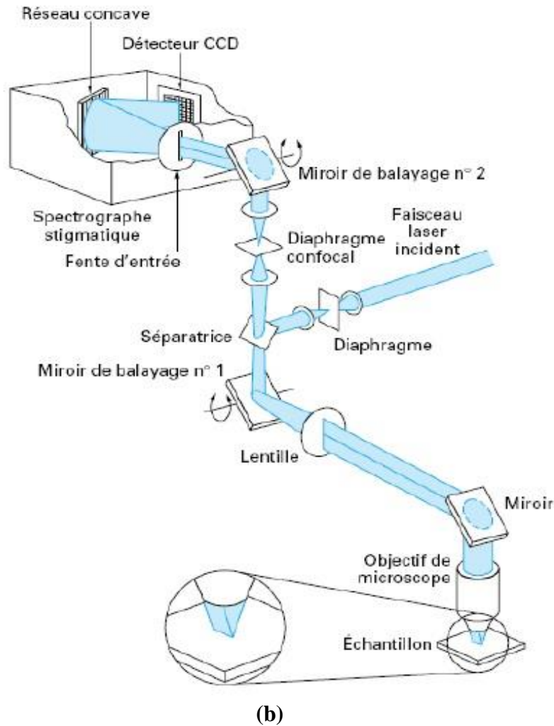
Figure 40 : (a) image de l'appareil Jobin-Yvon HR800 utilisé au LSPM, (b) schéma de fonctionnement d'un spectromètre Raman [261].
