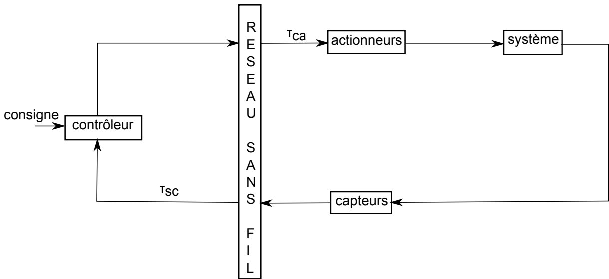
FIGURE 2.1 – Architecture d'un WNCs
