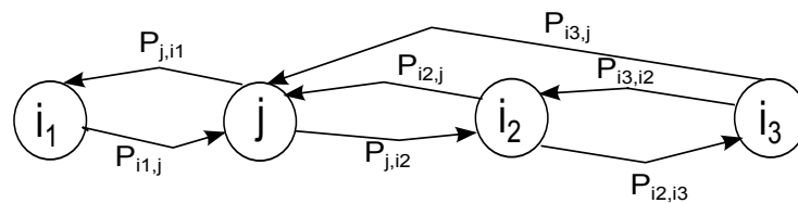
FIGURE 4.1 – Exemple d'une chaîne de Markov
