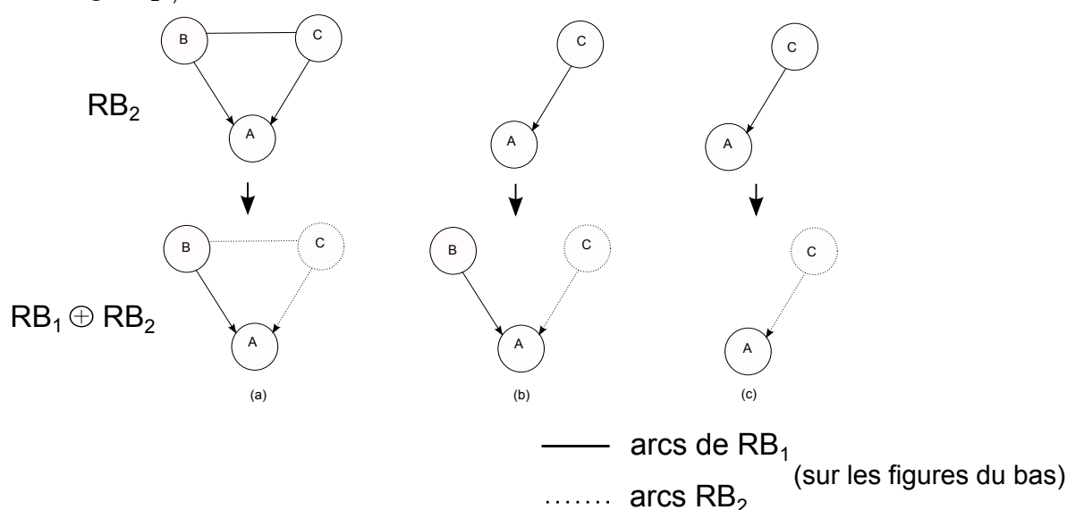
FIGURE 5.19 – Combinaison qualitative des réseaux bayésiens [HW13]
