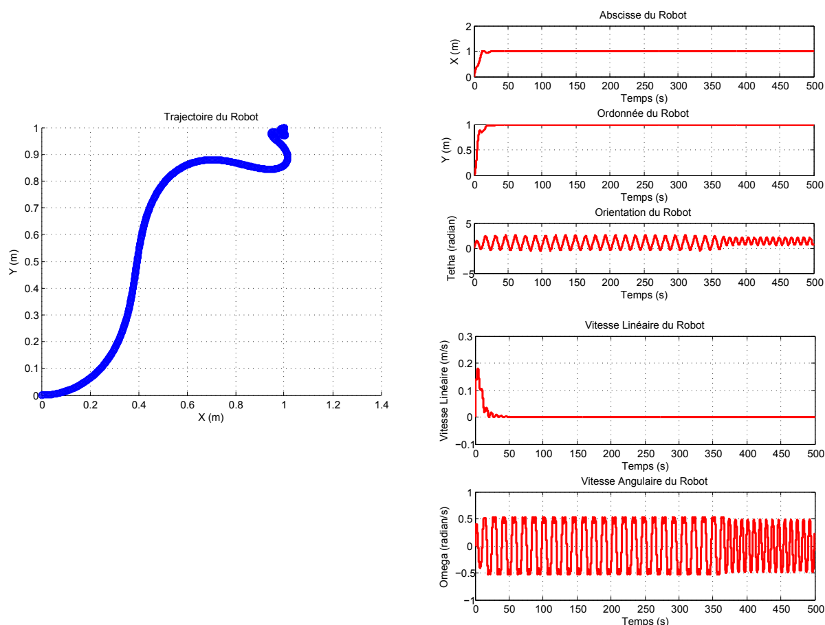
FIGURE 5.9 – Comportement du robot avec un retard de 2s
