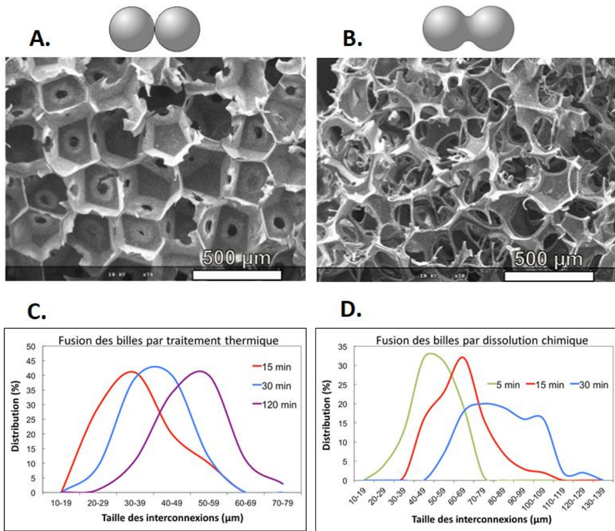
Figure 12. Scaffolds d'hybride gélatine-bioverre sans préfusion (A) et avec préfusion des billes (B). Élargissement des interconnexions de scaffolds d'hybride gélatine-bioverre en préfusionnant les billes par traitement thermique (C) ou par dissolution chimique partielle (D). D'après les travaux de Lao et al. [66].
