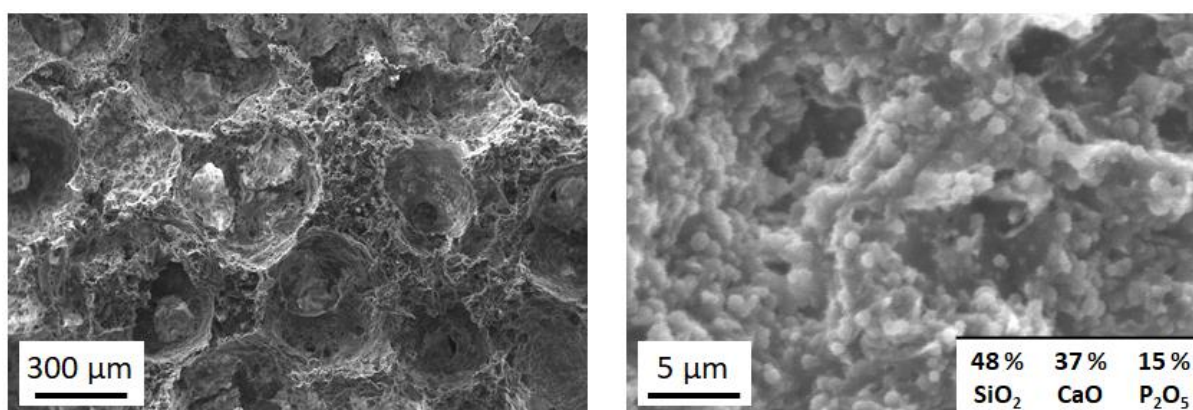
Figure 86. Clichés MEB d'un scaffold d'un hybride de composition massique 35 % PCL - 35 % PHB - 30 % bioverre avant (à gauche) et après (à droite) immersion dans le SBF pendant 3 jours.
