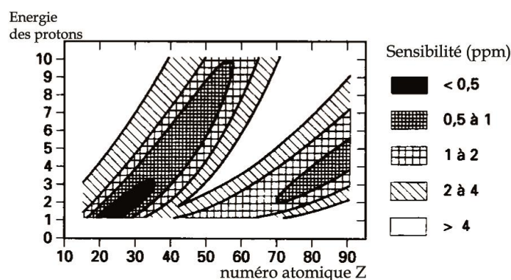
Figure 19. Limite de détection en PIXE avec des protons en fonction de leur énergie et de la composition de la cible.
