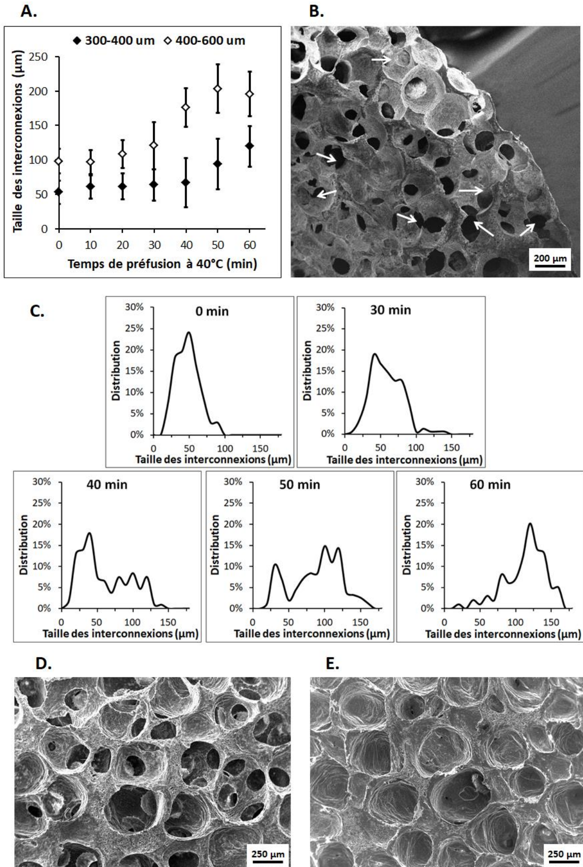
Figure 47. Taille des interconnexions des scaffolds hybrides PCL-bioverre en fonction du temps de préfusion des billes à 40°C (A). Scaffold d'un hybride PCL-bioverre fabriqué par préfusion des billes à 40°C pendant 90 min (B) ; les flèches blanches pointent des interconnexions qui se touchent. Distribution des tailles des interconnexions en fonction du temps de préfusion à 40°C des billes 300-400 µm (C). Les scaffolds fabriqués par préfusion à 45°C (D) ont une interconnectivité plus homogène en comparaison avec ceux obtenus à 40°C qui possèdent des zones faiblement interconnectées (E).
