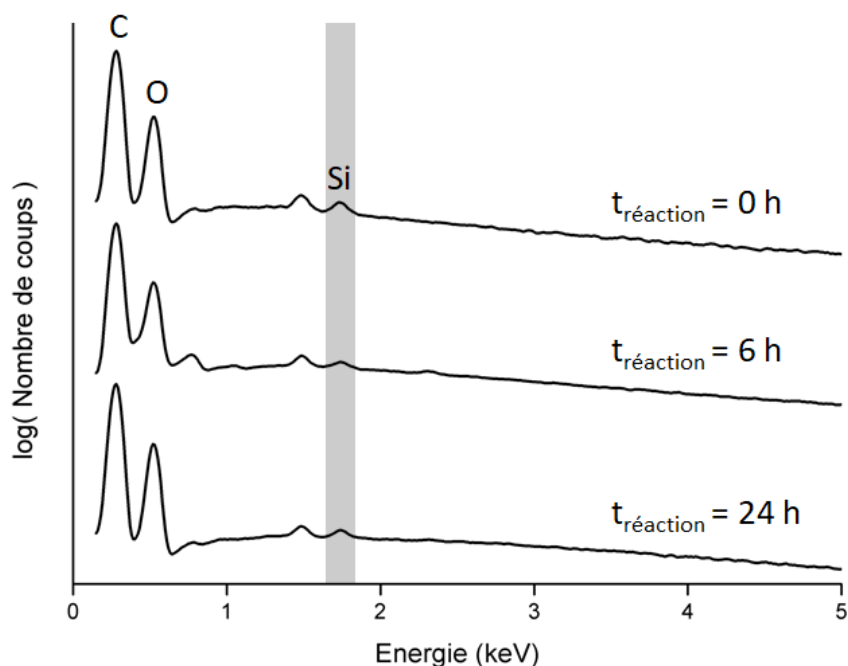
Figure 97. Spectres d'émission des rayons X obtenus par analyse EDX du PCL après la réaction avec le GPTES pendant un temps t .
