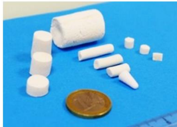
Figure 13. Exemples de structures réalisables grâce au procédé de fabrication. Scaffolds d'hybride gélatine-bioverre avec des structures mixtes dense-poreuses (A). Scaffold d'hybride polycaprolactone-bioverre avec gradient de porosité (B). Scaffolds d'hybride aux formes diverses et variées (C).
