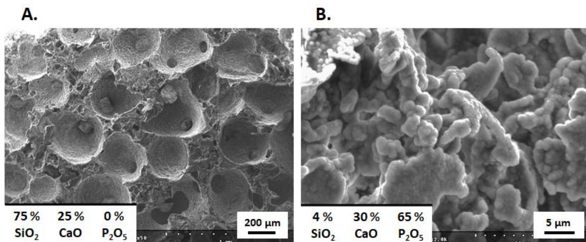
Figure 35. Scaffold d'un hybride PCL-bioverre synthétisé à partir de \text{CHCl}_3 avant (A) et après interaction avec le SBF pendant 3 jours (B). Les compositions massiques sont déterminées en EDX ( n = 3 ), les erreurs relatives sont inférieures à 1 %.
