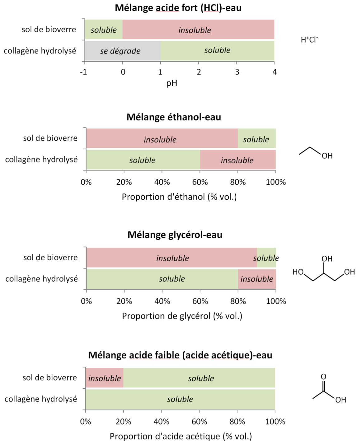
Figure 28. Solubilité du sol de bioverre et du collagène hydrolysé dans différents mélanges de solvants.
