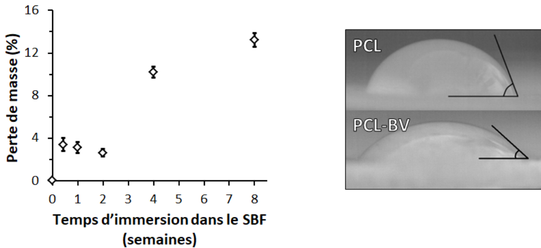
Figure 63. Dégradation des scaffolds d'un hybride PCL-bioverre dans le SBF (à gauche) et exemples de mouillabilité de pastilles en PCL pur et en hybride PCL-bioverre (à droite).
