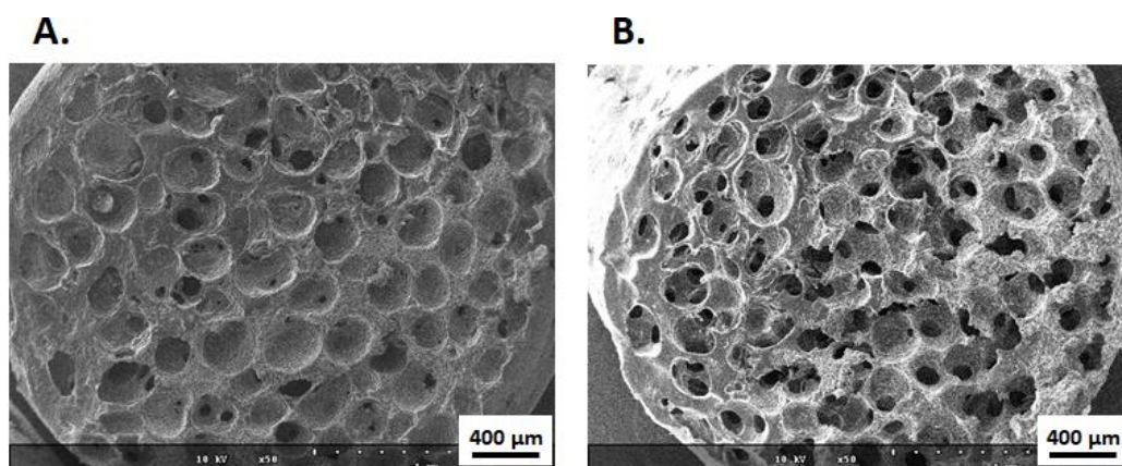
Figure 44. Scaffolds d'un hybride PCL-bioverre fabriqués en centrifugeant à 3900 (à gauche) ou à 6000 tr/min (à droite).
