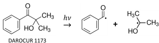
Figure 93. Réaction de dissociation du 2-hydroxy-2-méthylpropiophénone ou DAROCUR 1173.
