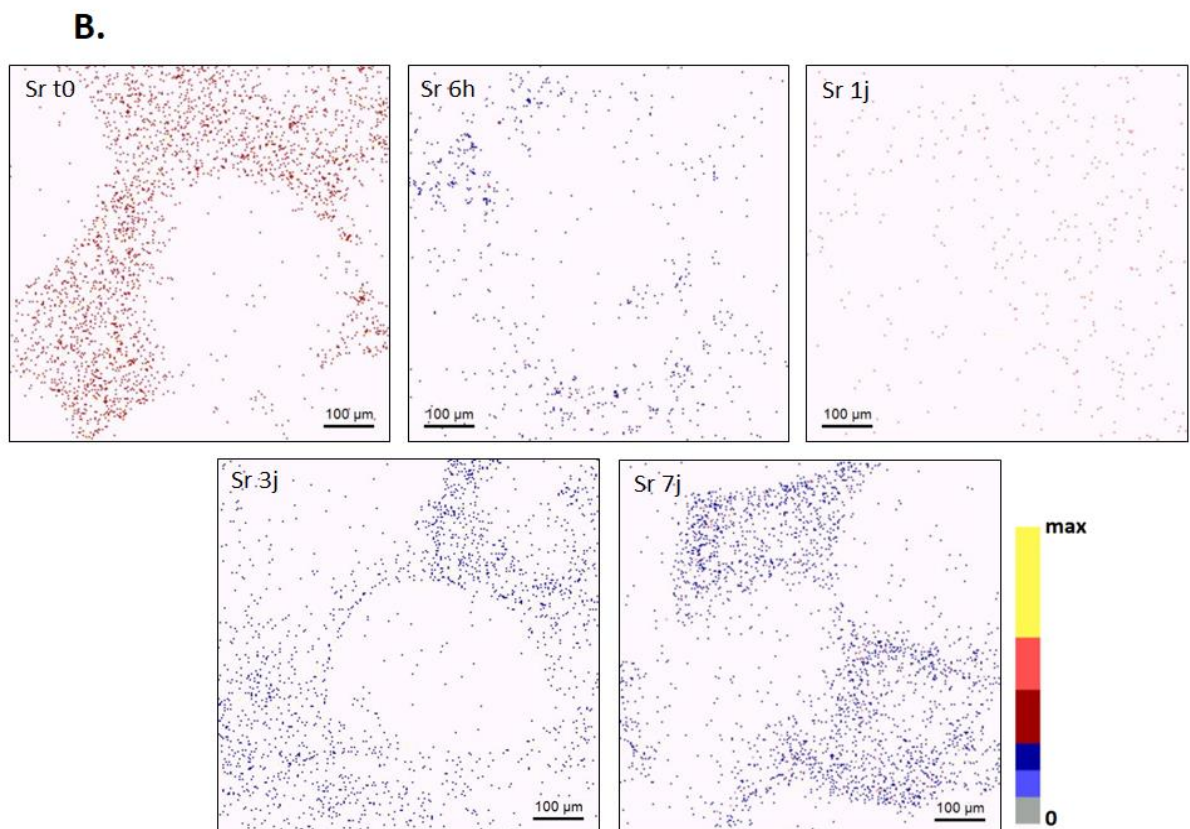
Figure 76. Cartographies élémentaires du scaffold hybride PCL-Sr5 acquises par micro-faisceau d'ions (PIXE) : cartographies du Si, Ca, P et Sr après 3 jours d'interaction (A) et suivi de la distribution du Sr au sein des coupes de scaffolds en fonction du temps d'interaction (B).
