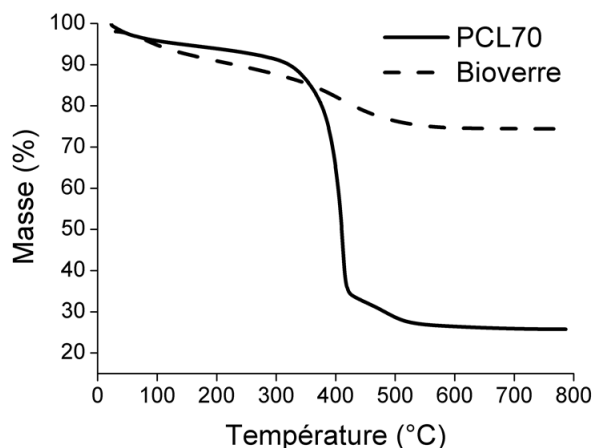
Figure 54. Analyse thermogravimétrique de l'hybride PCL-bioverre (PCL70) et du bioverre pur.
