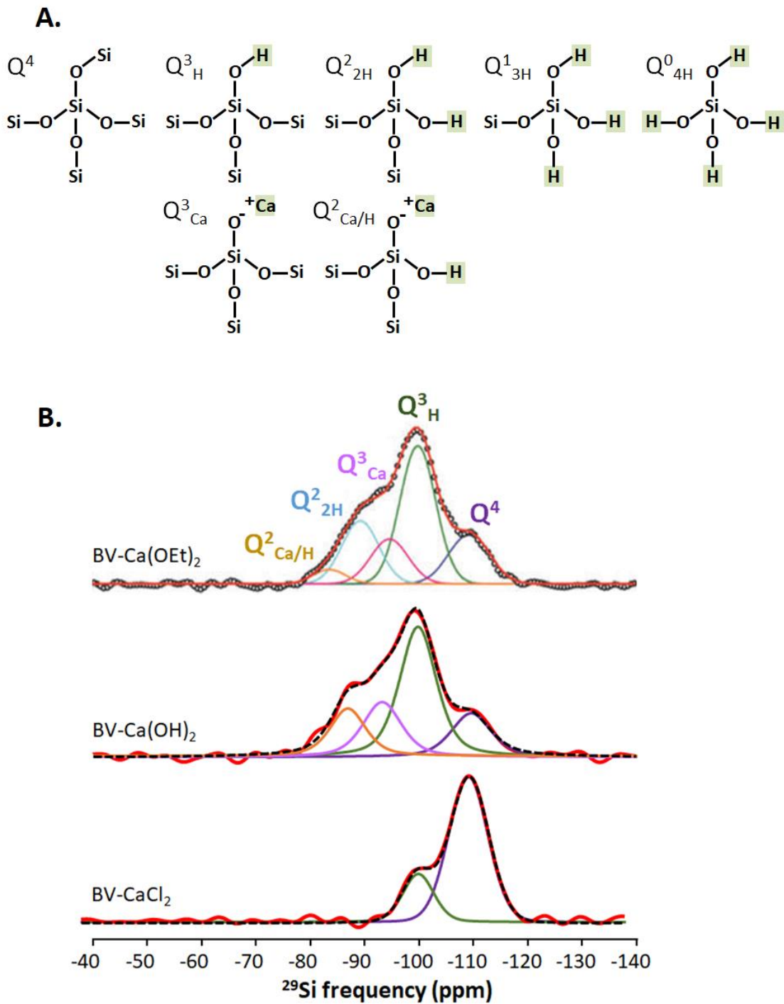
Figure 38. Représentation des espèces Q^n (A). Distributions des espèces Q^n dans les bioverres BV- \text{Ca}(\text{OEt})_2 , BV- \text{Ca}(\text{OH})_2 et BV- \text{CaCl}_2 obtenues par RMN solide du silicium 29 (B).
