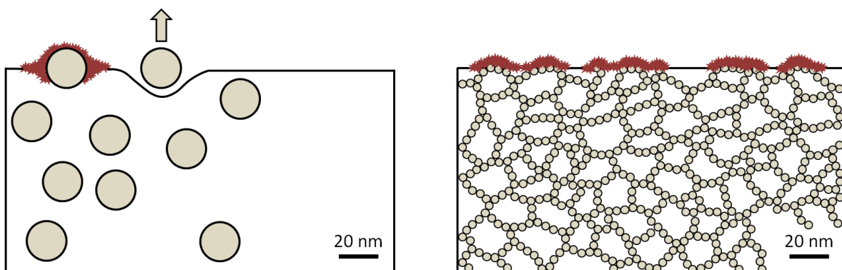
Figure 6. Schéma structural d'un nanocomposite (à gauche) et d'un hybride (à droite). L'apatite est représentée en rouge.
