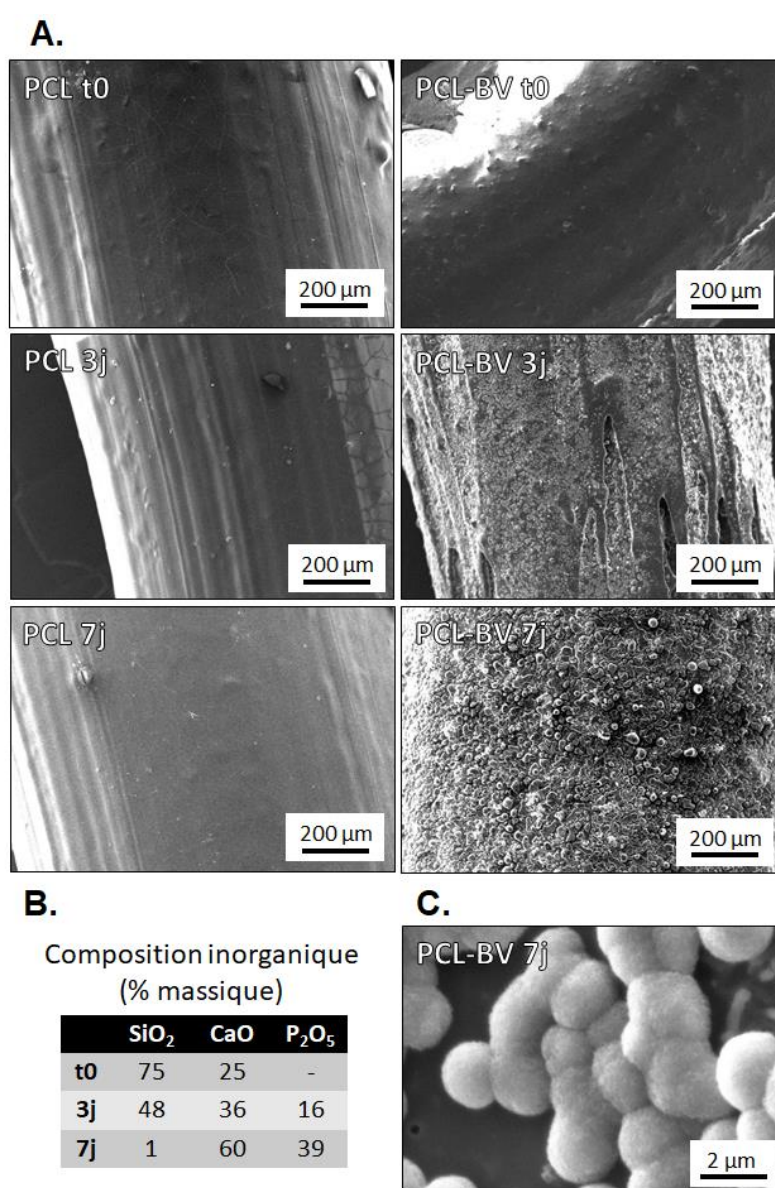
Figure 107. Évolution de l'état de surface de barreaux imprimés en PCL pur et en hybride PCL-bioverre (noté PCL-BV) au cours de l'interaction avec le SBF, vue au MEB (A). Évolution de la composition inorganique du barreau hybride PCL-bioverre au cours de l'interaction, déterminée par EDX (B). Cliché MEB des précipités formés en surface du barreau hybride après 7 jours d'immersion (C).
