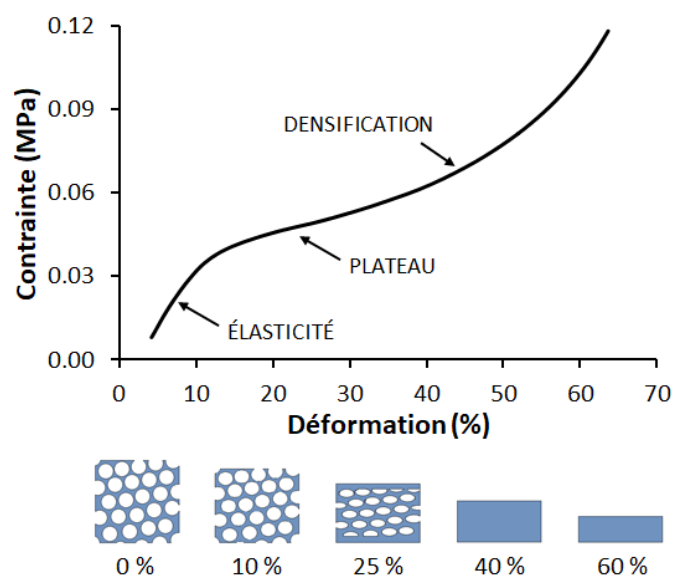
Figure 58. Courbe de contrainte-déformation obtenue par compression du scaffold sec.
