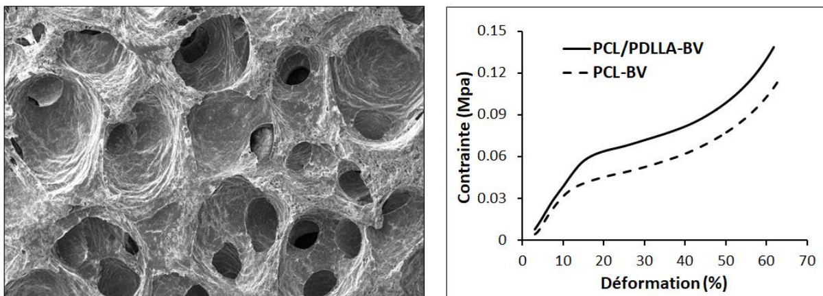
Figure 87. À gauche, cliché MEB d'un scaffold d'un hybride de composition massique 49 % PCL - 21 % PDLLA - 30 % bioverre. À droite, courbes de contrainte-déformation obtenues par compression des scaffolds de l'hybride contenant du PDLLA (noté PCL/PDLLA-BV) et de l'hybride n'en contenant pas (noté PCL-BV).
