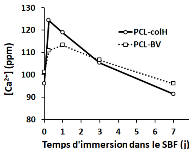
Figure 78. Évolution de la concentration en ions calcium dans le SBF au cours de l'interaction avec les scaffolds hybrides PCL-BV et PCL-colH.
