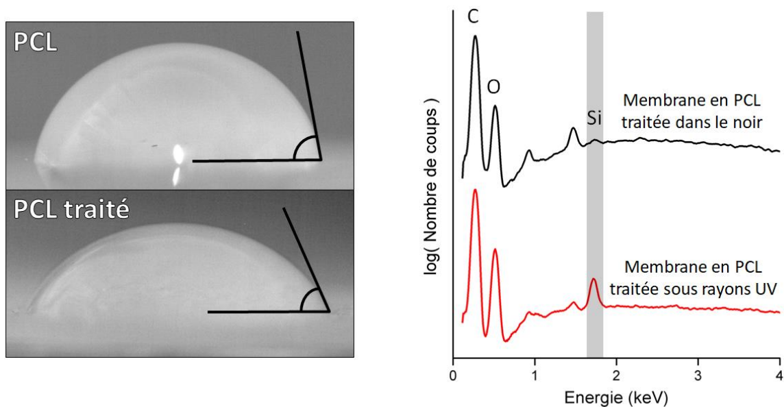
Figure 91. Exemples de mouillabilité de membranes en PCL pur avant et après traitement dans l'eau oxygénée (à gauche). Spectres d'émission des rayons X obtenus par analyse EDX des membranes en PCL fonctionnalisées avec le triéthoxysilane de vinyle (à droite).
