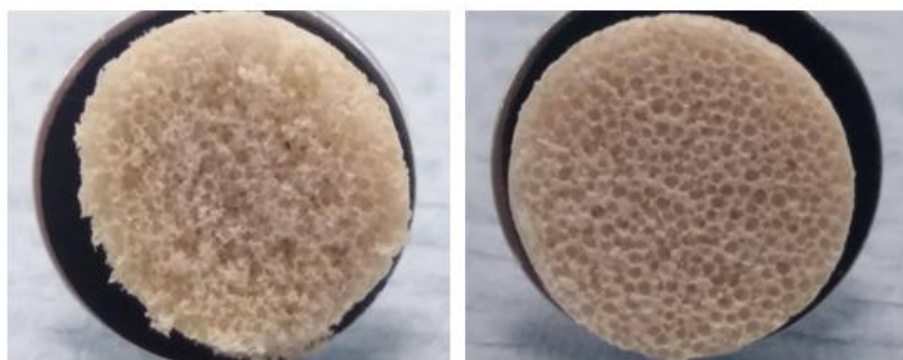
Figure 48. Coupe des scaffolds PCL40 (à gauche) et PCL50 (à droite).
