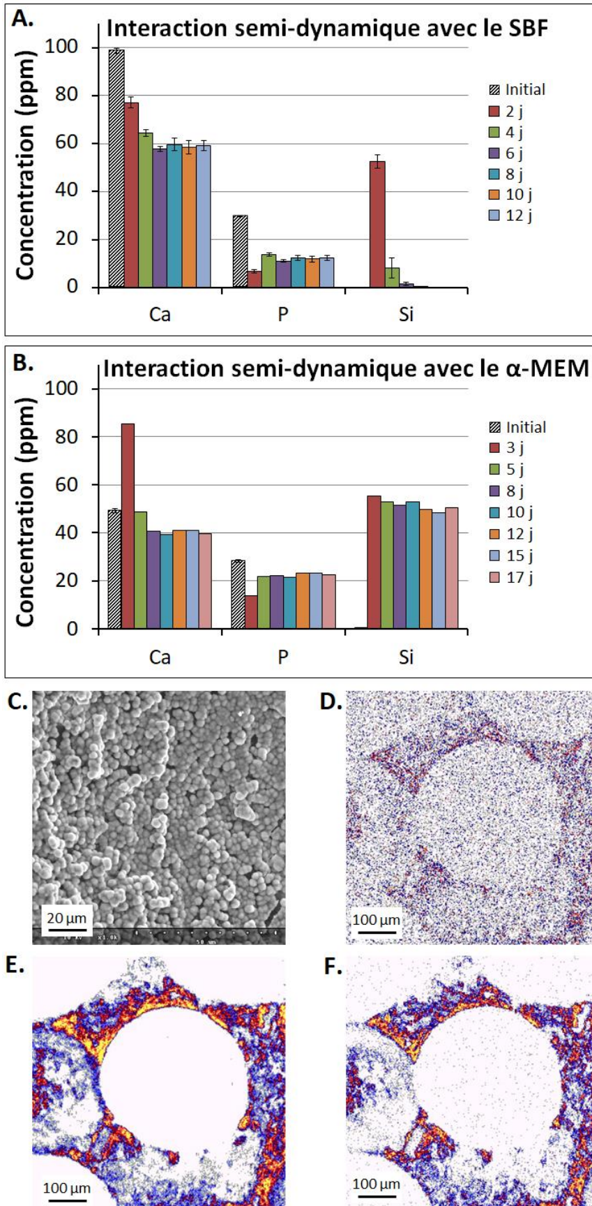
Figure 61. Concentrations déterminées par ICP-AES en Si, Ca et P dans le SBF (A) et dans le milieu de culture (B) après interaction avec un scaffold. Scaffold après 12 jours d'interaction avec du SBF vu au MEB (C) et en PIXE (D-F).
