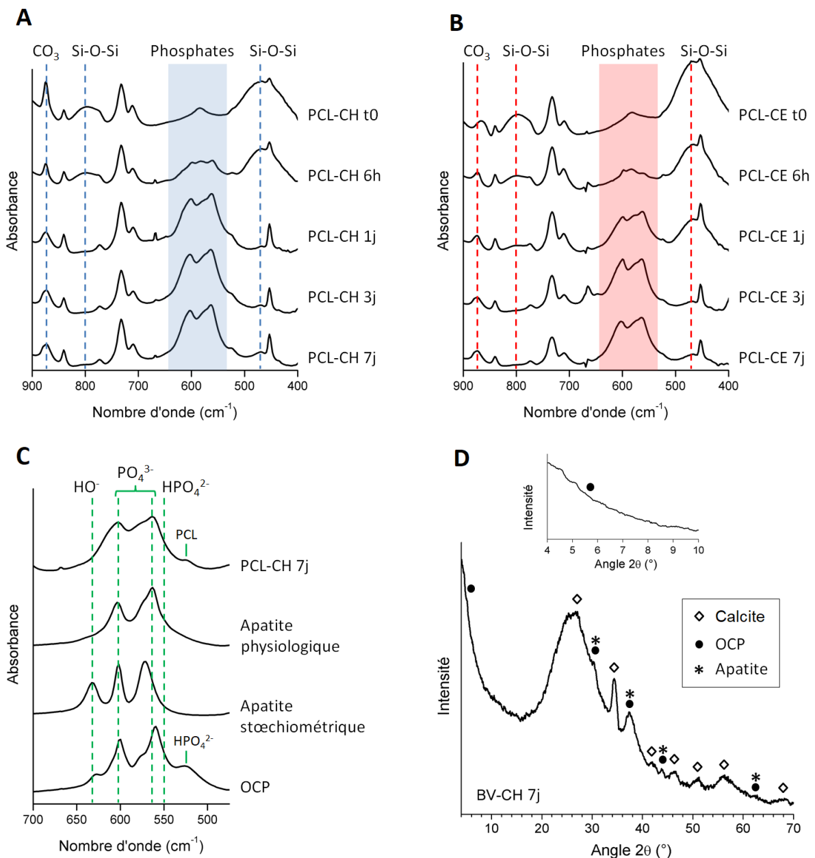
Figure 42. Évolution des spectres IR des scaffolds hybrides PCL-bioverre PCL-CH (A) et PCL-CE (B) au cours de leur interaction avec le SBF. Comparaison du spectre IR du PCL-CH interagi 7 jours avec les spectres de différents phosphates de calcium (C). Diffractogramme du bioverre BV-CH interagi 7 jours (D).
