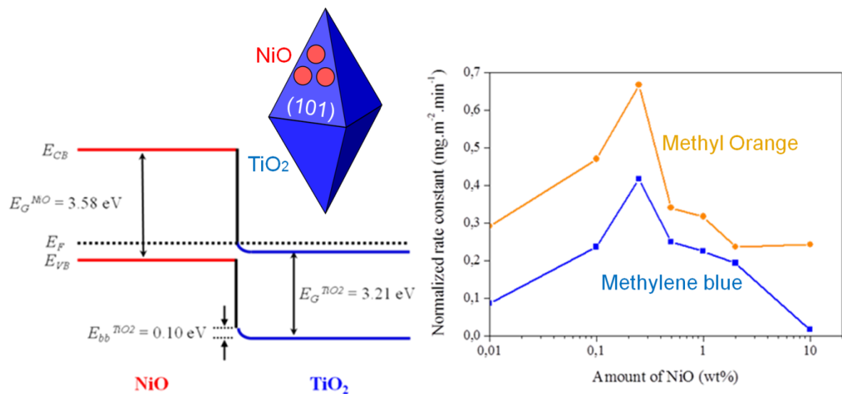
Figure 4 : Alignement des bandes d'énergie et propriétés photocatalytiques des systèmes NiO/(101)-anatase-TiO 2 préparés par la méthode de dépôt chimique en fluide supercritique.
