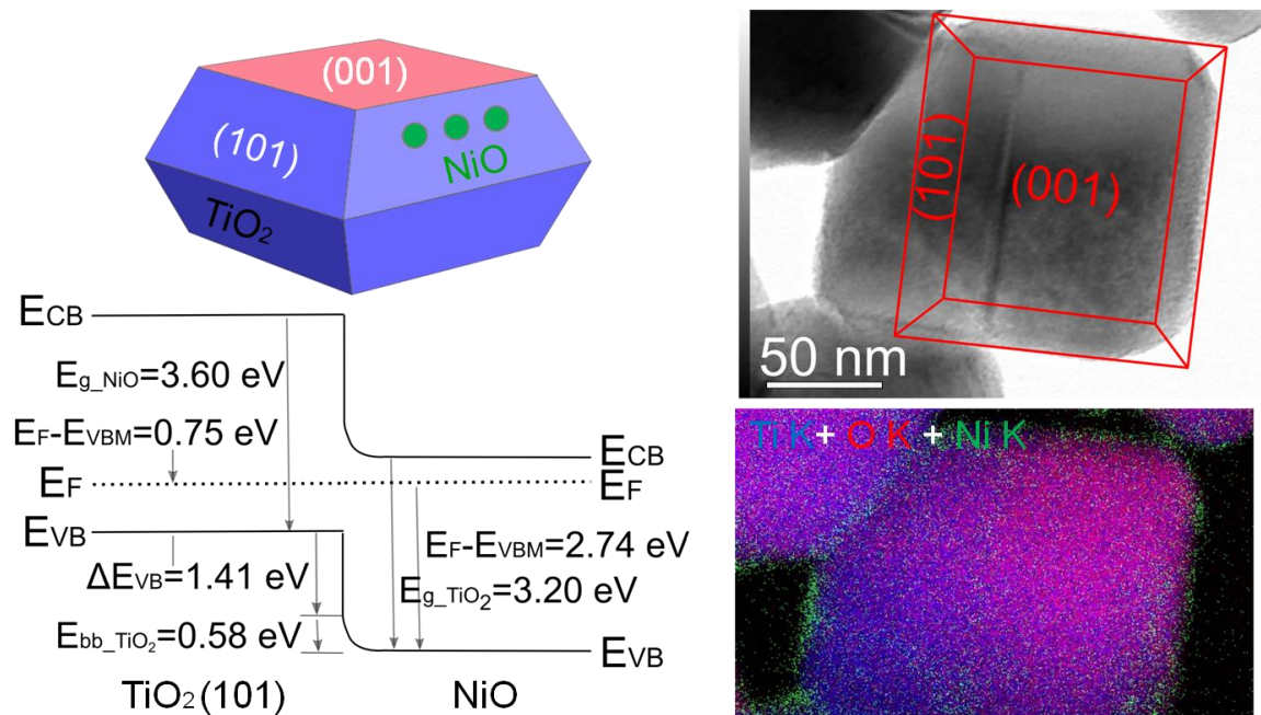
Figure 5 : Dépôt sélectif photoinduit de NiO sur les facettes (101) de nanocristaux d'anatase co-exposant des facettes (001) et (101).
