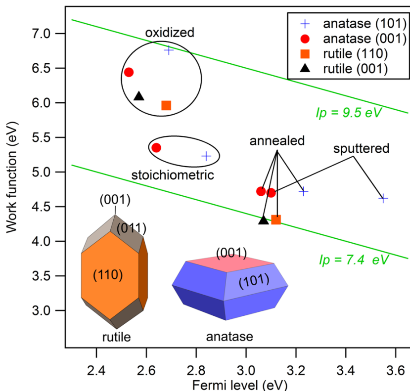
Figure 2 : Travail de sortie de cristaux de TiO 2 anatase et rutile d'orientations et stoechiométries variées.
