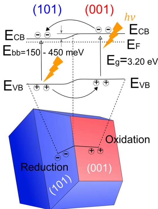
Figure 1 : Processus de séparation des porteurs de charges dans des cristallites d'anatase co-exposant des facettes (001) et (101) déduit des diagrammes d'alignement des bandes d'énergie.
