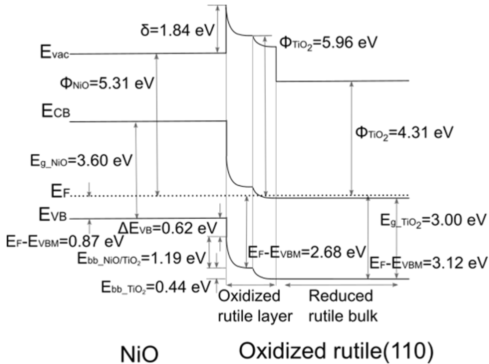
Figure 3 : Alignement des bandes d'énergie pour la surface (110) du p-NiO/n-TiO 2 rutile oxydé déterminé à partir des expériences d'interface.
