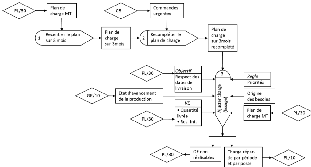
Figure 23. Exemple de Réseau GRAI (Vallespir et Doumeingts, 2002)
