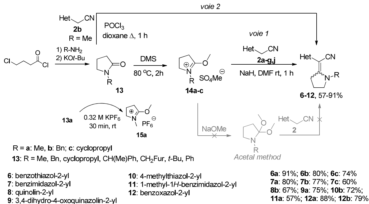
Schéma 2. Synthèse de 2-azahétéaryl-2-(1-alkylpyrrolidin-2-ylidène)acétonitriles 6-12.
