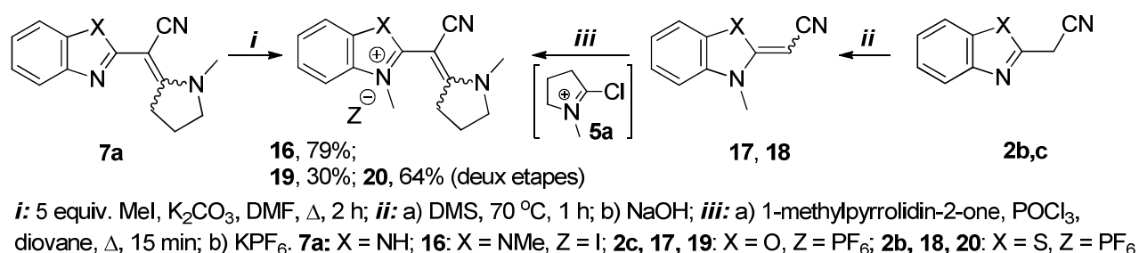
Schéma 3. 2-(Pyrrolidin-2-ylidène)acétonitriles substitués par des benzazoles quaternisés 16, 19, 20 .
