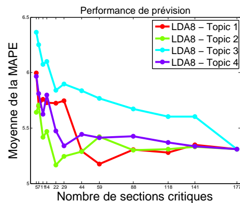
Fig. 4.7.: Évolution des performances associées aux jeux de variables produits par les K_{lda} = 4 motifs en fonction du nombre n de sections sélectionnées : a) à un horizon de 30 minutes sans distinction des conditions de trafic. b) à un horizon de 90 minutes sans distinction des conditions de trafic. c) à un horizon de 30 minutes en conditions non récurrentes. d) à un horizon de 90 minutes en conditions non récurrentes.
