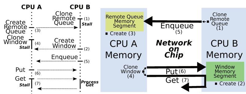
FIGURE A.2 – Utilisation des segments mémoires et des protocoles
