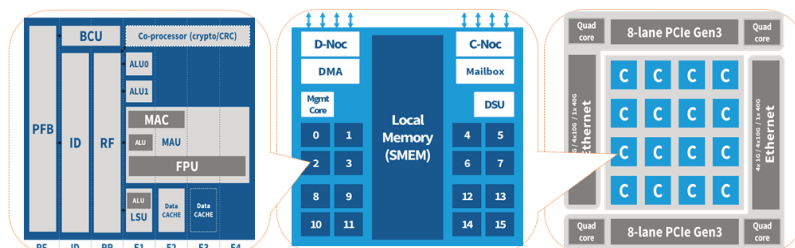
FIGURE A.1 – Le processeur MPPA ® de Kalray
