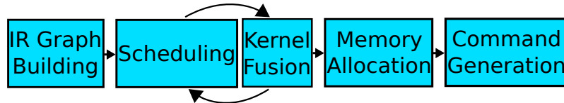
FIGURE A.3 – Vérification et optimisation du graphe OpenVX applicatif - vxVerifyGraph [G + 17]
