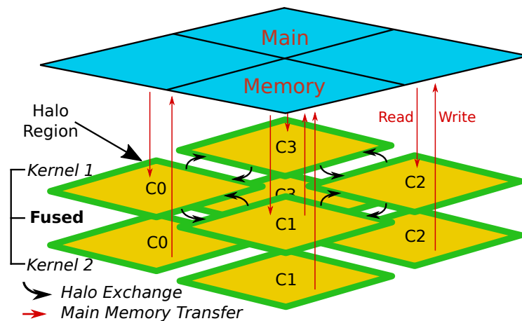
FIGURE A.4 – Automatisation de la fusion de nœuds standard OpenVX à l'exécution
