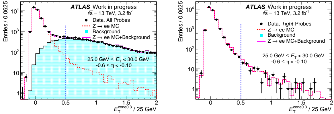
FIGURE V.2 Distribution d'isolation des électrons en données (noir), pour le bruit de fond (bleu clair) et en simulation (rouge hachuré). À gauche, la distribution d'isolation des probes reconstruits est montrée, à gauche, pour des probes identifiés. La ligne bleu foncée hachurée indique la définition d'échantillon du signal et de contrôle.
