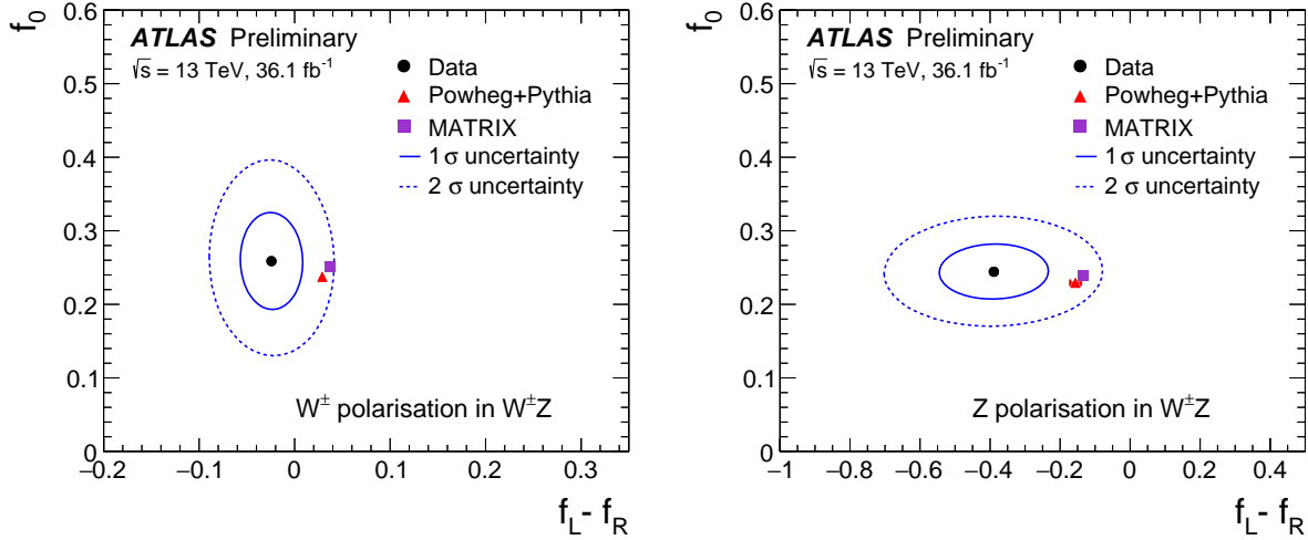
FIGURE VIII.1 Résultats de la mesure de la polarisation des bosons W (gauche) et Z (droit) dans des événements W^\pm Z et leurs incertitudes. Les résultats sont comparés avec les prédictions de POWHEG+PYTHIA et MATRIX
