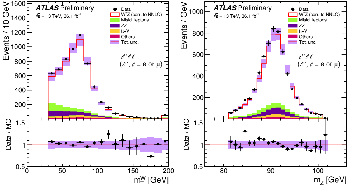
FIGURE VI.1 Distributions cinématiques du signal (blanc) et du bruit de fond (coloré). Les points noirs représentent les données. À gauche, la masse transverse du boson W est montrée et à droite, la masse invariante du boson Z .
