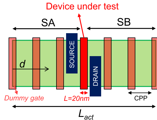
Figure C.12: Illustration d'un layout typique d'un transistor. SA/SB sont les paramètres de distance entre la grille et le bord de la zone active de part et d'autre du canal et W est la largeur d'active. La longueur d'active L_{act} dépend du nombre de pas de fausses grilles (CPP) utilisé.
