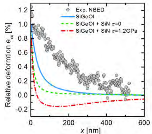
Figure C.8: Comparaison entre le profil de déformation expérimental et plusieurs simulations mécaniques dans le domaine élastique. La simulation ne prévoit pas une relaxation sur une distance aussi élevée, surtout si en considérant le masque dur SiN contraint en tension (1.2GPa après dépôt par LPCVD).
