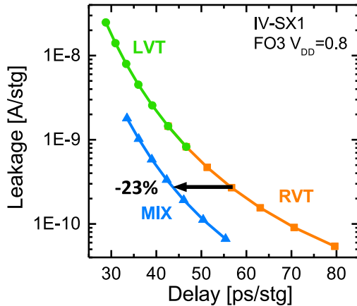
Figure C.18: Compromis fuite/délai simulé pour un inverseur à un doigt (IV-SX1) à V_{DD}=0.8V pour les différentes options de V_T . Une réduction du délai de 23% est prédite pour l'approche MIX par rapport à la référence RVT.
