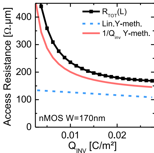
Figure C.2: Résistance d'accès en fonction de la charge d'inversion selon la méthodologie employée. Notre nouvelle méthode est en accord avec la méthode R_{TOT}(L) , sans faire l'hypothèse d'une mobilité constante.
