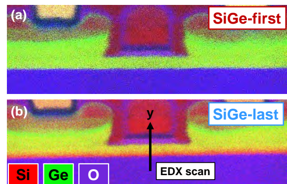
Figure C.23: Cartographie d'analyse dispersive en énergie (EDX) montrant un canal SiGe uniforme pour l'intégration "SiGe-first" et un bi-couche SiGe/Si pour le cas "SiGe-last".
