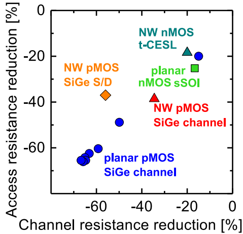
Figure C.5: Corrélation entre la variation de résistance d'accès par rapport à la variation de résistance de canal (c'est à dire mobilité) pour différents types de transistors et d'intégrations de contrainte. La résistance d'accès est impactée par la contrainte au même titre que la mobilité, avec une sensibilité similaire.
