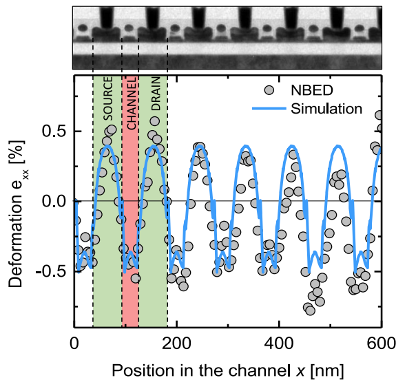
Figure C.10: Déformation relative par rapport au Silicium dans le SiGeOI en fin de procédé de fabrication. La simulation est en accord avec la mesure expérimentale par NBD. Les oscillations proviennent de l'alternance entre les canaux (sous la grille) et les régions de source/drain. Une déformation supplémentaire d'environ -0.4% est générée par les source/drain \text{Si}_{0.7}\text{Ge}_{0.3}\text{B} .
