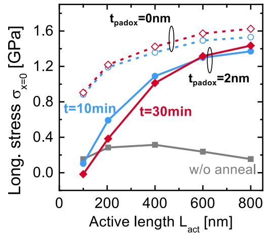
Figure C.35: Contrainte générée par BOX-creep en fonction de la longueur d'active. La diminution de la contrainte pour les courtes zones actives est fortement diminuée lorsqu'aucun oxyde pad n'est utilisé.
