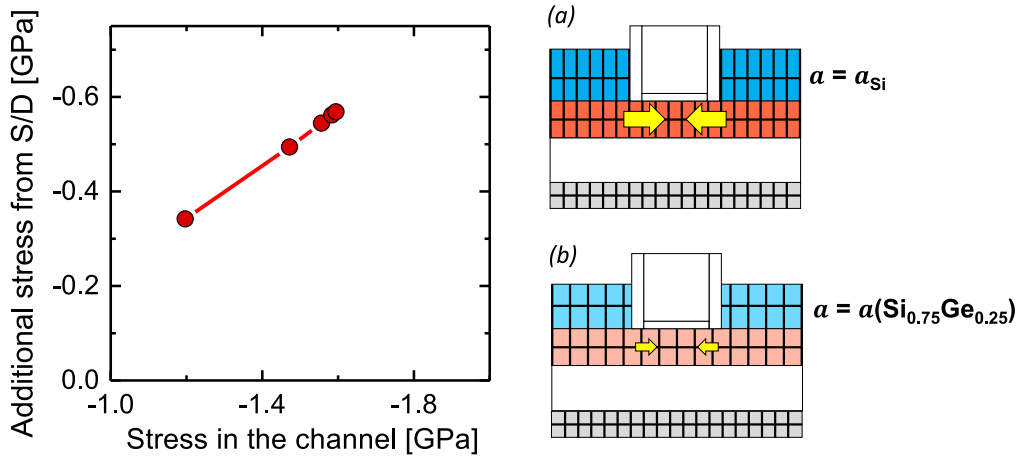
Figure C.11: Simulation de la contrainte additionnelle générée par les source/drain \text{Si}_{0.7}\text{Ge}_{0.3}:\text{B} en fonction de l'état de contrainte du substrat SiGeOI. A cause de la relaxation latérale du SiGeOI induite par la gravure, la croissance des source/drain est réalisée sur un substrat dont le paramètre de maille est plus large que celui du Silicium. En conséquence, la contrainte intrinsèque aux source/drain est plus faible et il est résulte une plus faible contrainte générée dans le canal.
