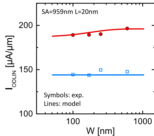
Figure C.31: Courant I_{ODLIN} en fonction de la largeur de zone active W pour des nFETs sSOI et SOI. La faible variation du courant I_{ODLIN} pour le substrat sSOI est due à la relaxation de la contrainte. La contrainte en tension transverse n'a que peu d'impact sur la mobilité des électrons.
