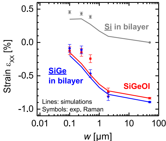
Figure C.9: Déformation \varepsilon_{XX} extraite par mesures \mu Raman dans des lignes de SiGe en fonction de leurs largeurs w . Deux cas sont étudiés: SiGeOI obtenu par condensation et un bi-couche SiGe/Si obtenu par épitaxie. Plus la ligne est étroite, plus la déformation est sensible à la relaxation latérale à partir des bords. La mesure \mu Raman permet également d'extraire la déformation en tension dans le Si du bi-couche SiGe/Si.
