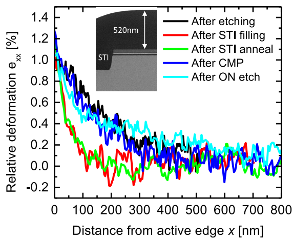
Figure C.7: Profil de déformation du SiGe relative au Silicium dans le plan ( e_{xx} ) mesurée par NBD en bord de zone active pour différentes étapes du procédé. La condition de bord libre introduite après gravure permet à la contrainte compressive du SiGe de se relaxer latéralement.
