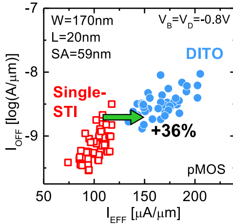
Figure C.28: Compromis I_{EFF}/I_{OFF} pour les pMOSFETs démontrant +36% de gain à même fuite avec une isolation duale (DITO) par rapport à la référence.
