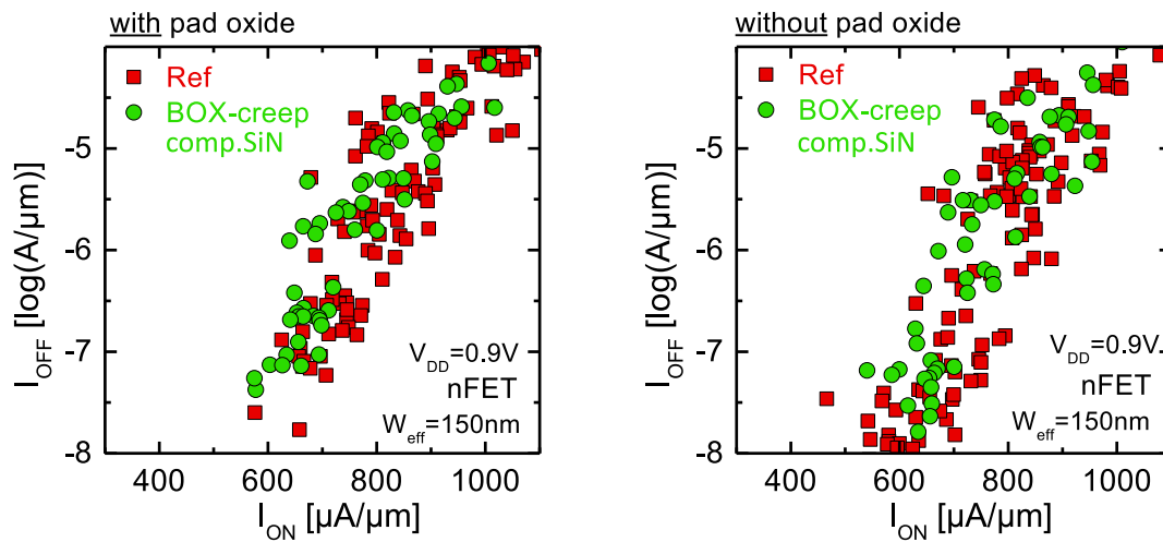
Figure C.36: Compromis I_{ON}/I_{OFF} de nFETs avec et sans BOX-creep que ce soit (gauche) avec ou (droite) sans oxyde pad. Le procédé de BOX-creep, qui utilise un SiN compressif obtenu par PECVD, n'a que très peu d'impact sur la performance. Ce résultat suggère qu'aucune contrainte tensile significative n'a été générée dans le SOI.
