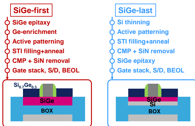
Figure C.22: Schémas d'intégration des procédés "SiGe-first" (référence avec condensation) et "SiGe-last", dans lequel le SiGe est fabriqué par épitaxie après le module de définition des zones actives.
