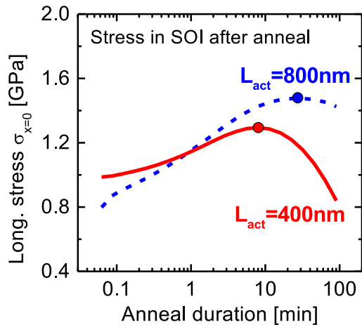
Figure C.34: Contrainte dans le SOI au cours du recuit pour deux longueurs d'active. Une durée optimale pour maximiser la contrainte est mise en évidence.
