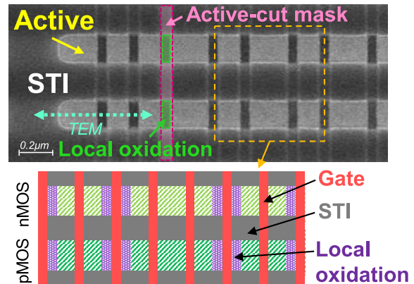
Figure C.26: Image MEB en vue du dessus prise après la définition des zones actives et dessin associé mettant en évidence l'isolation duale par tranchées et oxydation. L'isolation dans le sens longitudinal est réalisée par oxydation locale pour maintenir la contrainte compressive tandis que des tranchées classiques (STI) isolent les transistors dans la direction transverse.
