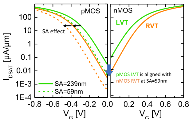
Figure C.16: Caractéristiques de transfert I_D(V_G) pour les deux options de V_T et pour deux longueurs de zone active. Pour SA=59nm, le nFET RVT est aligné au pFET LVT à cause de la relaxation de la contrainte augmentant le V_T du pFET.
