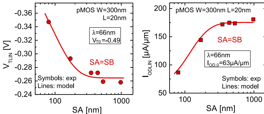
Figure C.13: (gauche) V_{TLIN} and (droite) I_{ODLIN} en fonction de la distance au bord de zone active SA (=SB) pour un pFET à canal SiGeOI ( W=300nm L=20nm ). La tension de seuil augmente et I_{ODLIN} diminue pour les zones actives courtes à cause de la relaxation de la contrainte longitudinale. Le modèle de relaxation nous permet de reproduire la variation des caractéristiques électriques.
