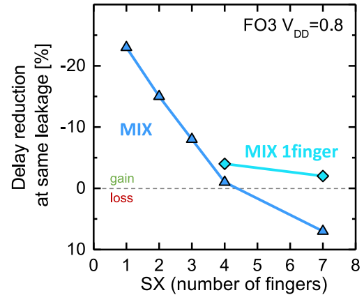
Figure C.19: Gain en délai pour une fuite donnée en fonction du nombre de doigts de grille de l'inverseur. Plus la zone active est longue, moins l'approche MIX est pertinente car la relaxation de la contrainte a lieu en bord de zone active. L'approche "MIX 1 finger" où seulement les premiers doigts de grille en partant du bord sont de type LVT au lieu de RVT permet d'améliorer le compromis pour les inverseurs à plus de 4 doigts de grille.
