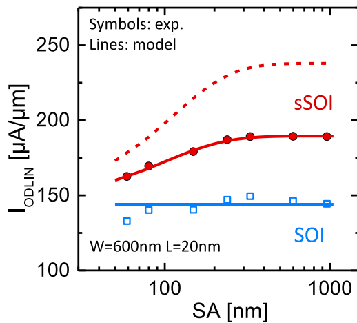
Figure C.30: Courant I_{ODLIN} en fonction de la distance grille-STI SA pour un nFET fabriqué sur substrat sSOI et comparé à la référence SOI. La dégradation du courant pour les petits SA est due à la relaxation longitudinale. Le modèle surestime le gain (tirets). Afin de reproduire les mesures, une résistance d'accès R_{ACC}=132\Omega\cdot\mu\text{m} doit être considérée. La longueur typique de relaxation est \lambda=86\text{nm} .
