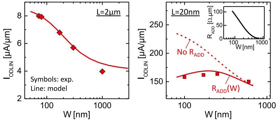
Figure C.14: I_{ODLIN} vs. largeur d'active W pour un canal (gauche) long L=2\mu\text{m} et (droite) court L=20\text{nm} . La relaxation de la contrainte transverse pour les zones actives étroite se traduit par un gain en mobilité. Alors que le modèle permet de bien reproduire l'effet layout pour un canal long, ce n'est pas le cas pour un canal court. Une hypothèse de résistance d'accès plus prononcée pour les zones actives étroites est avancée. Cette résistance d'accès pourrait provenir de l'épitaxie des source/drain avec facettes (faible vitesse de croissance des plans 111).
