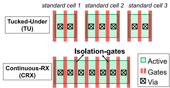
Figure C.20: Illustration des approches de dessin conventionnel ("Tucked-Under") et de type "Continuous-RX" (CRX). Le CRX consiste à dessiner les cellules sur une même bande de zone active et de les isoler à l'aide de grilles d'isolations. De ce fait, la zone active n'est pas gravée dans le sens longitudinal et la contrainte compressive est maintenue dans cette direction.
