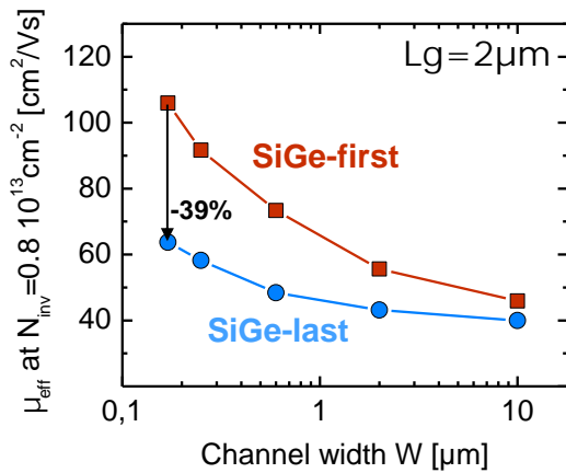
Figure C.24: Mobilité des trous extraite par split-CV sur canal long en fonction de la largeur du transistor pour les deux schémas d'intégration. L'amélioration due à la relaxation de la composante transverse de la contrainte est moins prononcée pour "SiGe-last".
