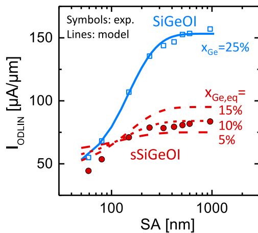
Figure C.32: Courant I_{ODLIN} en fonction de la distance grille-STI SA pour les pFETs à canal SiGe fabriqués sur substrat sSOI (sSiGeOI) et comparé à la référence SiGeOI. Le niveau de contrainte compressive dans le canal sSiGeOI est fortement réduit à cause de la tension du sSOI. Le modèle, calibré sur les données SiGeOI, permet de reproduire les données expérimentales en assumant une contrainte compressive équivalente à une concentration x_{Ge,eq}=10\% après condensation. La longueur typique de relaxation est \lambda=82\text{nm} .
