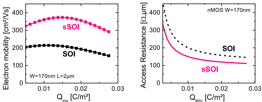
Figure C.4: Extraction de (gauche) la mobilité des électrons pour un canal long ( L=2\mu\text{m} ) et (droite) la résistance d'accès selon notre nouvelle méthodologie pour des nFETs fabriqués sur SOI et sSOI. La contrainte en tension améliore la mobilité mais également diminue la résistance d'accès des dispositifs.
