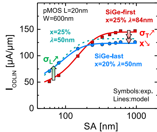
Figure C.25: Courant de drain I_{\text{ODLIN}} (mesuré à V_G=V_T+0.5 ) en fonction de SA (distance du transistor au bord de zone active dans le sens longitudinal). La réduction de I_{\text{ODLIN}} pour les petits SA est due à la relaxation de la contrainte, dégradation la mobilité des trous. L'approche "SiGe-last" est moins sensible, suggérant une plus faible longueur typique de relaxation latérale.
