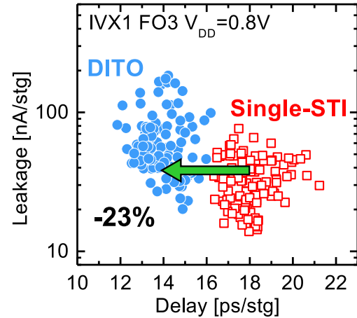
Figure C.29: Compromis fuite/délai ( I_{DDQ}/\tau_P ) d'oscillateurs en anneaux d'inverseurs à un doigt de grille. L'intégration avec isolation duale permet de réduire le délai de 23% par rapport à l'intégration de référence avec STI.
