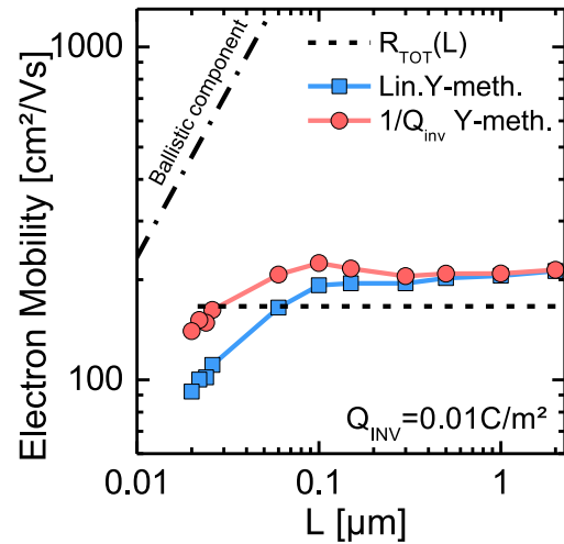
Figure C.3: Mobilité en fonction de la longueur de grille selon la méthodologie d'extraction employée. La chute de mobilité pour les transistors courts donnée par la Fonction-Y classique est atténuée pour notre méthodologie.
