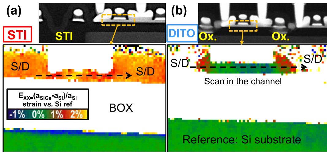
Figure C.27: Cartographie de la déformation par rapport à la référence Si, mesurée par diffraction d'électrons PED (Precession Electron Diffraction) pour un dispositif (a) proche d'une tranchée (STI) et (b) entre deux oxydations locales.
