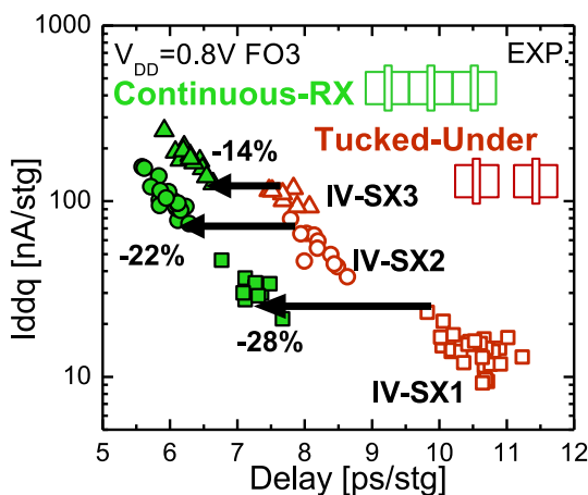
Figure C.21: Compromis Fuite/Délai pour des oscillateurs en anneau d'inverseurs à 1, 2 ou 3 doigts de grille selon la configuration CRX ou "Tucked-Under" (résultats expérimentaux). L'approche CRX permet de fortement réduire le délai (-28% pour l'IV-SX1) en optimisant l'état de contrainte. L'augmentation de la fuite est due au plus faible V_T des pFETs ainsi qu'aux grilles d'isolations (transistors parasites).
