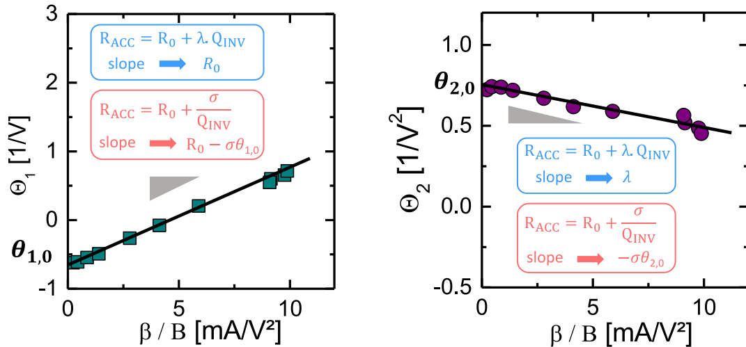
Figure C.1: (gauche) \Theta_1 et (droite) \Theta_2 vs. \beta (ou B ). Les paramètres de mobilité et de résistance d'accès sont extraits à partir de régressions linéaires, selon le modèle de dépendance en charge d'inversion considéré.
