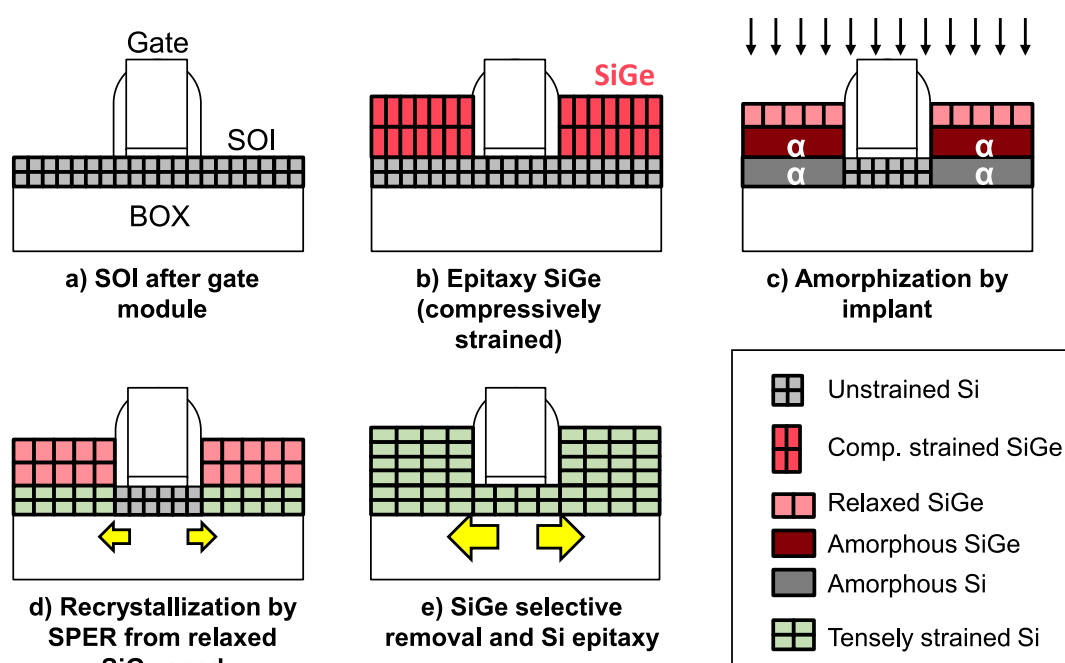
Figure C.37: Procédé de fabrication de la technique "SDRASS". a) dispositif SOI après formation de la grille et des espaceurs. b) Epitaxie de SiGe pseudomorphe dans la région des source/drain (30% Ge). c) Amorphisation par implantation Si ( 2.5 \cdot 10^{14} \text{ cm}^{-2} à 40keV sans tilt). Un germe de SiGe cristallin doit être maintenu à la surface. d) Recristallisation par épitaxie en phase solide (SPER). Le SOI recroît selon le paramètre de maille du germe SiGe. Une contrainte en tension est générée si le germe SiGe est relaxé. e) Retrait sélectif du SiGe et épitaxie des source/drain surelevés en Si. Cette dernière étape permet d'avoir un volume plus important de Si en tensions dans les source/drain et donc de favoriser la génération de contrainte dans le canal voisin.
