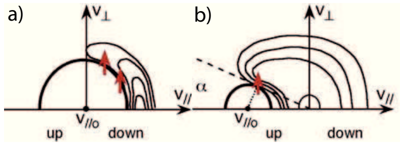
Figure 2.7 – (a) Distribution d'électrons de type coquille. Le gradient positif \nabla v_{\perp} de la fonction de distribution est situé le long du bord extérieur de la distribution. Le cercle de résonance de l'IMC menant à une amplification est tangent à celui-ci et est centré sur v_{\parallel 0} = 0 ; (b) Distribution d'électrons de type cône de perte. Le cône de perte est la région appauvrie en électrons, perdus par collision avec l'atmosphère. Cette région est située sous la ligne en pointillés, définie par l'angle d'attaque \alpha . Le plus grand gradient positif \nabla v_{\perp} de la fonction de distribution (flèche rouge) est sur le bord du cône, à la vitesse de résonance v . Le cercle de résonance de l'IMC menant à une amplification maximale est tangent à ce gradient, et est centré sur v_{\parallel 0} = v_r / \cos \alpha – Figure tirée de Hess et al. (2008).
