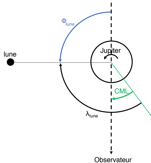
Figure 6.5 – Définition du CML de l'observateur (en vert), de la phase d'Io \Phi_{Io} (en bleu) et la longitude d'Io \lambda_{Io} (en noir) – Figure inspirée de Marques et al. (2017).
