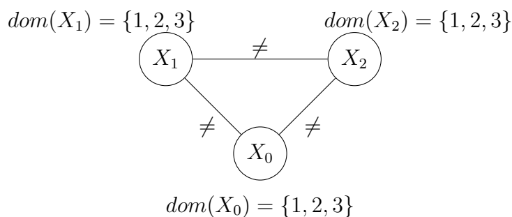
FIGURE 1.2 – Exemple d'un CSP
