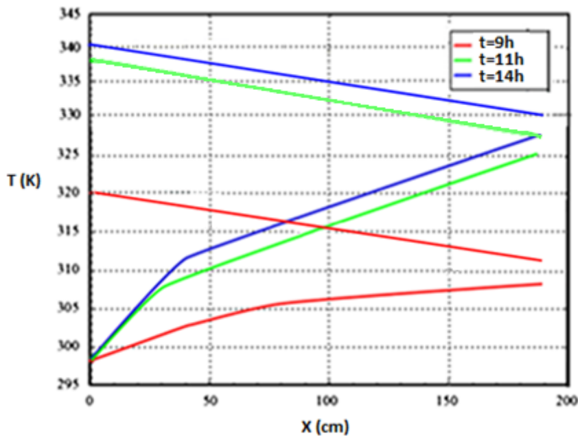
Figure 2.2 : Évolution de la température de l'air T_{fl} dans les phases aller et retour dans le capteur.
