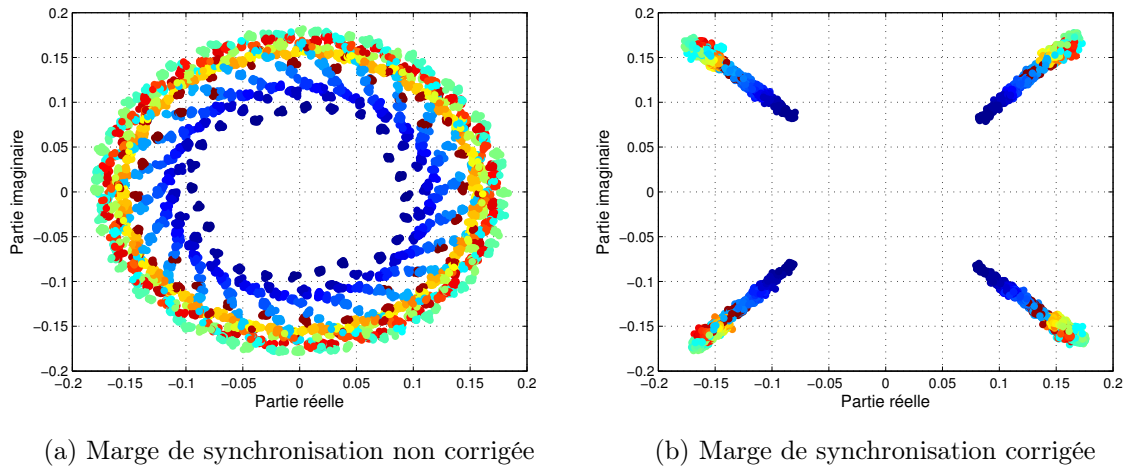
FIGURE 3.17 – Constellations des symboles de données reçus par l'utilisateur avant et après la correction de la marge de synchronisation
