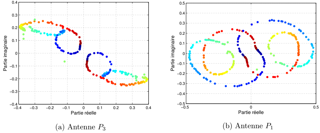
FIGURE 3.15 – Constellations d'un symbole OFDM pilote reçu par deux antennes du point d'accès lors de la phase d'estimation dans une configuration NLOS
