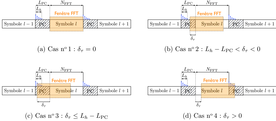
FIGURE 3.1 – Les quatre cas de synchronisation temporelle : seul les cas n° 1 et n° 2 permettent une synchronisation correcte
