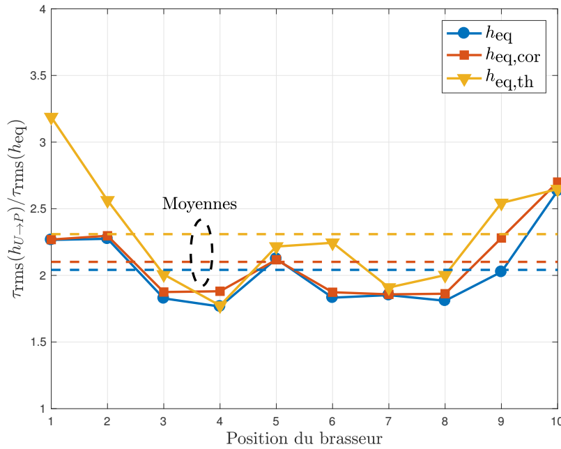
FIGURE 5.32 – Facteur de compression temporelle en fonction de la position du brasseur
