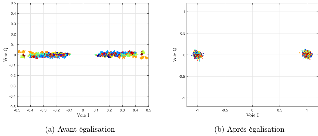
FIGURE 5.11 – Constellations BPSK reçues
