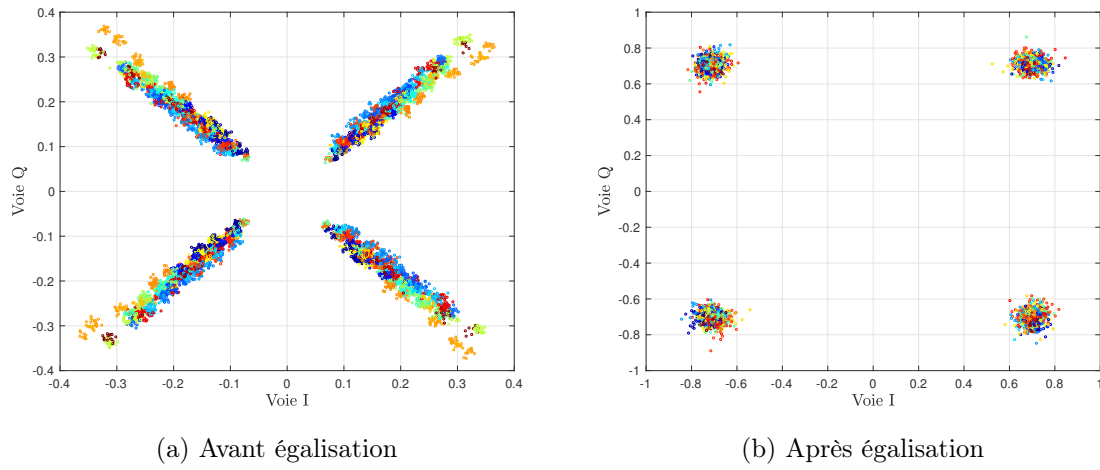
FIGURE 5.12 – Constellations QPSK reçues
