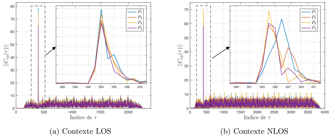
FIGURE 3.14 – Module de la fonction d'intercorrélation de la détection du début de trame de la phase d'estimation
