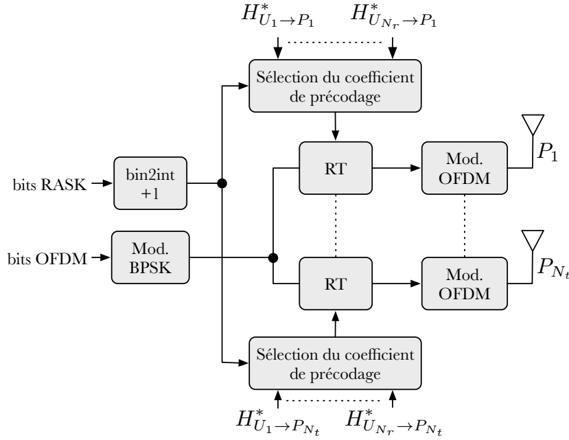
FIGURE 6.3 – Schéma du modulateur RASK-OFDM
