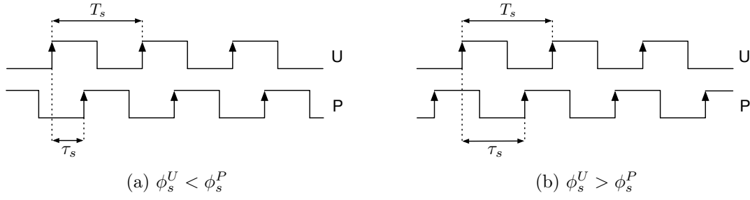
FIGURE 4.12 – Décalage temporel, dû à la présence de SPO, entre l’horloge du CNA de l’utilisateur et celle du CAN du point d’accès
