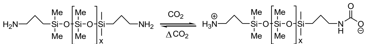
Figure 2 : Réaction entre une amino-silicone et le CO 2 [54]
