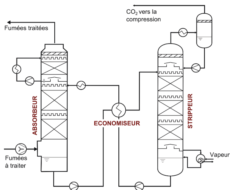
Figure 1: Procédé de captage de CO 2 en post combustion par absorption chimique (d'après document interne EDF R&D)
