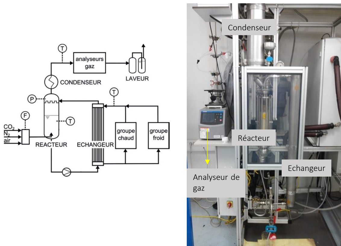
Figure 11 : Représentation schématique et photo du banc d'essai LEMEDES-CO 2 [90] (T : sonde de température ; P : sonde de pression ; F : débitmètre)
