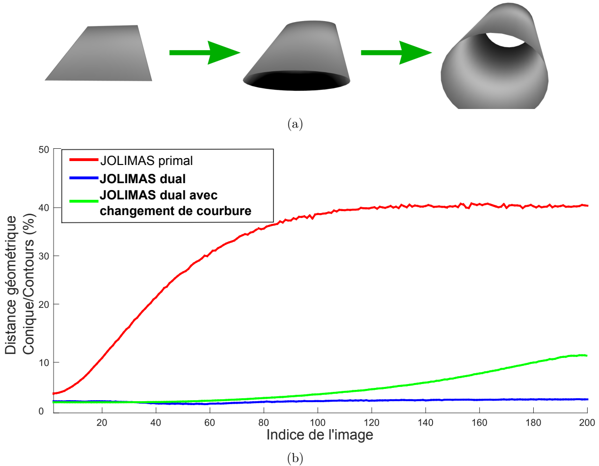
FIGURE 5.6 – Comparaison entre JOLIMAS primal et notre modèle JOLIMAS dual. Dans cette séquence de synthèse, la courbure augmente progressivement à chaque image comme illustré dans (a). En utilisant 6 poses de caméra, les deux modèles primal et dual sont reconstruits et comparés en utilisant la distance 2D entre la prédiction de spécularité et les contours de la spécularité détectée. Notre approche duale réalise de meilleurs résultats que JOLIMAS primal avec une erreur moyenne de 1% par ellipse comparée à une erreur de 33% par ellipse en moyenne pour JOLIMAS primal. Nous testons également la prédiction de spécularité de notre modèle dual en reconstruisant une quadrique sur une surface plane (première image) et en l'utilisant pour les changements de courbure restants. Même si l'erreur croît pour chaque image, la prédiction de spécularité reste fiable avec une erreur relativement faible (7% en moyenne).
