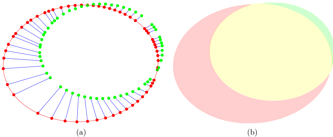
FIGURE B.3 – Dans (a) le distance point/point est représenté comme étant la somme des distances Euclidiennes entre les contours de spécularités (en vert) et l'ellipse discrétisée par notre méthode (points rouges). Dans (b), nous illustrons la distance de Jaccard en utilisant l'intersection (en jaune) de l'aire des deux ellipses (en rouge et vert). L'union correspond à la somme de ces 3 couleurs.
