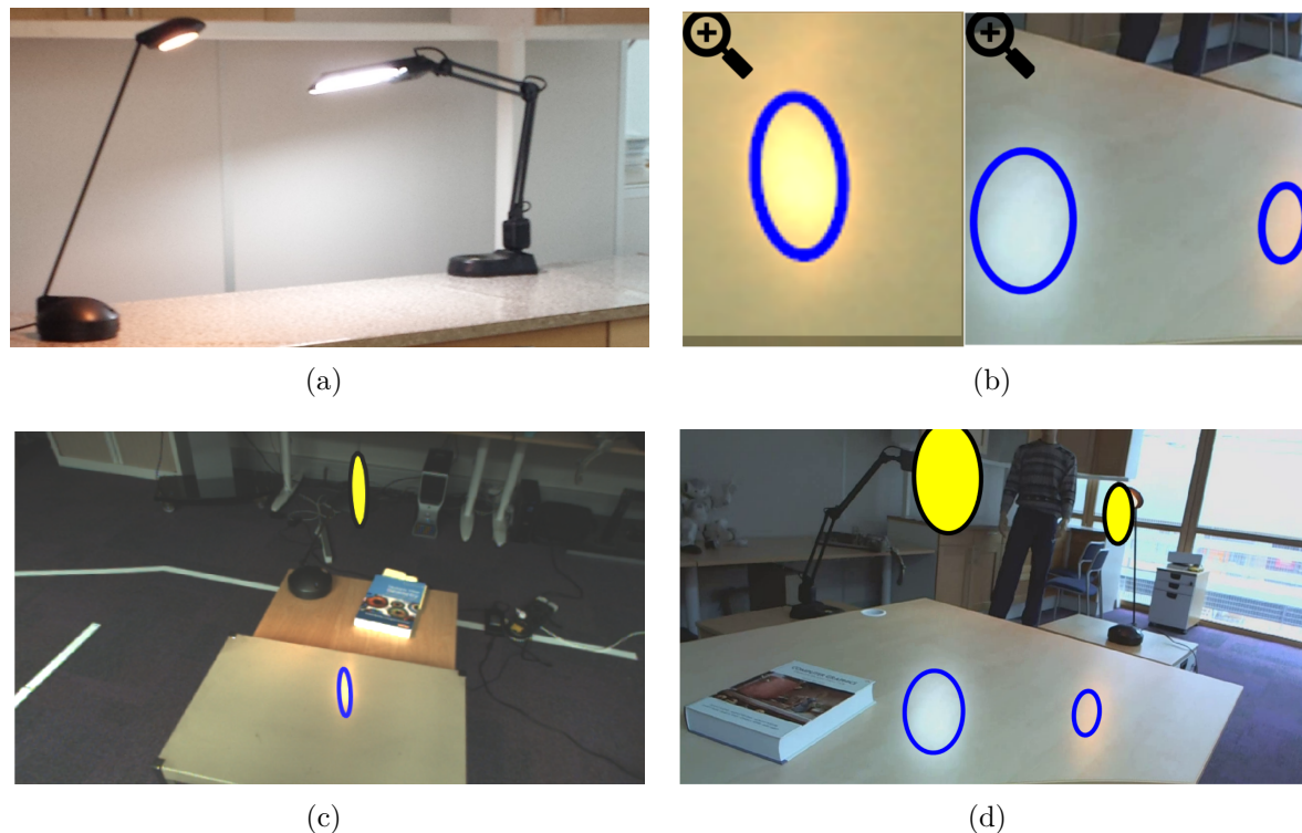
FIGURE 4.5 – Nous observons qu’une spécularité présente une forme elliptique. Nous la prédisons en projetant une quadrique virtuelle fixe incluant les propriétés de lumière et de matériau. Cette figure présente des exemples de reconstruction de quadrique (ellipsoïde jaune) pour deux types de lumière (ampoule (c) et néon (d)) et de matériaux (table en fer (c) et plan de travail d’une cuisine (d)). Une fois notre modèle reconstruit, nous l’utilisons pour prédire les spécularités pour des points de vue inconnus en la projetant sous forme d’ellipse (en bleu). (b) illustre un gros plan de la prédiction dans les séquences respectives.
