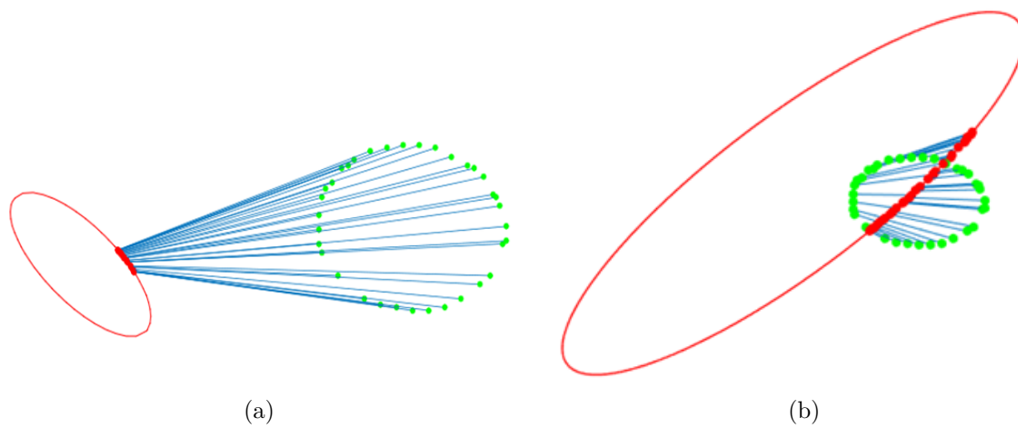
FIGURE B.5 – Limitation de la paramétrisation classique d'ellipse à partir de points de contours. Dans (a), nous illustrons le problème de la paramétrisation pour des contours éloignés considérablement de l'ellipse associée. Notre paramétrisation recherche les points de l'ellipse les plus proches des points de contours ce qui provoque une mauvaise répartition des points sur l'ellipse. Dans (b), nous illustrons le problème d'une paramétrisation entre des points contours répartis sur une surface beaucoup plus importante que l'ellipse associée. Ces deux problèmes ont pour impact d'avoir une distance ellipse/point trop faible et incohérent.
