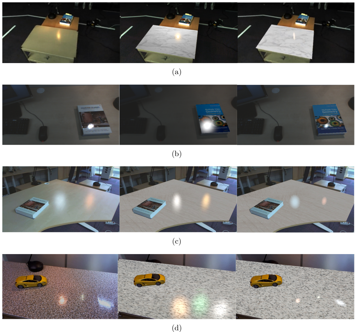
FIGURE 7.4 – Comparaison des méthodes de retexturing de notre implémentation de Buteau et Saito (2015) (milieu) et de notre approche (droite). La méthode de Buteau et Saito (2015) étant une méthode pour reconstruction des sources de lumière ponctuelles, nous avons manuellement ajouté la rugosité, la couleur et l'intensité de la source de lumière en utilisant le modèle d'illumination locale de Phong. Nous utilisons uniquement le terme spéculaire. Le retexturing est illustré sur la séquence ampoule/table de fer (a) en utilisant une texture de marbre, (b) la séquence ampoule/libre en changeant la couverture du livre par une autre, (c) la séquence néon/ampoule/table en bois en changeant la texture de bois d'une table en une autre et (d) la séquence multi-lumière/comptoir de cuisine en utilisant une texture de roche. Sans prendre en compte le terme diffus sur la texture, la texture de la surface peut être changée de façon réaliste en utilisant uniquement le terme spéculaire prédit par JOLIMAS. Contrairement à l'approche de Buteau et Saito (2015) , nous calculons de façon précise la forme, la position et l'intensité de la spécularité avec un temps d'exécution faible pour un résultat réaliste. De plus, calculer l'illumination à partir de modèles comme celui de Phong ne peut pas être fait sans données sur les matériaux et le nombre de sources lumineuses.
