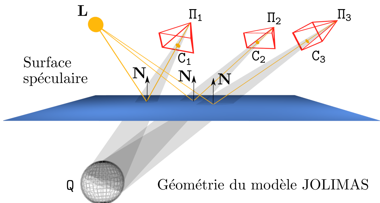
FIGURE 4.1 – Lien entre le modèle physique (lumière et matériaux) et la géométrie multi-vues (notre modèle empirique). À partir de plusieurs points de vue, une quadrique est reconstruite à partir de spécularités de forme elliptique. Cette quadrique virtuelle projetée sur chaque point de vue correspond aux spécularités.
