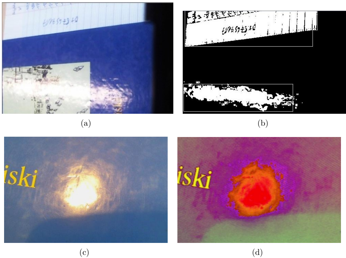
FIGURE A.4 – Dans l'image (a), le papier a un aspect semblable à une spécularité et pourrait être détecté à tort comme étant une spécularité. (b) montre l'étape de séparation des candidats spéculaires de la figure (a). (c) représente une spécularité vue dans l'espace RVB. (d) illustre la décroissance progressive de l'intensité d'une spécularité à partir de son centre dans l'espace TSV.
