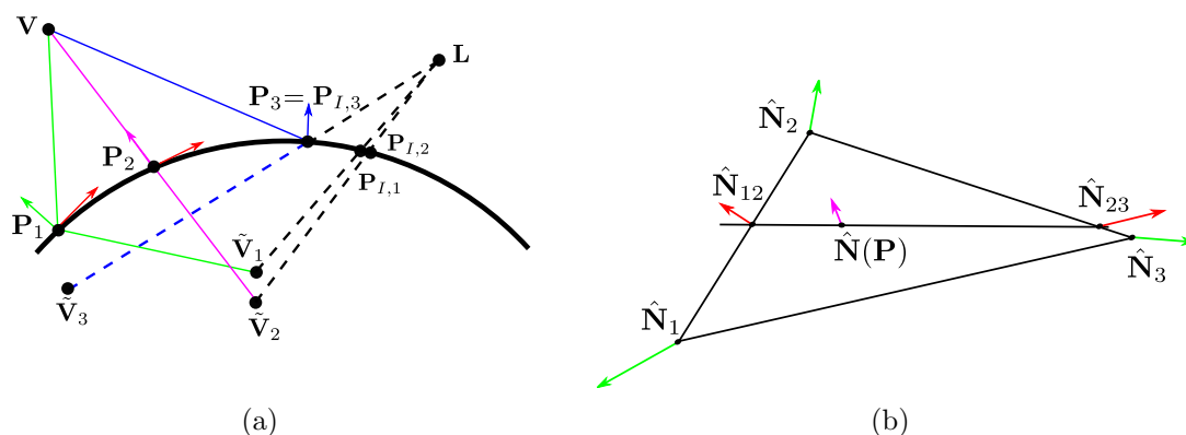
FIGURE 5.4 – Calcul du point le plus intense et interpolation de normale. Dans (a), notre algorithme pour calculer le point le plus intense est illustré. À partir d’une initialisation \mathbf{P}_1 , nous calculons la position de la caméra virtuelle \tilde{\mathbf{V}}_1 (symétrique de \mathbf{V} ) par rapport au plan tangent à la surface en \mathbf{P}_1 et la ligne contenant \tilde{\mathbf{V}}_1 et \mathbf{L} . Puisque l’intersection \mathbf{P}_{I,1} entre la ligne et la surface S n’est pas égale à \mathbf{P}_1 , nous itérons à la face adjacente dans la direction du point d’intersection. Ce procédé s’arrête quand la distance entre \mathbf{P} et \mathbf{P}_I est minimale. Pour améliorer l’estimation sur la face restante, nous calculons une normale plus précise en utilisant une interpolation de normale dans (b). Dans cet exemple, à partir d’un polygone comportant trois sommets avec normales associées, la normale \hat{\mathbf{N}}(\mathbf{P}) en \mathbf{P} est calculée en interpolant les normales sur la ligne horizontale contenant \mathbf{P} avec les arêtes du polygone donnant \hat{\mathbf{N}}_{12} et \hat{\mathbf{N}}_{23} . À partir d’une interpolation linéaire de ces deux normales, \hat{\mathbf{N}}(\mathbf{P}) est calculé.
