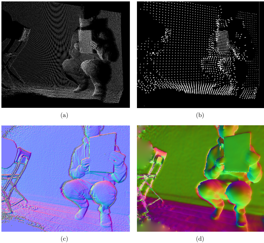
FIGURE 6.10 – Calcul de la carte de normale. À partir du nuage de points de la carte de profondeur (a), nous utilisons la bibliothèque PCL afin de calculer les normales à partir des points 3D voisins (b). Dans (c), nous illustrons une approche naïve du calcul de la carte de normale à partir de l’image de profondeur (2D) directement au lieu d’utiliser le nuage de points (3D). Nous constatons un bruit assez important sur des surfaces qui sont censées être planes (mur et livre). La carte de normale (d) obtenue à partir de la PCL est suffisamment précise pour notre application.
