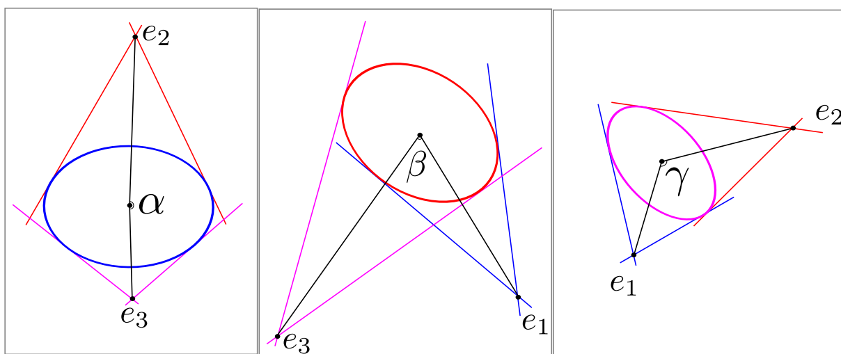
FIGURE B.9 – Critère utilisant la répartition des tangentes épipolaires afin de sélectionner les images clés. L'objectif est de maximiser l'angle entre chaque droite contenant le centre de l'ellipse et chaque épipôle à partir de trois images.
