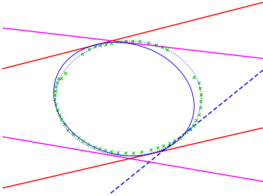
FIGURE B.2 – Correction épipolaire de Reyes et Bayro-Corrochano (2005). L'ellipse observée (points bleus) est calculée à partir des points de contour (croix noires) de la spécularité. Les quatre droites épipolaires créées à partir des autres points de vue sont représentées en rouge et magenta. Afin d'estimer la conique duale respectant la géométrie épipolaire, une cinquième droite calculée à partir de la tangente d'un point de contours (droite en pointillée en bleu). Nous calculons une ellipse dans l'espace dual pour chaque point de contour et nous choisissons celle (représentée ici) minimisant la distance ellipse/point évoquée à section B.3.2.2 pour chacun des trois points de vue. Les ellipses obtenues seront utilisées dans le processus de reconstruction d'une quadrique précise à partir d'ellipses épipolairement consistantes.
