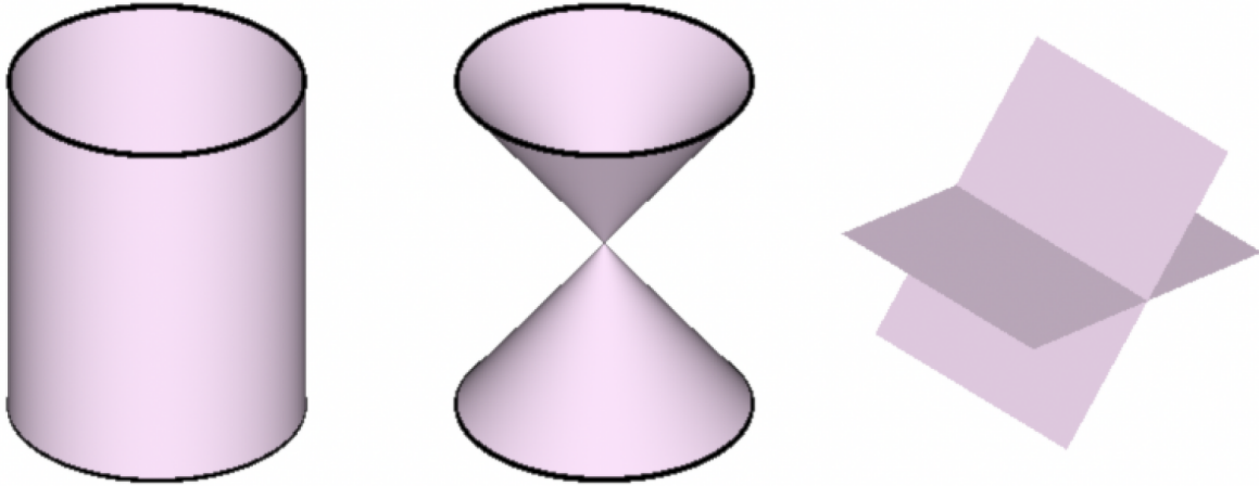
FIGURE 2.5 – Exemples de quadriques dégénérées. De gauche à droite nous avons un cylindre, un cône et une paire de plans (de rang 2). Les illustrations sont extraites de Cross (2000) .
