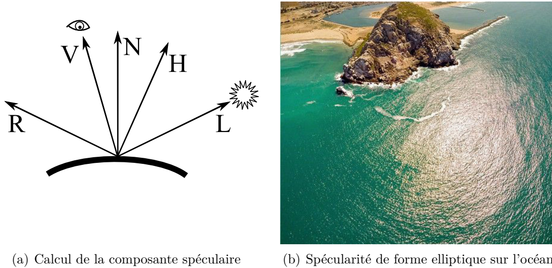
FIGURE 2.15 – Calcul de la composante spéculaire en utilisant le rayon réfléchi \mathbf{R} dans le modèle de Phong ou \mathbf{H} le vecteur mi-chemin entre \mathbf{V} et \mathbf{L} (a) et (b) spécularité visible sur l'océan de forme elliptique.
