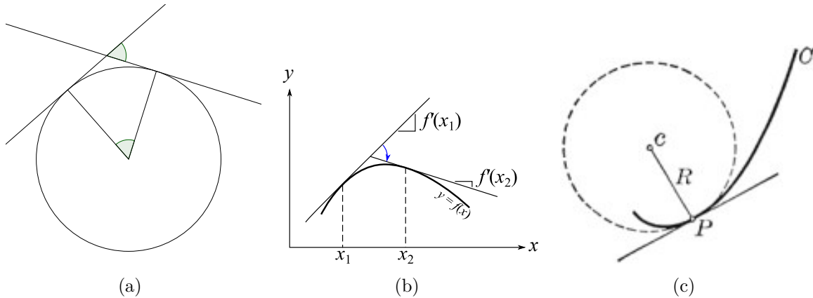
FIGURE 2.9 – Dans (a), nous montrons que l'angle entre les deux tangentes est égal à l'angle au centre. Dans (b), nous montrons que plus un arc est courbé, plus la pente de la tangente varie vite. Dans (c), un exemple de courbure est illustré. Au point \mathbf{P} , le rayon de courbure de la courbe C est égal à R .
