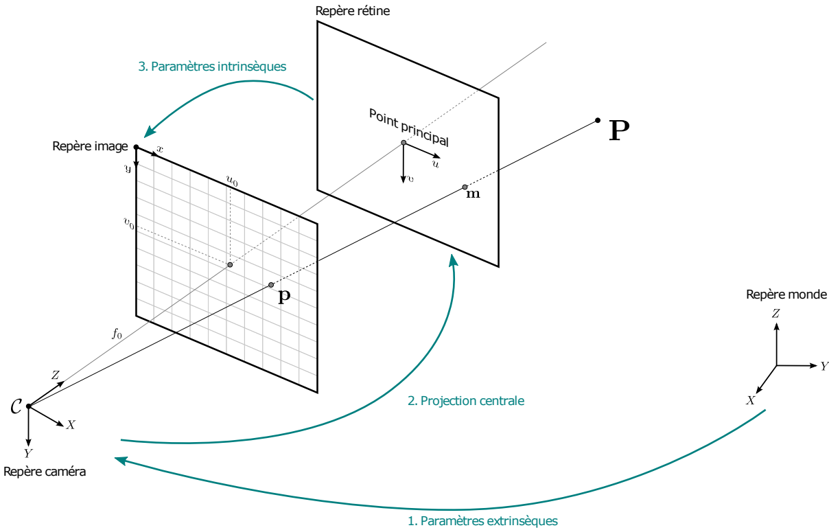
FIGURE 2.1 – Projection perspective. La projection perspective peut être vue comme trois transformations géométriques consécutives pour les points 3D.
