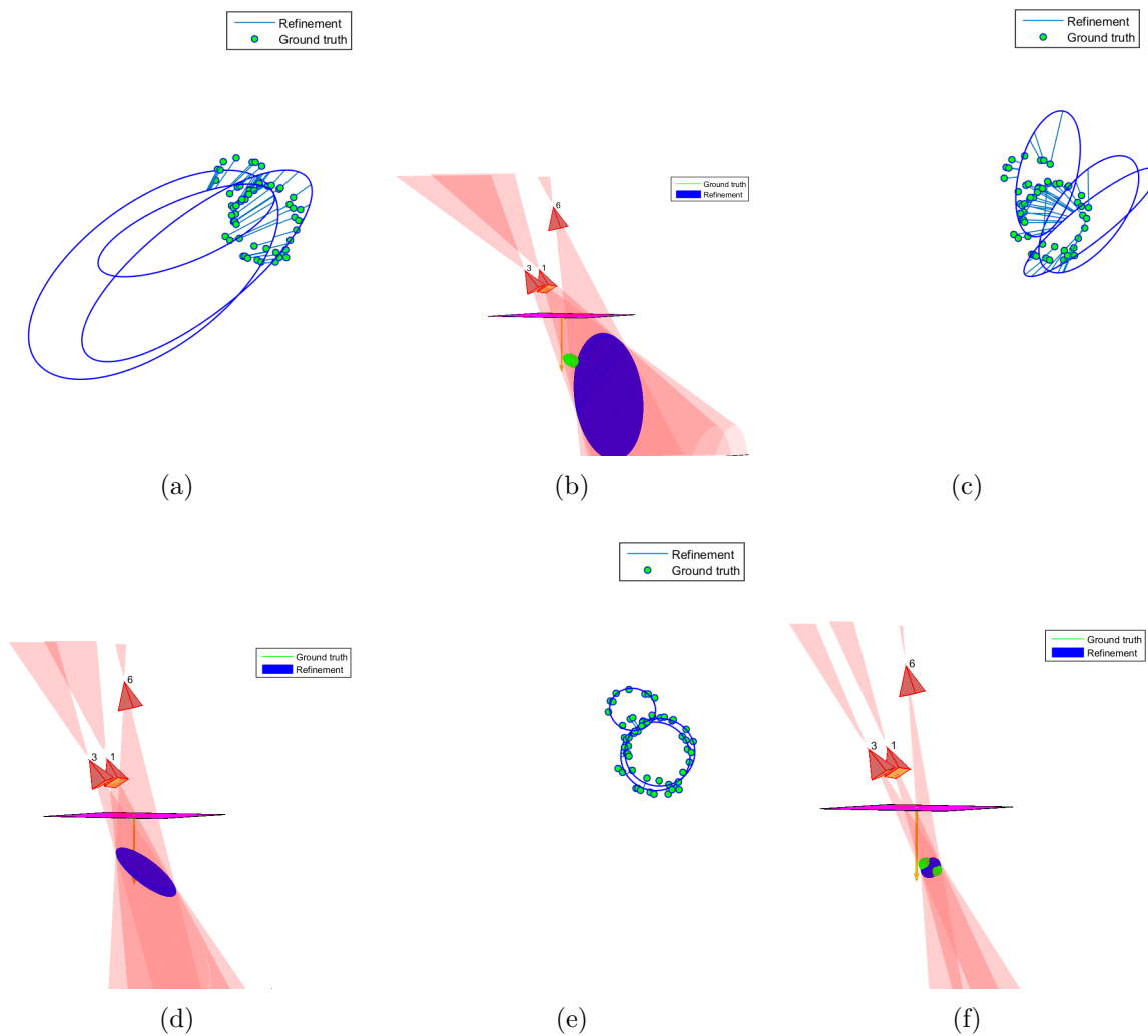
FIGURE B.8 – Illustration de l'évolution du raffinement non-linéaire de quadrique (à droite) à partir des contours de spécularité en vert. Nous pouvons observer l'évolution des ellipses correspondant aux projections de la quadrique en fonction des poses de caméra.
