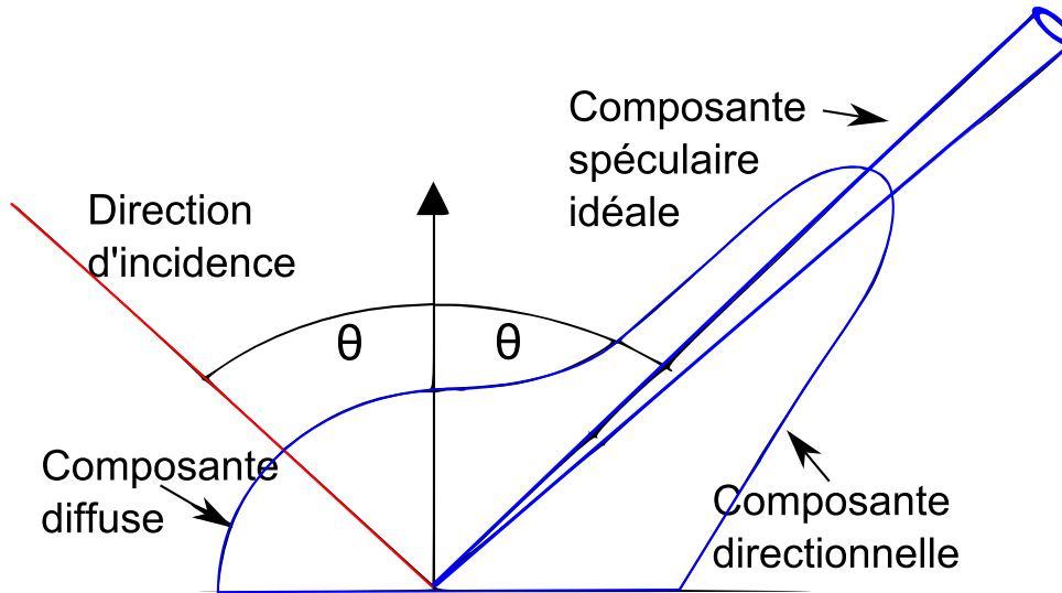
FIGURE A.5 – Représentation de la répartition lumineuse provoquée par la réflexion d'un rayon incident avec un objet. Cette répartition est déterminée en utilisant la BRDF du matériau. Nous constatons également que l'intensité de la lumière pour une réflexion spéculaire décroît progressivement autour du centre de gravité de la spécularité (composante spéculaire idéale).
