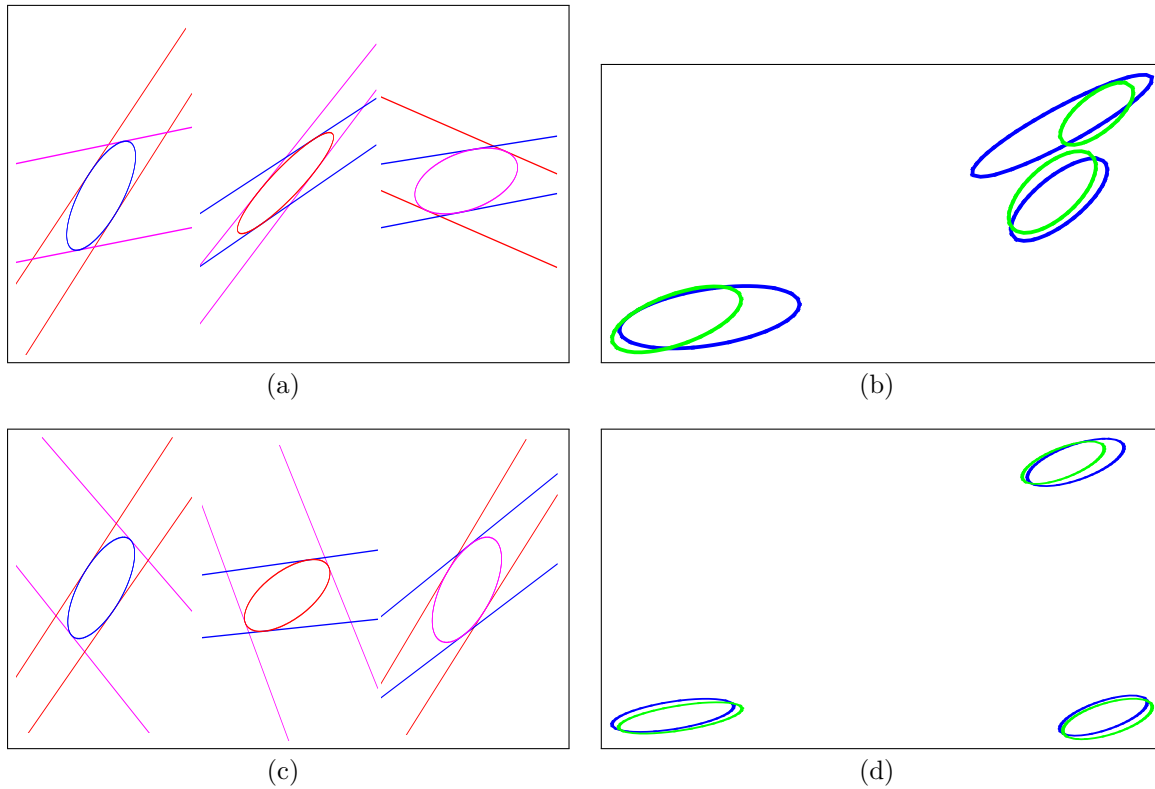
FIGURE B.10 – Comparaison de la qualité de reconstruction de quadrique pour des images choisies manuellement (première ligne) et par notre sélection d'images clés (deuxième ligne). Dans (a, c), nous illustrons les trois ellipses (bleu, rouge et magenta) utilisées pour la reconstruction ainsi que les contraintes épipolaires associées à chacune des ellipses provenant des deux autres points de vue. Nous pouvons observer que dans le cas des images clés, les contraintes épipolaires sont beaucoup plus réparties par rapport aux images sélectionnées manuellement ce qui permet d'améliorer le processus de reconstruction de la quadrique. Les ellipses issues de la projection de la quadrique (en bleu) pour les points de vue issus des images sélectionnées manuellement (b) et des images clé (d) sont comparées avec leurs vérités terrain. Dans le cas des images clé, nous pouvons observer que les ellipses projetées correspondent de manière presque identique à la vérité terrain.
