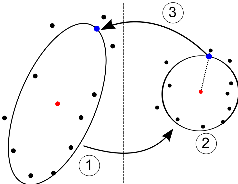
FIGURE B.4 – Paramétrisation d’ellipse. À partir de l’état initial (gauche) avec les contours de la specularité (points noirs), nous associons à chaque point de contours un point sur l’ellipse. Ces points de l’ellipse sont calculés en transformant l’ellipse (en cercle unitaire (droite)) et les points de contours par l’homographie H^{-1} (étape (1)). Dans l’étape (2), nous calculons les intersections des lignes passant par les points de contours et le centre du cercle unitaire avec ce même cercle. dans l’étape (3), les intersections (points bleus) sont transformées à nouveau sur l’ellipse avec l’homographie H .
