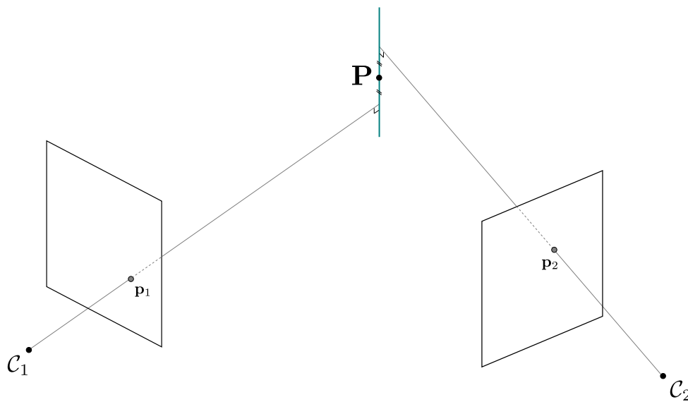
FIGURE 2.8 – Triangulation de points 3D. La structure de l'environnement peut être obtenue par triangulation des observations dans les images.
