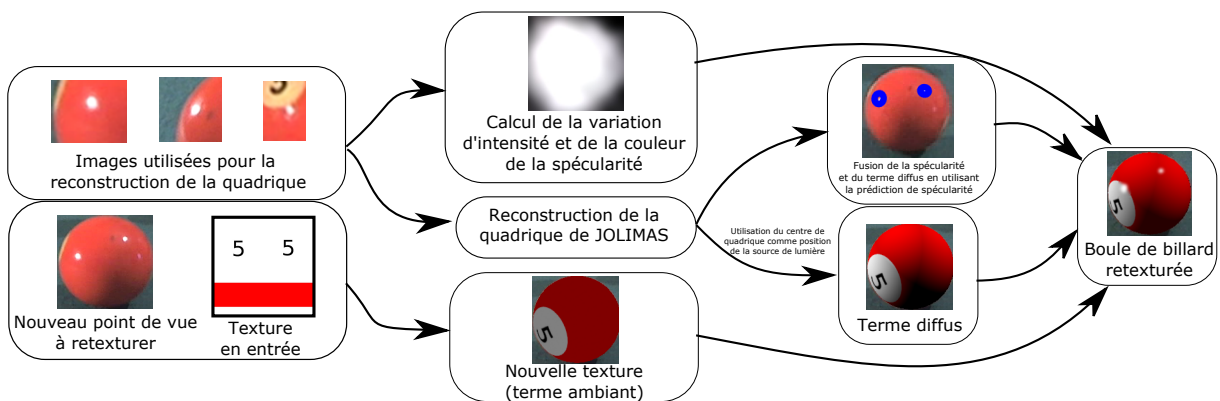
FIGURE 7.5 – Pipeline du processus de retexturing généralisé. La méthode est divisée en trois phases : la reconstruction de spécularité à partir des images utilisées pour la reconstruction de la quadrique 3D (partie du haut), calcul du terme diffus (partie du bas) et fusion de la spécularité synthétisée, la spécularité prédite et le terme diffus. La spécularité est reconstruite en termes de variation d'intensité et de couleur de façon empirique à partir des coniques prédites et des spécularités détectées dans les images. Afin de calculer le terme diffus, nous considérons le centre des quadriques reconstruites comme étant des sources ponctuelles. Nous calculons ensuite le terme diffus de Phong (1975). La spécularité et le terme diffus sont ensuite fusionnés afin de créer la nouvelle texture associée à la surface. L'ajout du terme diffus combiné aux spécularités améliore drastiquement le rendu.
