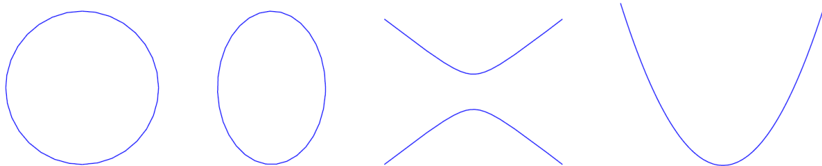
FIGURE 2.3 – Exemple de coniques. De gauche à droite, nous avons un cercle, une ellipse, une hyperbole et une parabole
