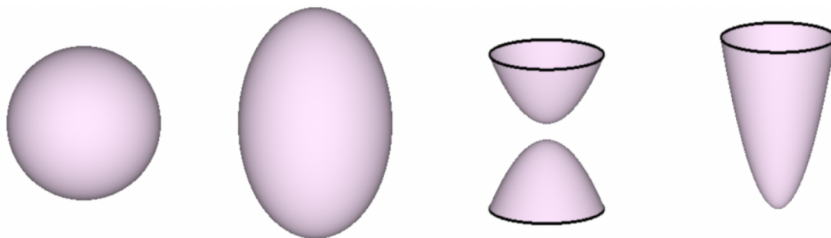
FIGURE 2.4 – Exemples de quadriques non-dégénérées. De gauche à droite, nous avons une sphère, une ellipsoïde, une hyperboloïde et une paraboloides. Les illustrations sont extraites de Cross (2000).
