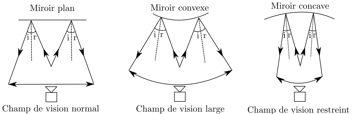
FIGURE 6.2 – Relation entre courbure et champ de vision dans le cas d’un miroir plan, convexe et concave (de gauche à droite). Nous observons que le champ de vision augmente lorsque le miroir devient convexe et diminue lorsque le miroir devient concave.
