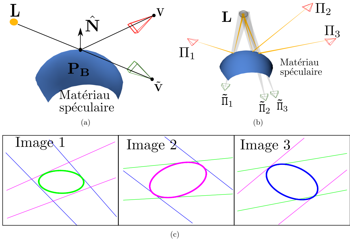
FIGURE 5.2 – JOLIMAS dual utilise des caméras virtuelles produisant des ellipses épipolairement consistantes. Dans (a), nous montrons la loi de la réflexion sur une surface convexe. Le point le plus intense \mathbf{P}_B correspond au point de la surface où l'intersection de la ligne contenant la position de la caméra virtuelle \tilde{\mathbf{V}} (en vert) et la source de lumière \mathbf{L} est confondue avec le point de la surface utilisé pour calculer la caméra virtuelle. Dans (b), nous présentons JOLIMAS dual sur une surface convexe pour 3 poses de caméra données \Pi_1, \Pi_2 et \Pi_3 . Les poses de caméra (en vert) \tilde{\Pi}_1, \tilde{\Pi}_2 et \tilde{\Pi}_3 permettent de reconstruire une quadrique proche de la source de lumière réelle \mathbf{L} . Dans (c), nous montrons que notre représentation virtuelle de caméra permet d'obtenir des ellipses respectant la géométrie épipolaire.
