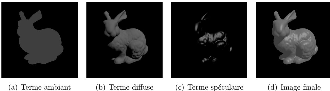
FIGURE 2.14 – Modèle de Phong produisant l'image (d) par la somme de 3 composantes : ambiante (a), diffuse (b) et spéculaire (c).
