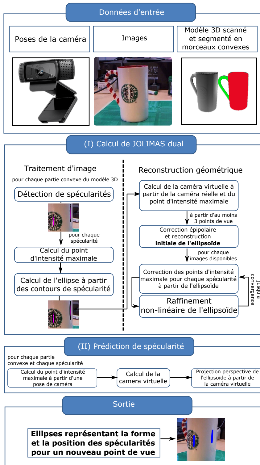
FIGURE 5.3 – Pipeline de notre méthode décrivant les données d'entrée, le calcul de notre modèle dual JOLIMAS et le processus de prédiction de spécularité. Notre méthode produit une ellipse décrivant la forme et la position de la spécularité dans l'image. Cette représentation géométrique abstrait l'interaction de la source de lumière (intensité, position, forme, couleur) avec le matériau (réflectance et rugosité) de la surface.
