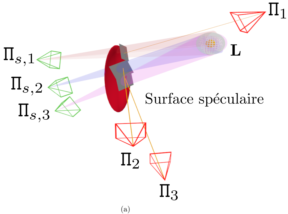
FIGURE 6.4 – Illustration de notre modèle canonique JOLIMAS. Pour chaque pose de caméra réelle ( \Pi_1 , \Pi_2 et \Pi_3 ), nous créons des poses de caméra virtuelles ( \Pi_{s,1} , \Pi_{s,2} et \Pi_{s,3} ) calculées à partir des points d'intensité maximale de chaque spécularité. En synthétisant la forme des spécularités sur le plan tangent aux points d'intensité maximale, nous sommes capables de reconstruire une quadrique localisée près de la source de lumière \mathbf{L} invariante à la courbure de la surface.
