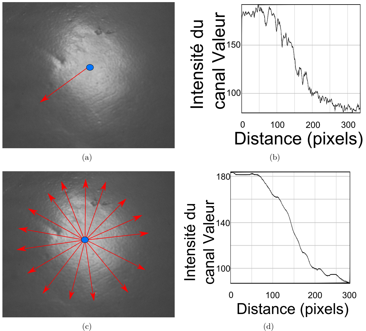
FIGURE A.6 – Analyse de la variation d'intensité du canal Valeur suivant. (a) représente un contour allant du centre de gravité et passant par un des contours de la spécularité. On observe une forme de sigmoïde très bruitée au niveau de son intensité dans (b). (c) représente un ensemble de contours sur le même principe que (a). La moyenne de l'intensité de ces contours nous donne un sigmoïde beaucoup plus exploitable.
