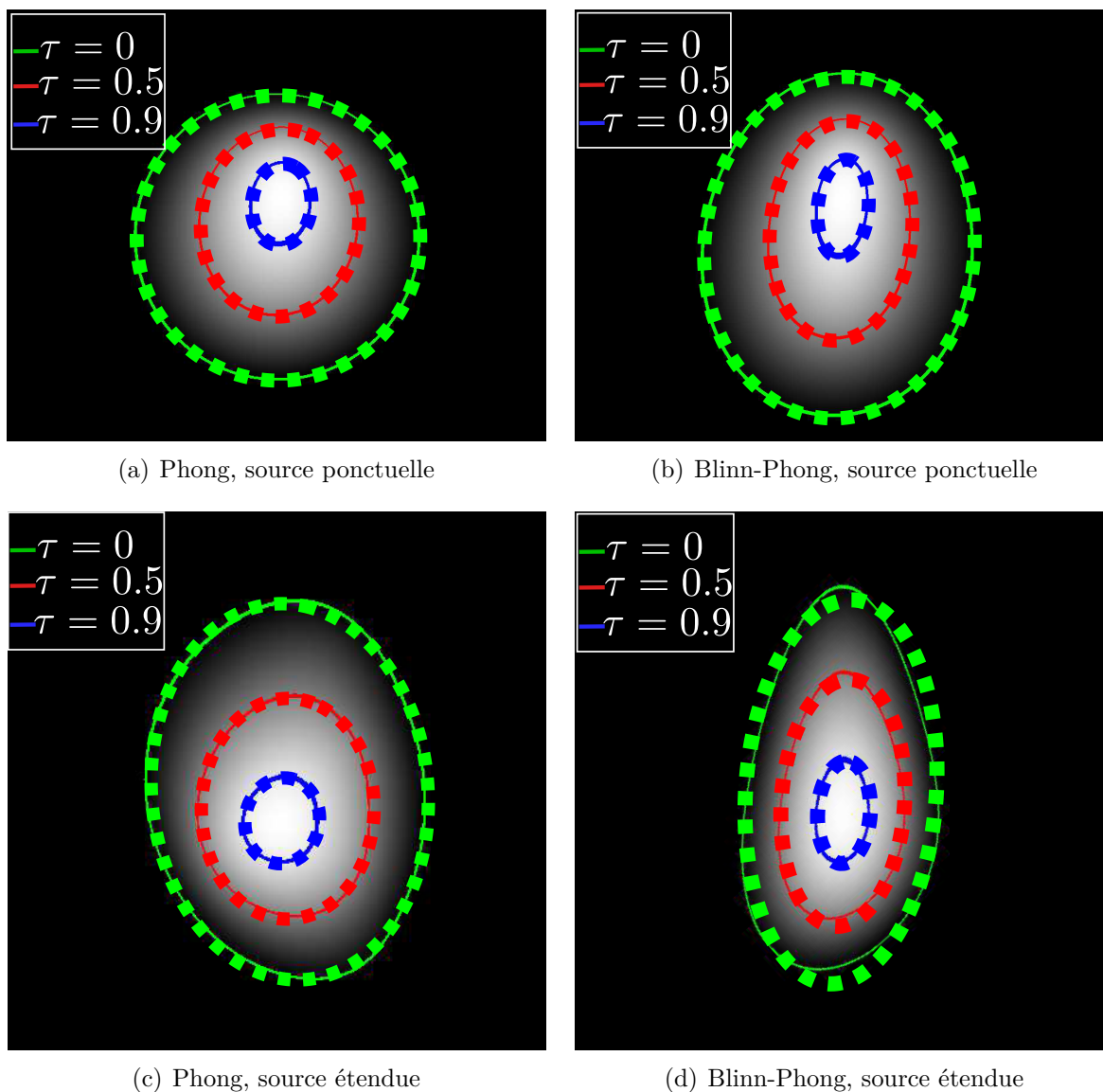
FIGURE 4.2 – Illustration de notre hypothèse de spécularités de forme elliptique. Une spécularité est créée à partir du terme spéculaire du modèle de réflexion de Phong dans (a) pour une simple lumière ponctuelle, et dans (c) pour une source de lumière étendue (une ligne composée de plusieurs sources ponctuelles) et à partir du terme spécularité du modèle de réflexion de Blinn-Phong dans (b) pour une simple lumière ponctuelle et dans (d) pour une source de lumière étendue. Les spécularités sont clairement de forme elliptique dans tous ces cas. En observant ces formes dans le plan images, nous obtenons des ellipses. Nous montrons dans ces exemples les différents isocontours associés à une intensité spécifique \tau \in \{0, 0.5, 0.9\} (contours en vert, rouge et bleu) ainsi que les ellipses correspondantes (en pointillés verts, rouges et bleus). Notre hypothèse de spécularité elliptique est distinctement vérifiée dans ces exemples.
