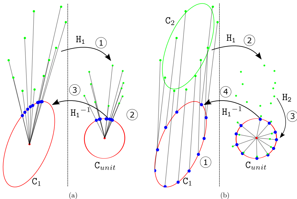
FIGURE B.6 – Amélioration des limitations de la paramétrisation d'ellipse classique. Dans (a), nous illustrons le problème de notre méthode précédente de paramétrisation pour des contours fortement éloignés de l'ellipse associée en appliquant les mêmes étapes que dans la figure B.4. Dans (b), nous présentons le même exemple avec notre nouvelle paramétrisation qui fournit un meilleur compromis entre répartitions des points sur l'ellipse paramétrée et distance entre points de contours et l'ellipse minimale. Nous partons de la partie gauche de la figure avec l'ellipse C_1 estimée par la projection de l'ellipsoïde. Les points de contours (vert) correspondent à nos données d'entrées avec l'ellipse C_2 (en verte) associée aux points. Nous estimons l'homographie H_1 qui transforme C_1 en cercle unitaire et centré (étape 1) et l'appliquons à C_1 , C_2 et aux points de contours (étape 2). Pour recentrer les contours, nous estimons H_2 l'homographie qui transforme C_2 en cercle unitaire centré et l'appliquons aux points de contours transformés par H_1 (étape 3). L'intersection entre le cercle unitaire et ces points (bleus à droite) transformés est calculée. Nous utilisons H_1^{-1} pour transformer ces points d'intersection sur C_1 (étape 4).
