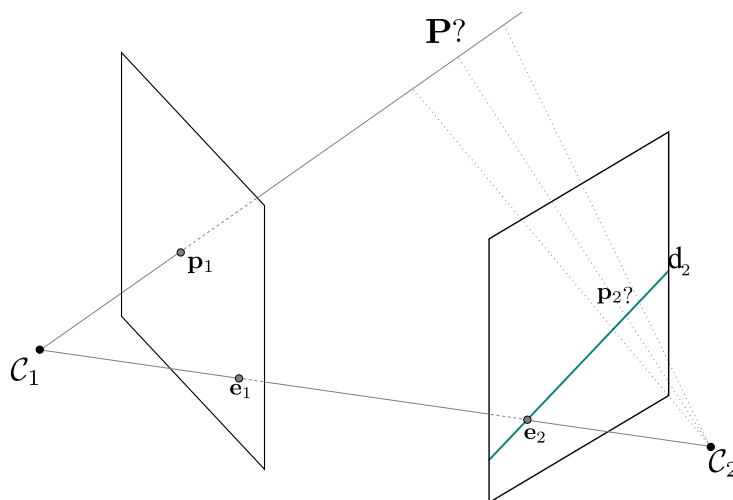
FIGURE 2.6 – Géométrie épipolaire. La géométrie épipolaire définit des contraintes géométriques entre les différentes observations d'un même point de l'espace.
