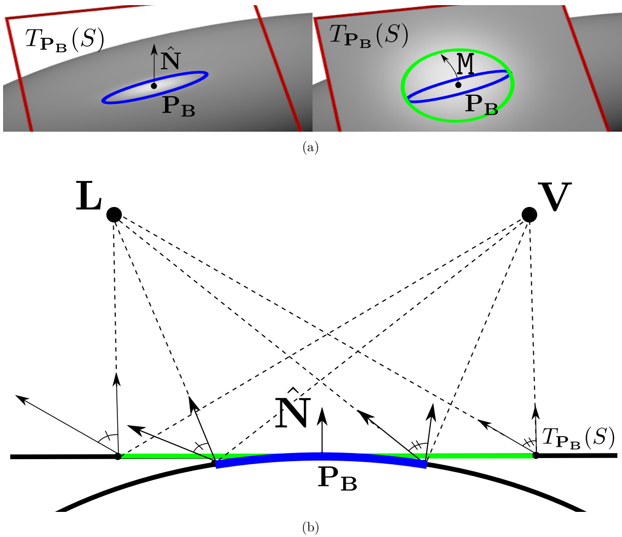
FIGURE 6.5 – Transformation d'ellipse de sa forme sur la surface courbe S en représentation canonique sur le plan tangent T_{P_B}(S) au point d'intensité maximale P_B . Dans (a), nous montrons le processus qui, à partir de l'ellipse correspondant à la spécularité (en bleu), applique la transformation M afin d'obtenir l'ellipse corrigée (en vert) dans le plan tangent T_{P_B}(S) . Dans (b), nous montrons que les angles limites conservent leurs valeurs aux contours de la spécularité sans être affectés par la courbure de la surface (bleu pour le courbe et vert pour le plan).
