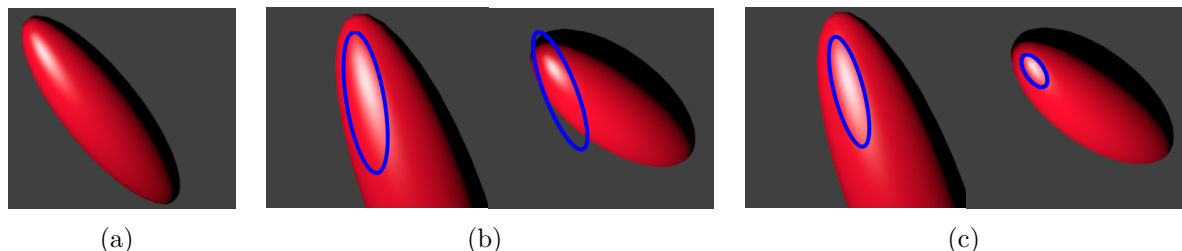
FIGURE 6.7 – Résultats de prédiction de spécularité pour notre séquence de synthèse d'ellipsoïde. Dans (a), nous montrons que l'ellipsoïde n'est pas uniforme en courbe. Dans (b) et (c), nous montrons une paire d'images de la séquence et le résultat de la prédiction de spécularité pour JOLIMAS dual (b) et JOLIMAS canonique (c). L'image de gauche correspond à la courbure utilisée pour reconstruire notre modèle et celle de droite correspond à une courbure plus importante. Nous constatons que notre modèle JOLIMAS canonique donne de meilleurs résultats pour les deux courbures contrairement à JOLIMAS dual qui reste correct, mais améliorable pour la première image, mais échoue complètement lorsque la courbure varie.
