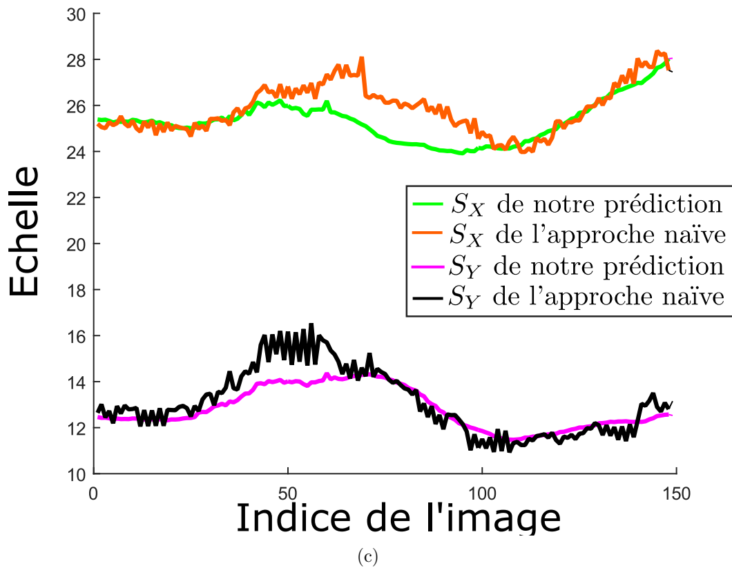
FIGURE 7.3 – Illustration d'incohérences temporelles en utilisant un calcul d'ellipse pour une application de retexturing dans une séquence multi-lumière présentée dans la figure 4.6(d) pour trois images consécutives (une image par ligne de (a) et (b)). Dans (a), un tremblement sur le processus de calcul d'ellipse est visible pour chaque spécularité où nous calculons l'ellipse directement à partir de la détection de spécularité. Ce tremblement est illustré dans (c) en mesurant l'évolution des demi-axes ( S_x et S_y ) de l'ellipse calculée (approche basique) comparée à l'ellipse prédite par notre modèle (JOLIMAS) pour chaque image de la séquence du tableau présenté dans la figure 4.6(a). Dans (b), nous copions directement le résultat de la détection de spécularité sur la nouvelle texture, ce qui provoque un décalage en termes d'intensité qui est difficile à estomper avec la texture. De plus, cette méthode est sensible à la qualité de la détection de spécularité et ne peut pas prédire de nouveaux points de vue.
