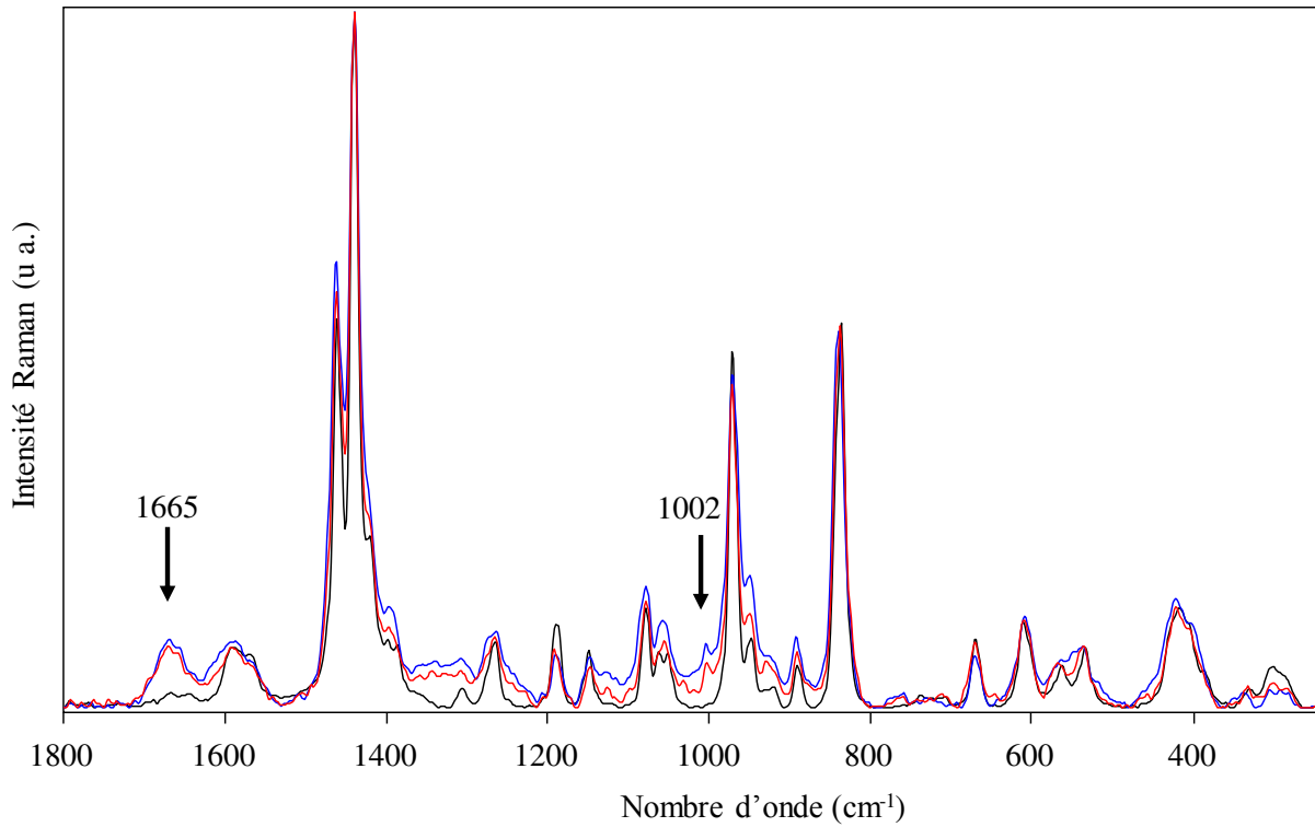
Figure 48 : Spectre RAMAN du sel de \text{Ca}_3\text{Cit}_2 (—) et des dépôts des essais B (—) et C (—) entre 1800 et 250 \text{cm}^{-1} . Analyse effectuée à la longueur d'onde \lambda de 1064 nm. Spectre avec correction de la ligne de base et mise à l'échelle.
