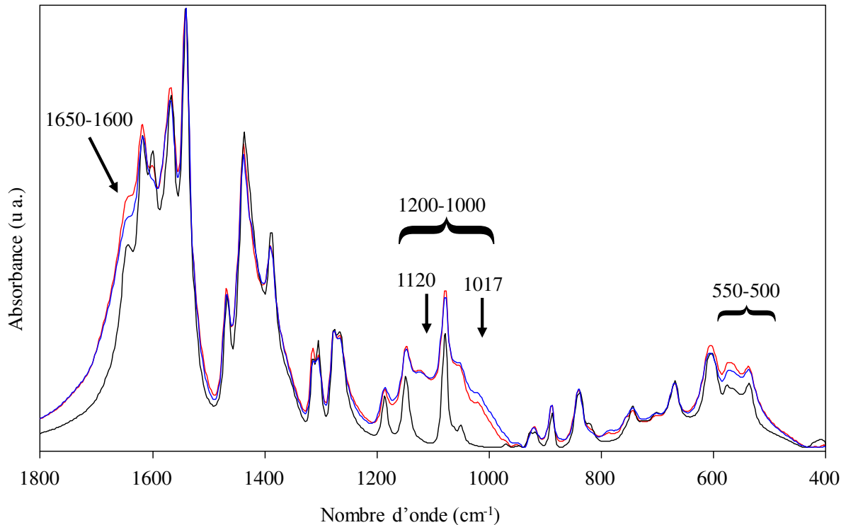
Figure 47 : Agrandissement du spectre FTIR du sel de \text{Ca}_3\text{Cit}_2 (—) et des dépôts des essais B (—) et C (—) sur la zone 1800-400 \text{cm}^{-1}
