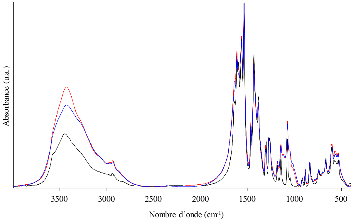
Figure 46 : Spectres FTIR du sel de \text{Ca}_3\text{Cit}_2 (—) et des dépôts des essais B (—) et C (—) – spectres avec mise à l'échelle et correction de la ligne de base
