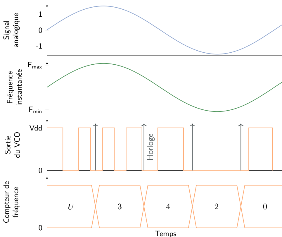
FIGURE I.10 – Visualisation des signaux lors d'une conversion par un ADC basé sur un VCO.
