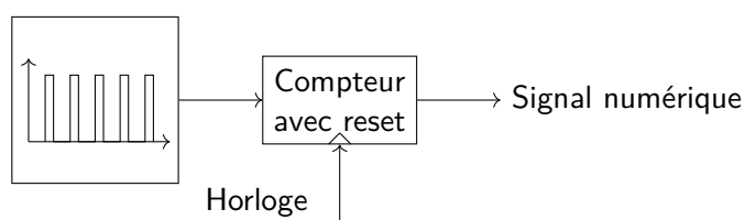
FIGURE I.18 – Exemple de calcul avec des trains de pulses et une horloge.
