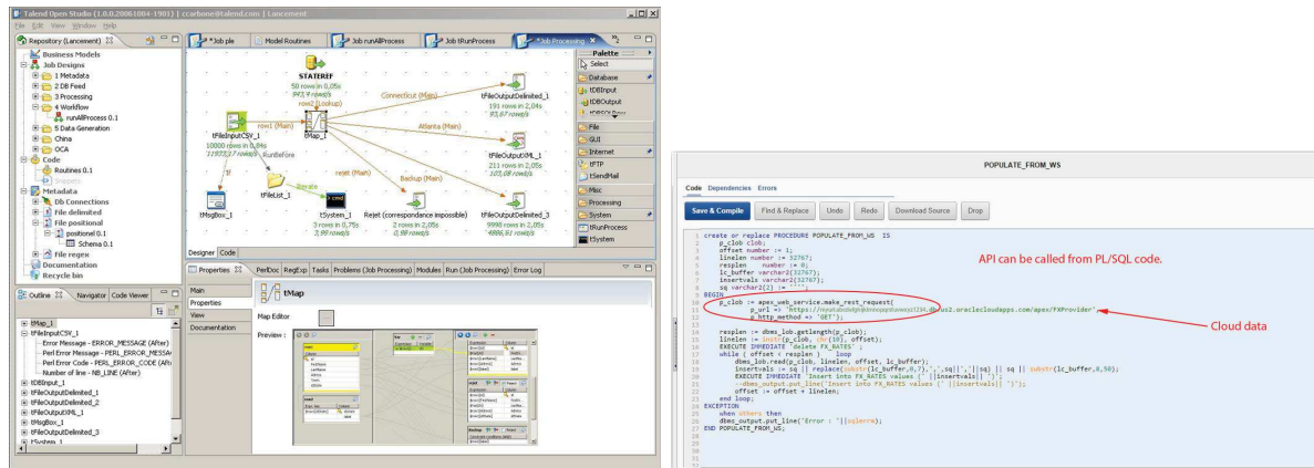
FIGURE 3.3: Comparaison Interface graphique d'un outil ETL et du code pur
