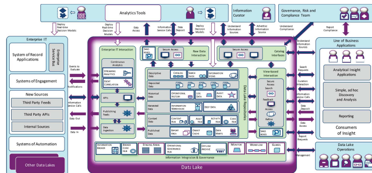
FIGURE 4.2: Architecture de Référence d'un lac de données proposée par IBM [10]
