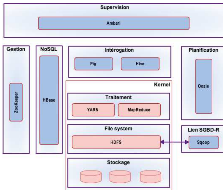
FIGURE 3.24: Vue de la plateforme Apache Hadoop
