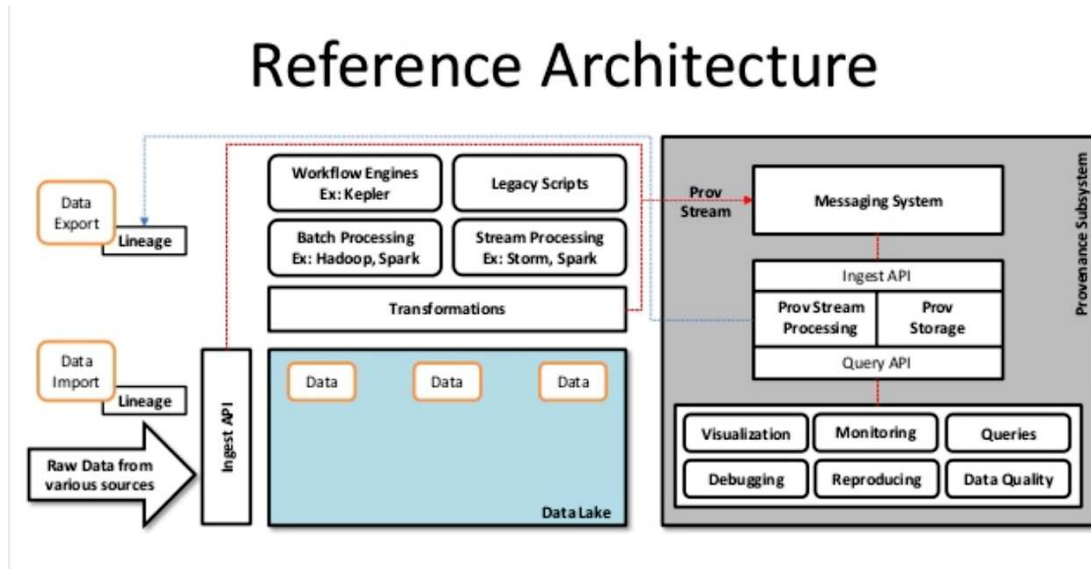
FIGURE 4.3: Architecture de Référence d'un lac de données proposée par [73]
