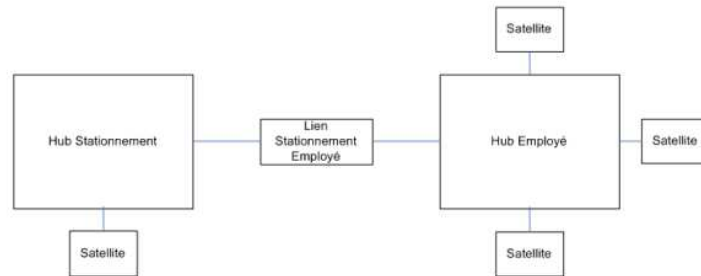
FIGURE 3.16: Modèle de Data Vault
