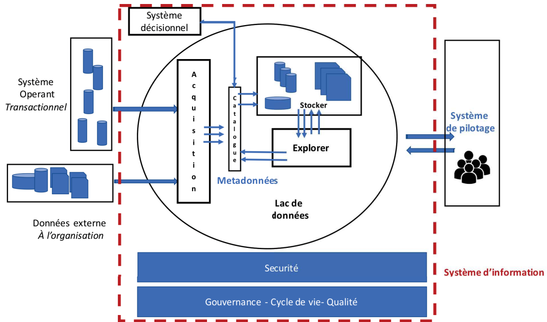
FIGURE 4.13: Macro composant ou fonctions d'un lac de données
