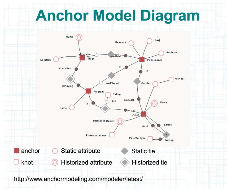
FIGURE 3.15: Modélisation de type ANCHOR MODELING
