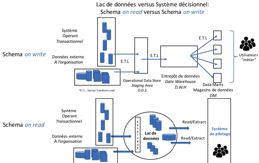
FIGURE 4.8: Lac de données versus Système décisionnel : Schema on read versus schema on write
