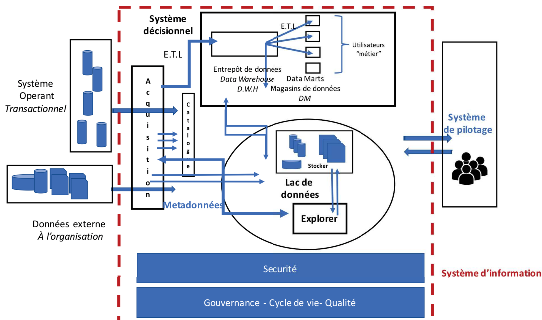
FIGURE 4.14: Mutualisation du composant acquisition entre le système décisionnel et le lac de données
