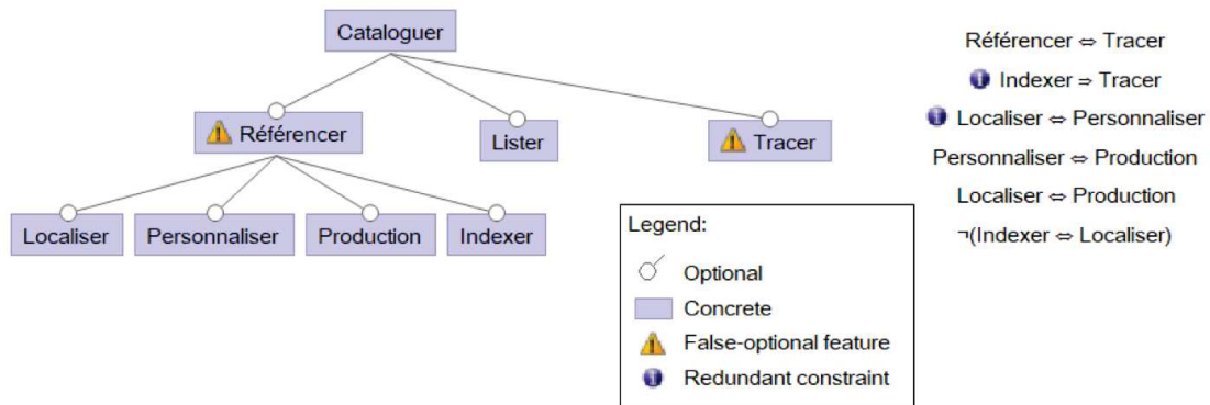
FIGURE 6.1: Feature Model de la fonctionnalité cataloguer
