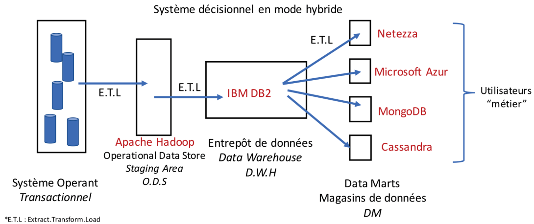
FIGURE 3.6: Système décisionnel avec une architecture hybride des stockages.
