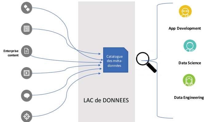
FIGURE 4.11: Architecture fonctionnelle d'un lac de données
