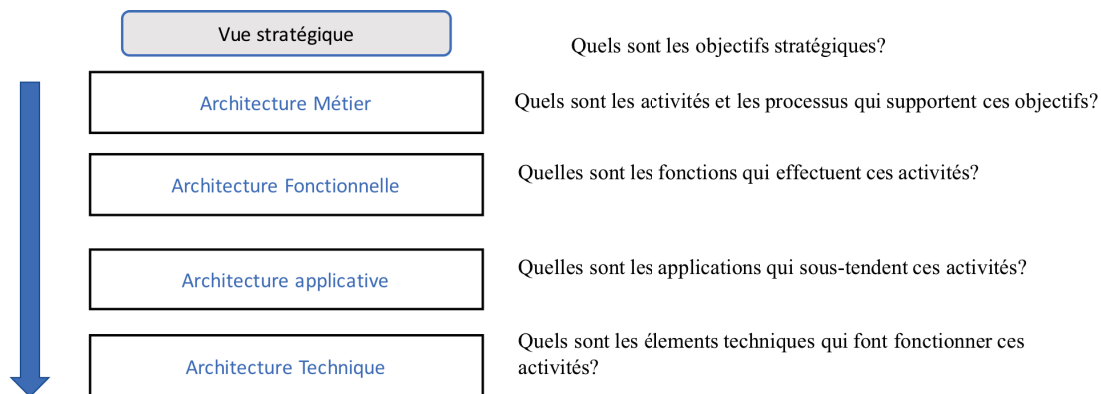
Démarche d'urbanisation du Système d'information
