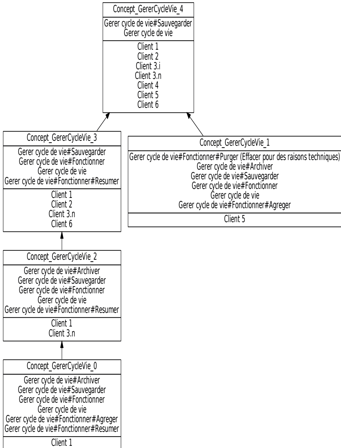
FIGURE 8.40: AOC-Gérer-plein
