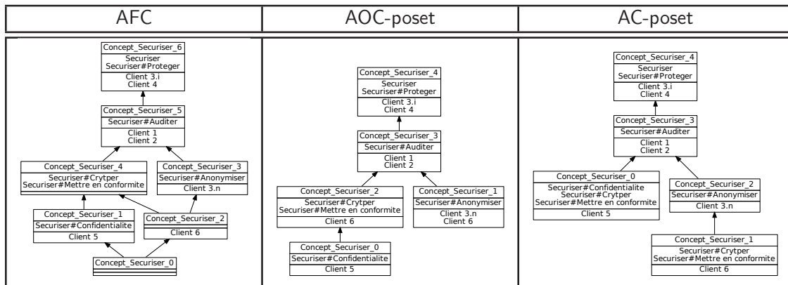
FIGURE 6.10: Comparaison de trois formats de treillis sur la fonction Sécuriser
