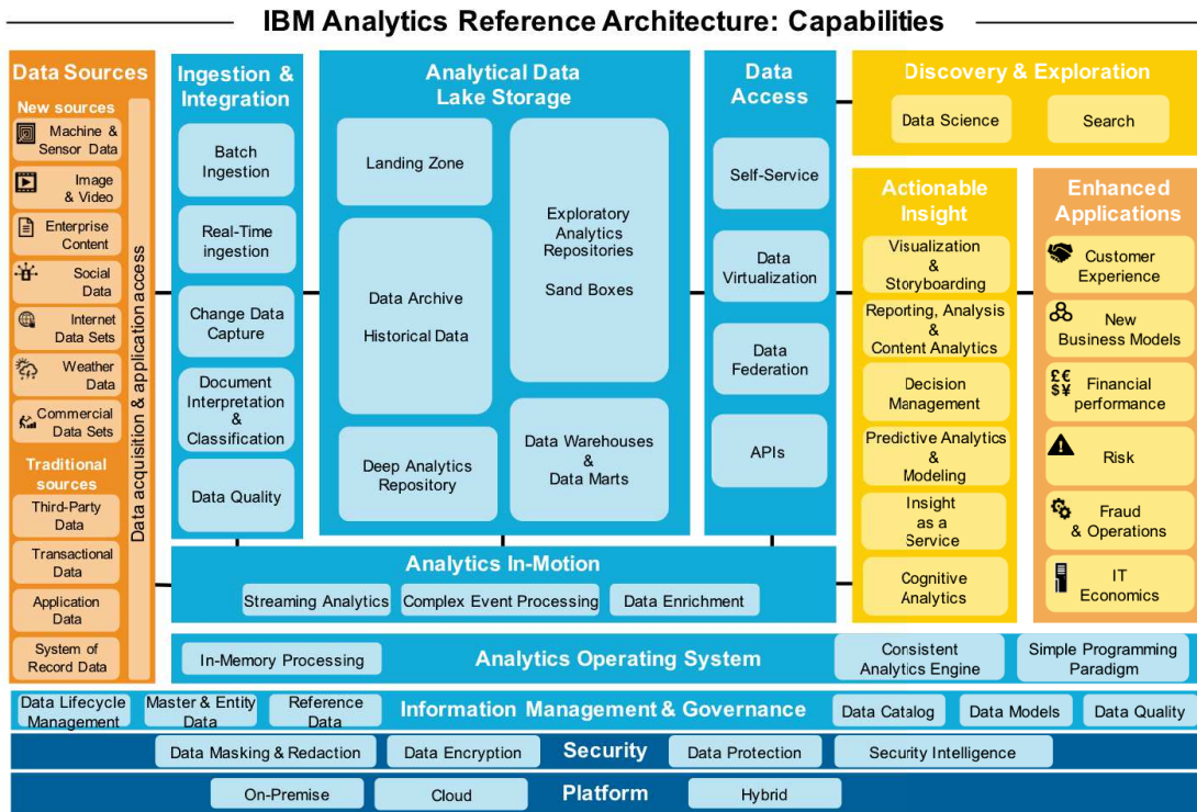
FIGURE 3.31: Architecture de référence analytique d'IBM
