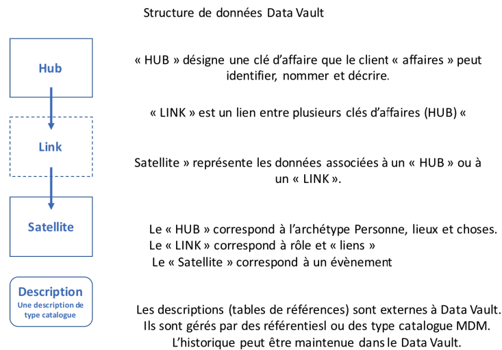
FIGURE 3.14: Structure de données du data Vault
