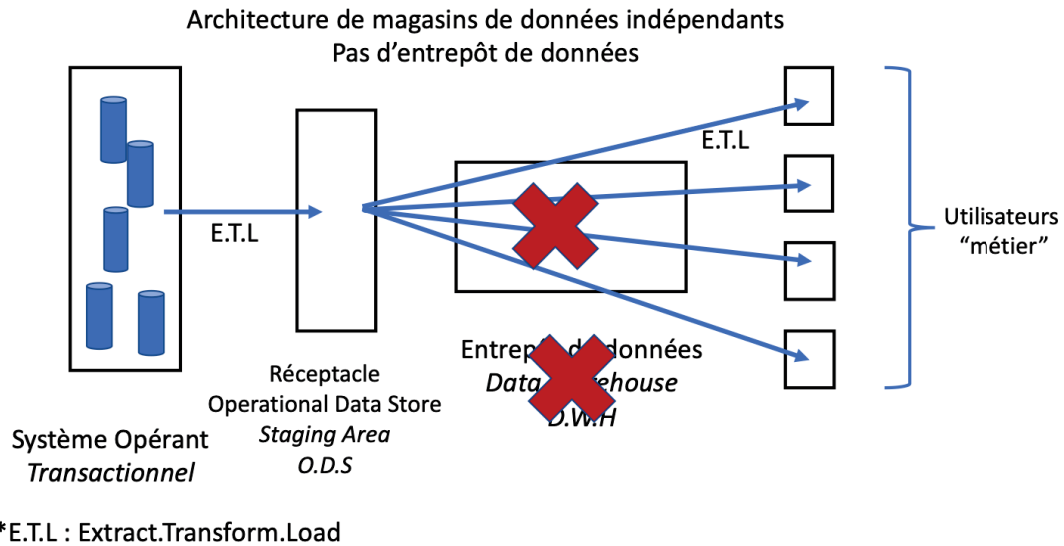
FIGURE 2.6: Architecture Décisionnelle pour des magasins de données indépendants
