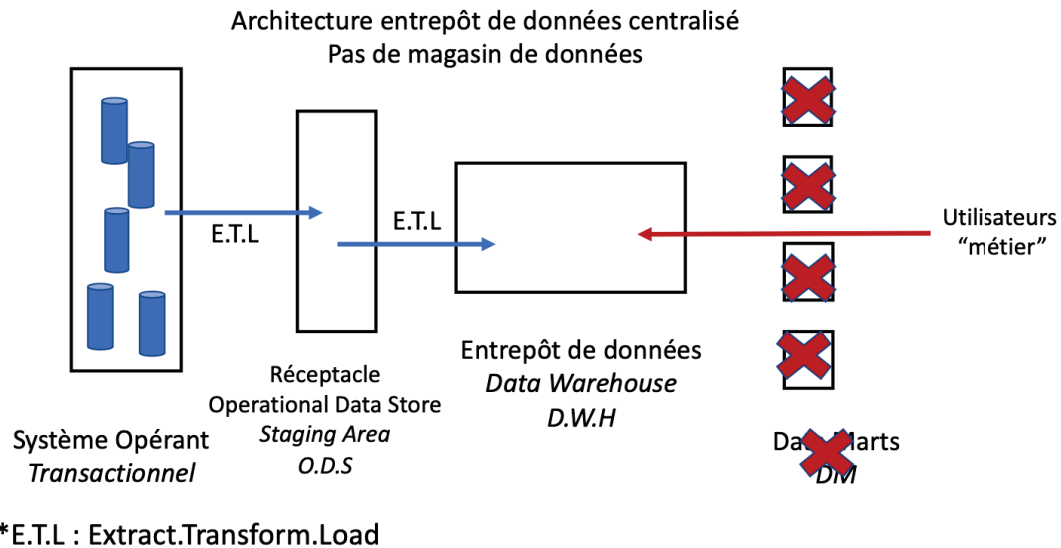
FIGURE 2.5: Architecture Décisionnelle pour un entrepôt central d'entreprise
