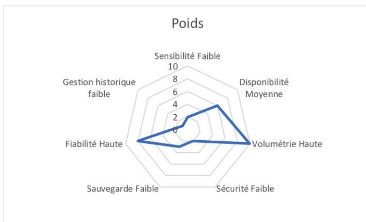
FIGURE 5.4: Évaluation initiale des contraintes non fonctionnelles pour le lac de données métrologie
