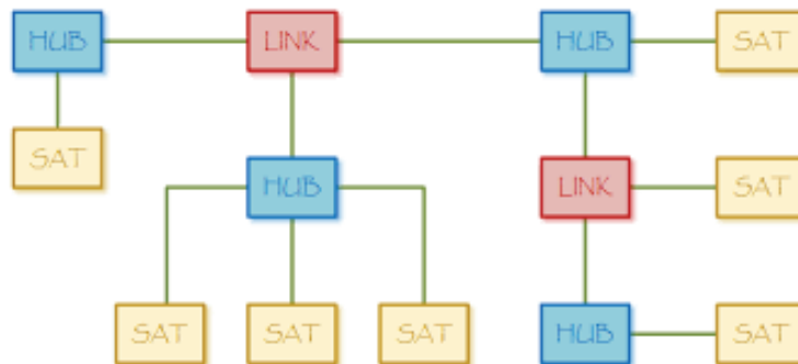
FIGURE 3.18: Exemple de Modélisation Data Vault
