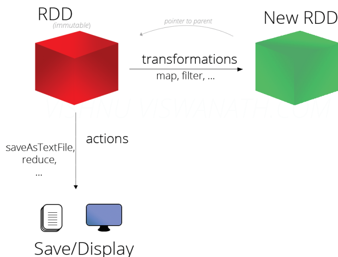
FIGURE 3.30: Mode de fonctionnement d'un Resilient Distributed Datasets -RDD avec Spark
