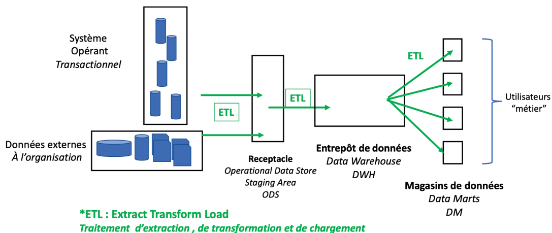
FIGURE 2.4: Vue d'une architecture de système décisionnel d'entreprise
