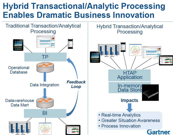
FIGURE 3.7: Description d'une architecture de type HTAP par le Gartner
