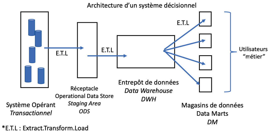
FIGURE 2.7: Architecture Décisionnelle d'un système décisionnel d'entreprise
