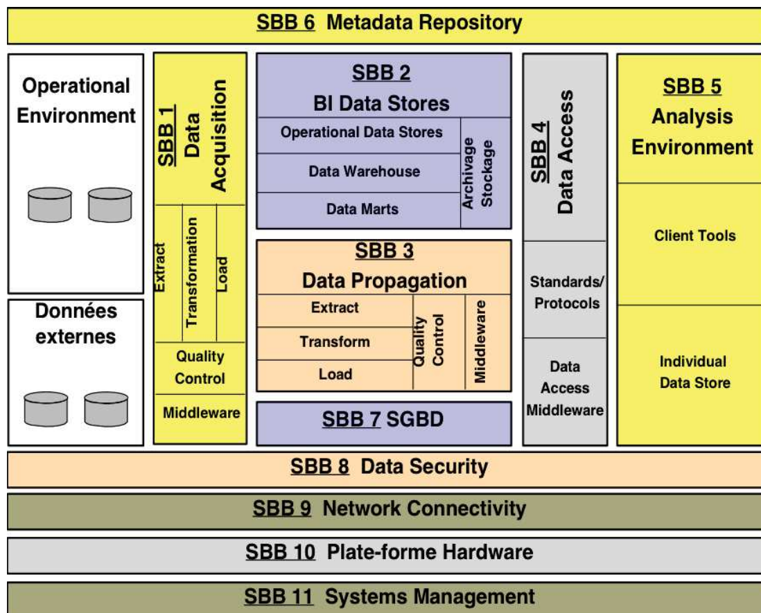
FIGURE 2.8: Architecture de référence décisionnelle - IBM
