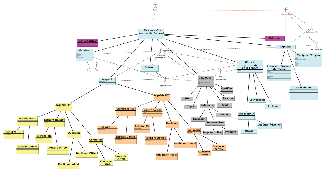
FIGURE 6.2: Modélisation d'un lac de données par fonctionnalités
