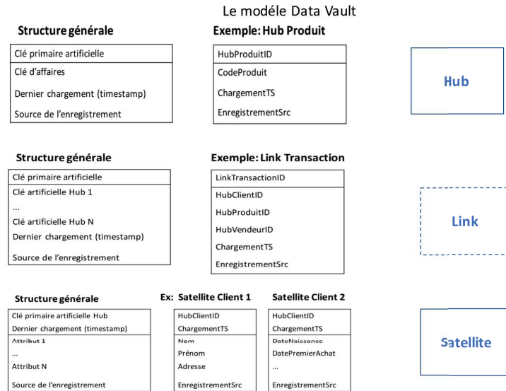
FIGURE 3.17: Synthèse des trois entités d'une modélisation Data Vault
