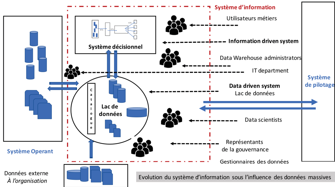
FIGURE 4.7: Interaction des lacs de données dans les systèmes d'une organisation
