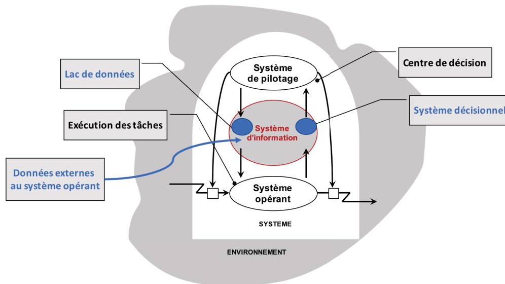
FIGURE 4.6: Proposition de positionnement des Lacs de données dans le Système d'information
