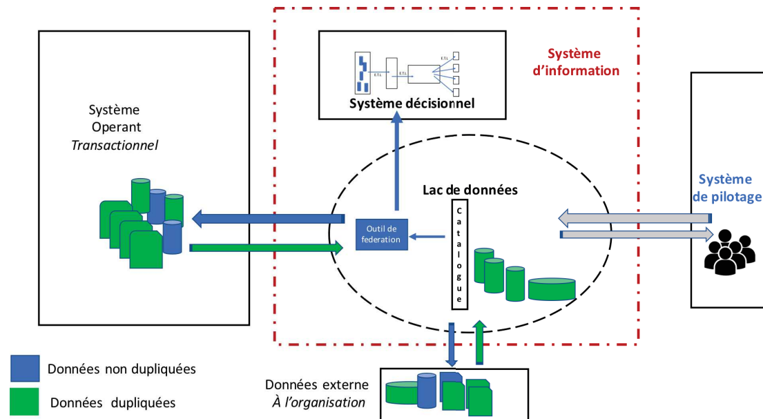
FIGURE 5.2: Architecture d'un lac de données mixte - en mode fédération et duplication
