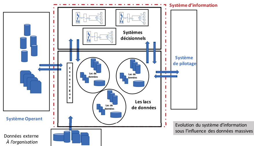
FIGURE 4.16: Vision d'une architecture globale du système d'information, sous l'influence des données massives
