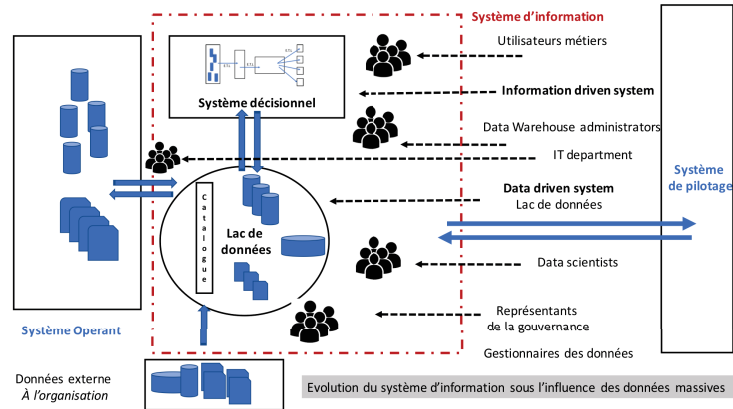
FIGURE 4.15: Interaction des lac de données dans les systèmes d'une organisation
