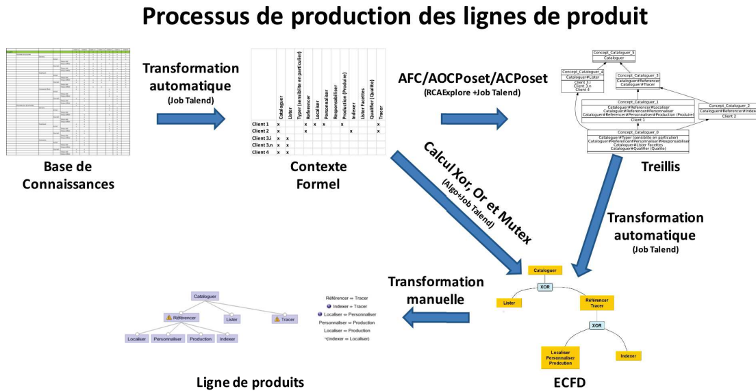
FIGURE 6.4: Processus de production des lignes de produit appliqués dans ces travaux.
