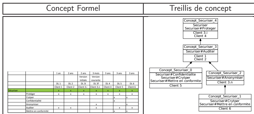
FIGURE 6.9: Contexte formel et treillis de concepts associés à la caractéristique "Securiser" des lacs de données
