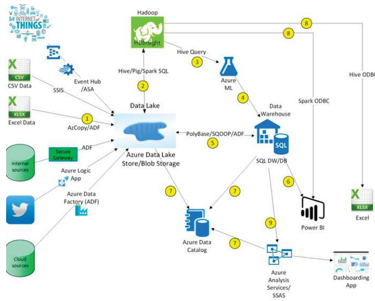
FIGURE 4.12: Architecture applicative d'un lac de données
