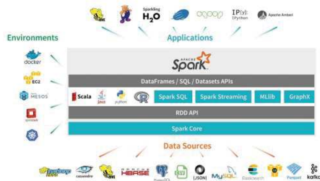
FIGURE 3.28: Description et composants de Apache Spark
