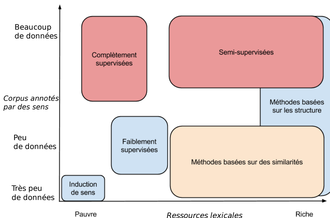
FIGURE 2.2: Les différentes méthodes de désambiguïstation lexicale [Schwab, 2017]
