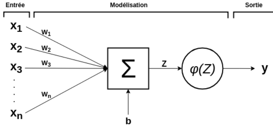
FIGURE 3.6: Structure d'un neurone artificiel
