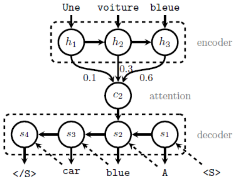
FIGURE 3.10: Illustration d'un modèle «sequence-to-sequence» avec Mécanisme d'attention [Bérard, 2018]
