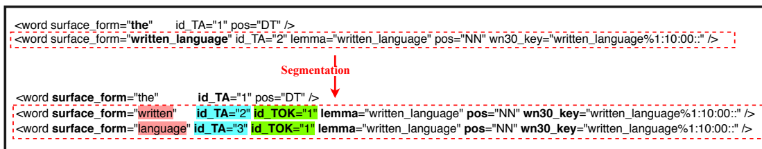
FIGURE 4.6: Exemple de normalisation du mot composé "written_language"
