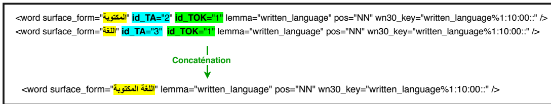
FIGURE 4.9: Concaténation des mots suivant la cible
