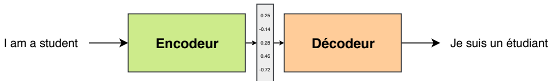
FIGURE 3.5: Processus d'apprentissage
