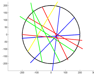
Figure C.34 – Évitement à 10 avions (pb34)
