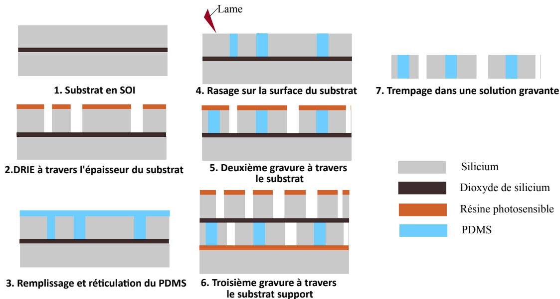
FIGURE 4.3 – Procédure de fabrication pour l'intégration du PDMS dans une structure en silicium présenté dans [Gerratt et al., 2010].
