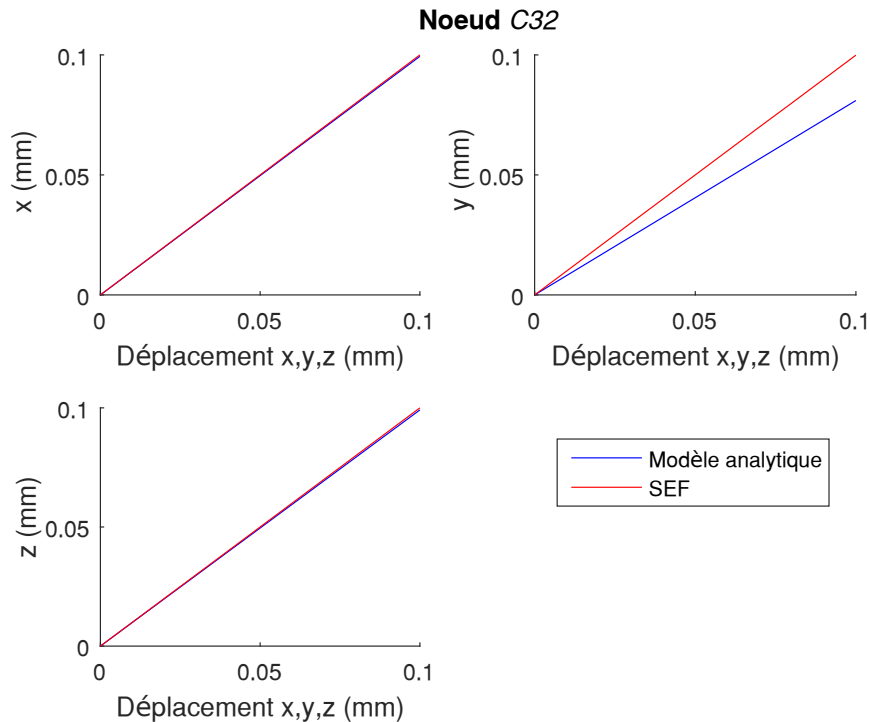
FIGURE 5.8 – Comparaison entre les résultats obtenus avec le modèle analytique et ceux obtenus avec ANSYS™ au niveau du nœud C32 .
