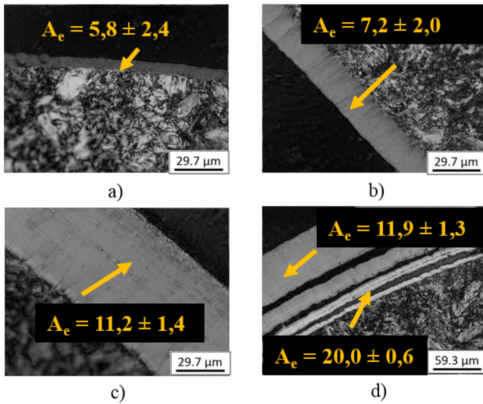
FIGURE D.4 – Cartographie d’anisotropie obtenues pour les dépôts réalisés durant 25 min à partir de butanol à : a) 1100°C, b) 1200°C, c) 1300°C et 1400°C
