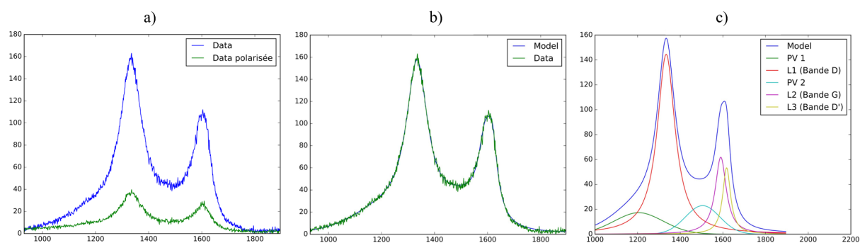
FIGURE E.26 – Dépôt de PyC à 1200°C à partir d'hexanol a) Spectres RMS avec et sans polariseur, b) Fit du spectre RMS sans polariseur et c) dé-convolution du spectre RMS sans polariseur
