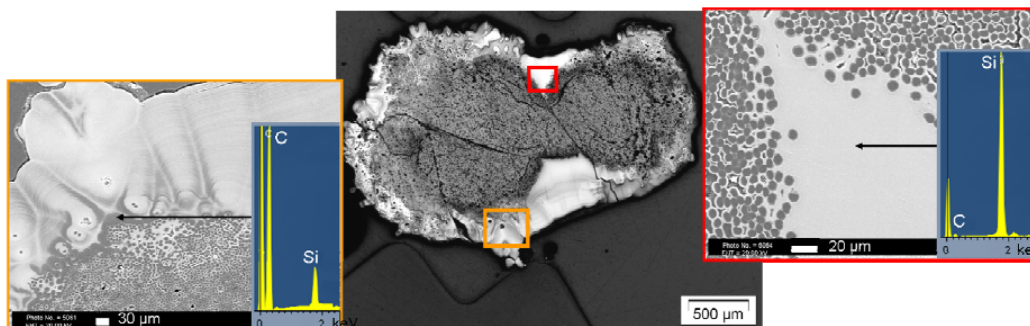
FIGURE I.3.5 – Cliché MO d'un dépôt élaboré à 1000°C pendant 60 min, clichés MEB des parties concaves (encadré rouge) et convexes (encadré orange) et pointés EDS associés [Serre_2013]
