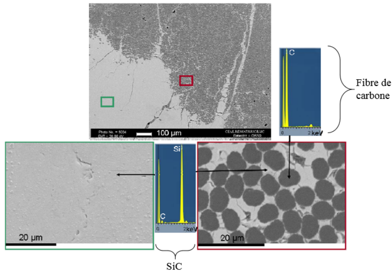
FIGURE I.3.11 – Clichés MEB et pointés EDS de fibres de carbone densifiées par caléfaction à 700°C pendant 90 min à partir de CVD 4000 [Serre_2013]
