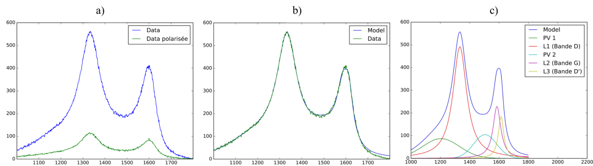
FIGURE E.20 – Dépôt de PyC à 1400°C à partir de butanol a) Spectres RMS avec et sans polariseur, b) Fit du spectre RMS sans polariseur et c) dé-convolution du spectre RMS sans polariseur
