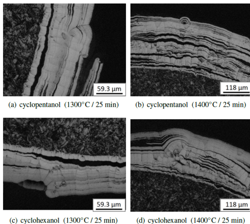
FIGURE III.3.9 – Clichés de MO montrant les délaminages des dépôts élaborés à haute température pour le cyclopentanol et le cyclohexanol
