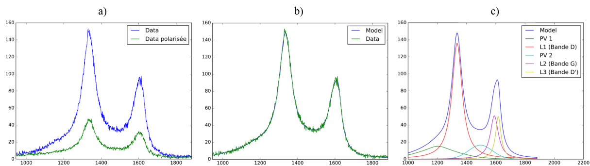
FIGURE E.15 – Dépôt de PyC à 1235°C à partir de propanol a) Spectres RMS avec et sans polariseur, b) Fit du spectre RMS sans polariseur et c) dé-convolution du spectre RMS sans polariseur
