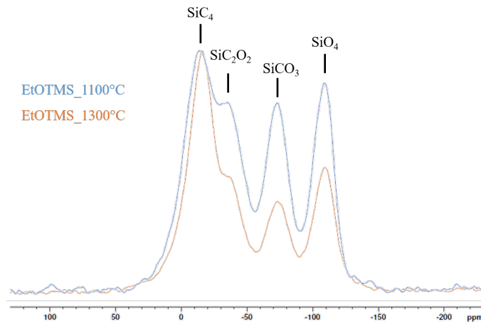
FIGURE IV.3.3 – Influence de la température sur la structure de la phase \text{SiC}_x\text{O}_{2(1-x)}
