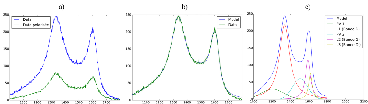
FIGURE E.3 – Dépôt de PyC à 1300°C à partir de cyclohexane a) Spectres RMS avec et sans polariseur, b) Fit du spectre RMS sans polariseur et c) dé-convolution du spectre RMS sans polariseur
