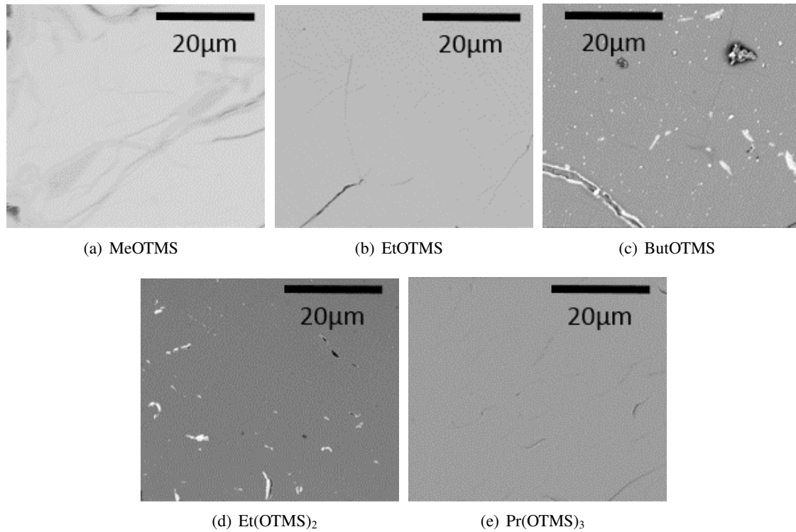
FIGURE IV.2.3 – Clichés MEB/BSED montrant les dépôts obtenus à 1100^{\circ}\text{C} pendant 20 min pour chaque précurseur
