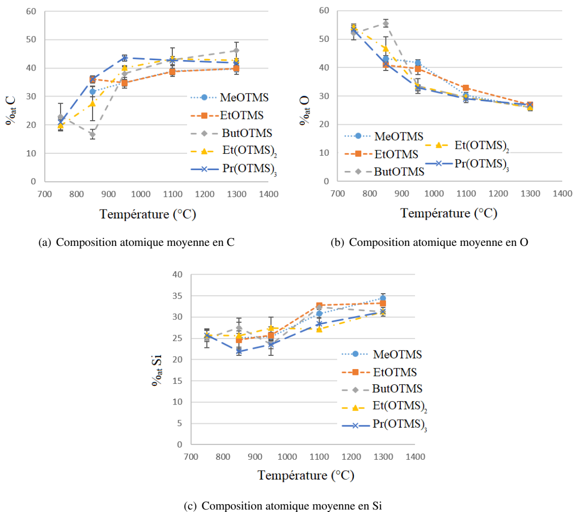
FIGURE IV.2.17 – Évolution de la composition chimique des revêtements en fonction de la température et du précurseur utilisé
