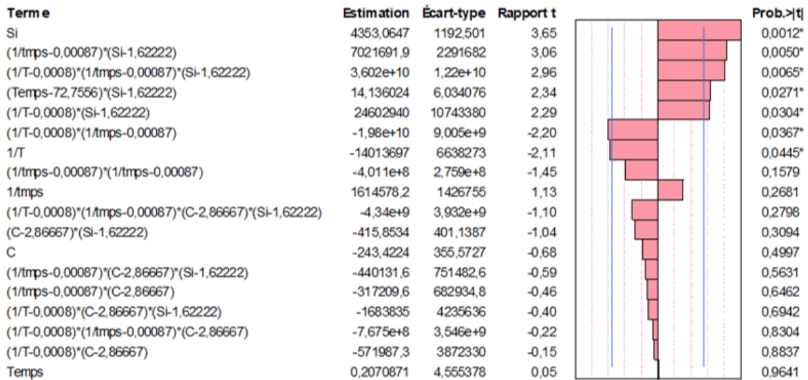
FIGURE IV.2.11 – Étude de sensibilité des régresseurs du modèle pour les précurseurs Si-O-C
