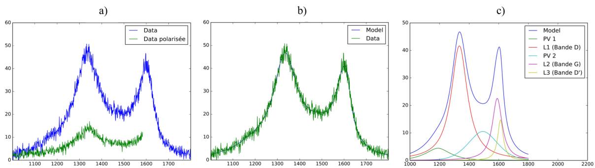
FIGURE E.36 – Dépôt de PyC à 1400°C à partir de cyclohexanol a) Spectres RMS avec et sans polariseur, b) Fit du spectre RMS sans polariseur et c) dé-convolution du spectre RMS sans polariseur
