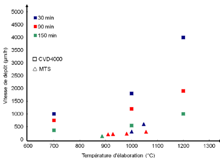
FIGURE I.3.12 – Vitesses de croissance des dépôts (en \mu\text{m/h} ) élaborés par caléfaction sur des fibres de carbone à partir de CVD 4000 et de MTS en fonction de la température [Serre_2013]
