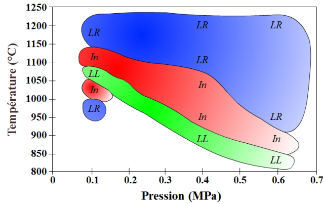
FIGURE I.3.3 – Domaines d'existence des microstructures de PyC en fonction de la pression et de la température pour une densification à partir de toluène [Beaugrand_2000]
