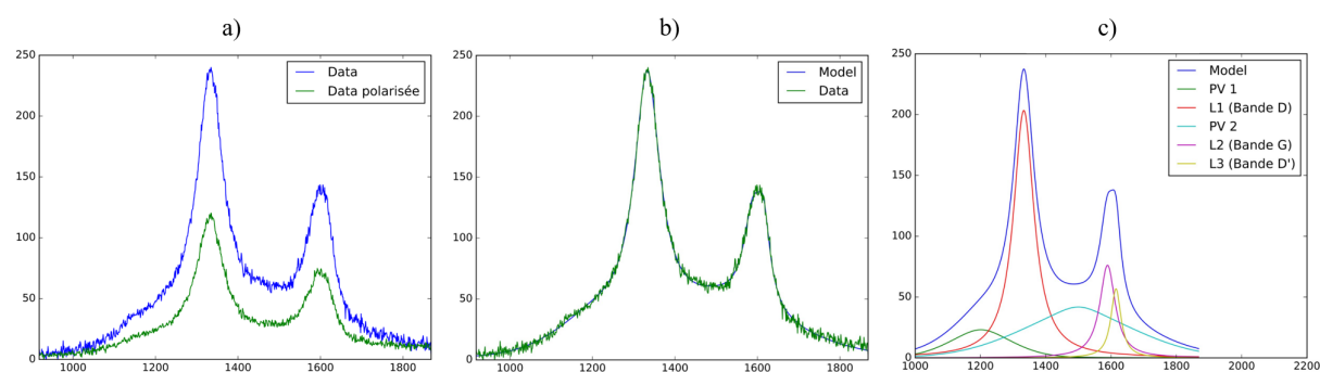
FIGURE E.17 – Dépôt de PyC à 1100°C à partir de butanol a) Spectres RMS avec et sans polariseur, b) Fit du spectre RMS sans polariseur et c) dé-convolution du spectre RMS sans polariseur
