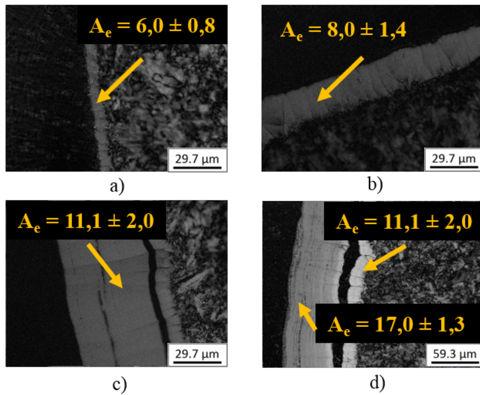
FIGURE D.5 – Cartographie d’anisotropie obtenues pour les dépôts réalisés durant 25 min à partir de pentanol à : a) 1100°C, b) 1200°C, c) 1300°C et 1400°C
