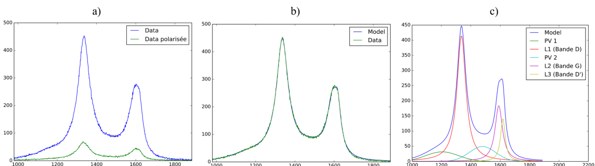
FIGURE E.10 – Dépôt de PyC à 1300°C à partir d'éthanol a) Spectres RMS avec et sans polariseur, b) Fit du spectre RMS sans polariseur et c) dé-convolution du spectre RMS sans polariseur
