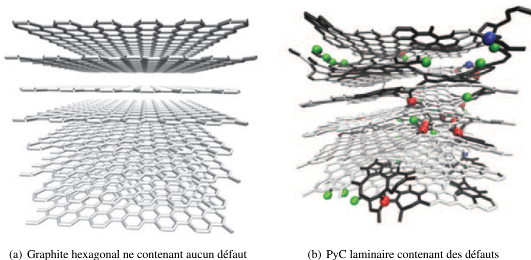
FIGURE I.2.2 – Schémas explicatifs représentant un graphite hexagonal et un PyC laminaire [Technique de l'ingénieur PyC_2015]
