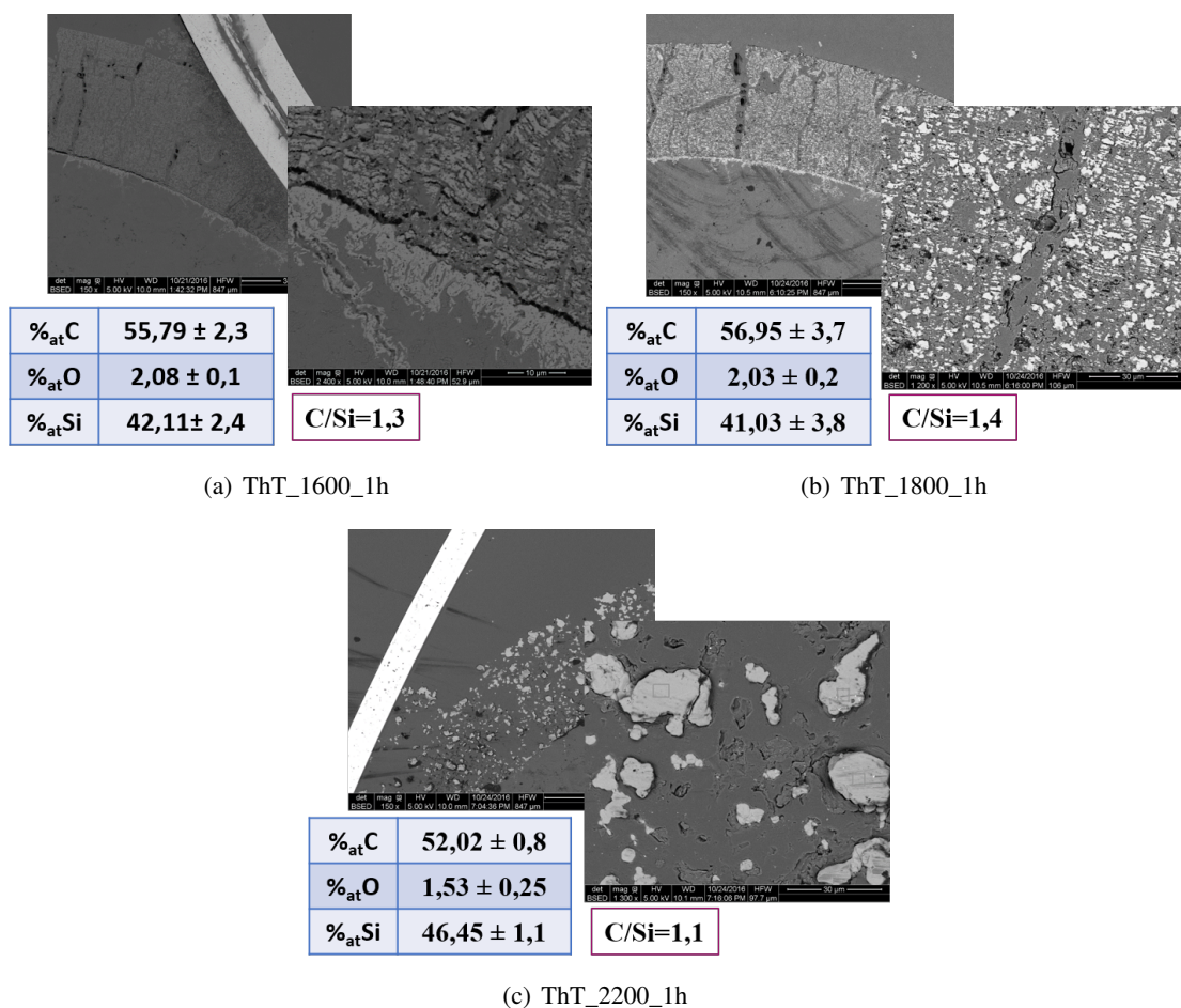
FIGURE IV.3.7 – Clichés MEB-BSED montrant les analyses chimiques et morphologiques des dépôts après traitement de carboréduction
