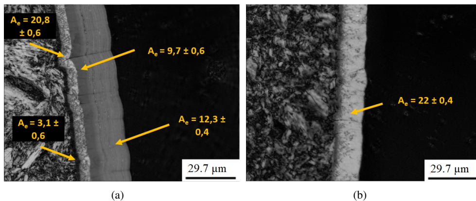
FIGURE III.3.27 – Cartographies d'anisotropie montrant le dépôt de PyC hautement anisotropique lors de l'utilisation du propanol en tant que précurseur : lors de l'essai dit "multi-couches" et b) lors de l'essai à 1235°C
