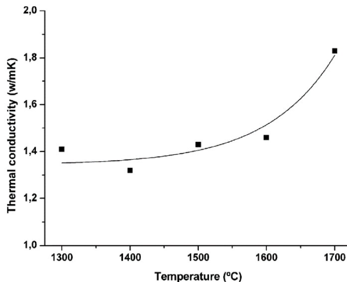
FIGURE I.2.19 – Evolution de la conductivité thermique avec l'augmentation de la température de SPS [Mazo_2017]
