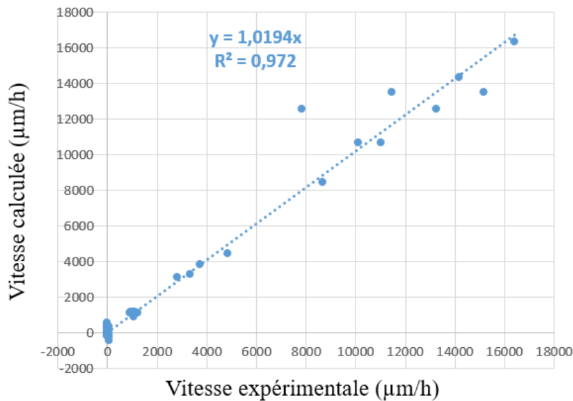
FIGURE IV.2.12 – Représentation graphique montrant les vitesses de dépôt calculées en fonction des vitesses mesurées expérimentalement
