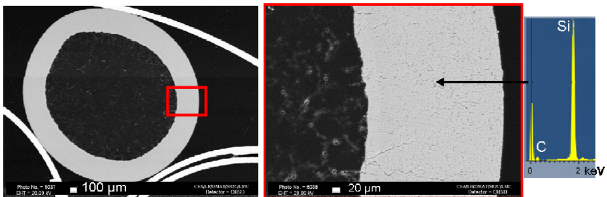
FIGURE I.3.14 – Clichés MEB et analyse EDS d'un dépôt élaboré par caléfaction à partir de HMDS à 800^\circ C pendant une durée de 90 min [Serre_2013]
