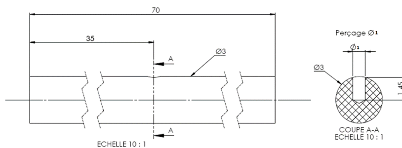
FIGURE II.2.4 – Schéma des barreaux de graphite utilisés comme substrats
