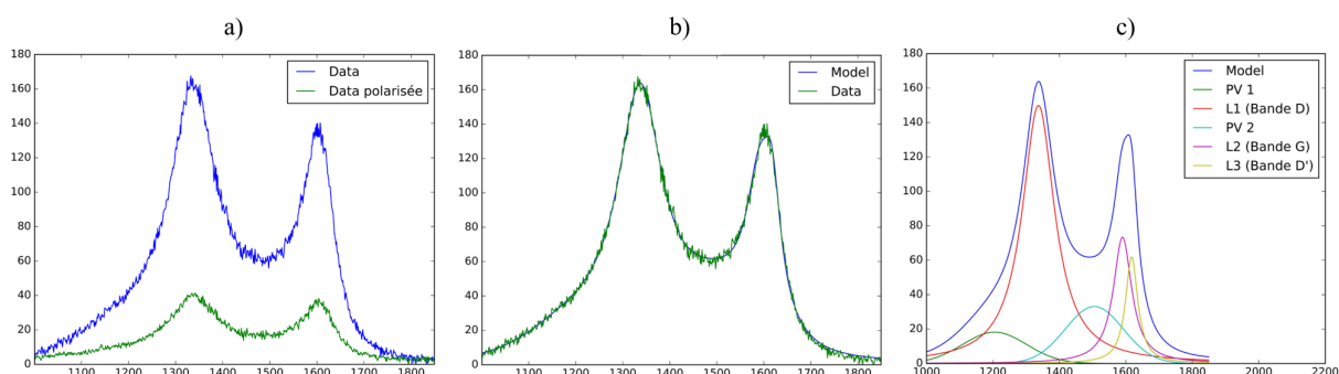
FIGURE E.28 – Dépôt de PyC à 1400°C à partir d'hexanol a) Spectres RMS avec et sans polariseur, b) Fit du spectre RMS sans polariseur et c) dé-convolution du spectre RMS sans polariseur
