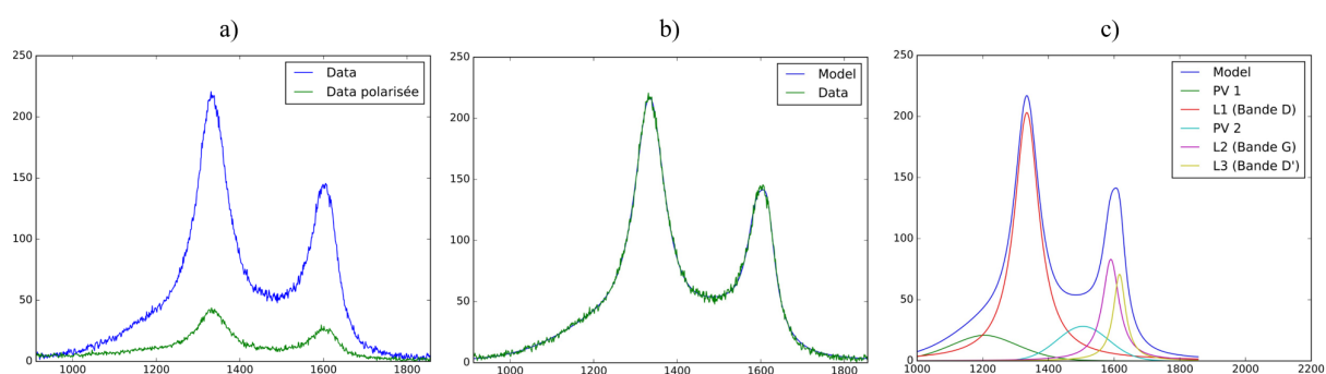
FIGURE E.25 – Dépôt de PyC à 1100°C à partir d'hexanol a) Spectres RMS avec et sans polariseur, b) Fit du spectre RMS sans polariseur et c) dé-convolution du spectre RMS sans polariseur
