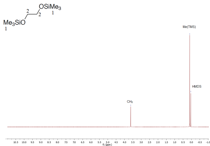
FIGURE IV.1.5 – Spectre RMN ^1\text{H} du produit issu de la synthèse relative aux paramètres du Tableau IV.1.3 entrée 2
