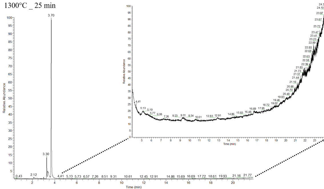
FIGURE C.7 – Chromatogrammes des résidus liquides obtenus pour l’essai à 1300°C pendant 25 min
