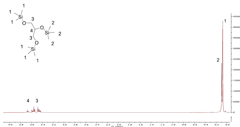
FIGURE IV.1.10 – Spectre RMN ^1\text{H} du 1,2,3-tris(triméthylsiloxy)propane avec les paramètres du Tableau IV.1.5 entrées 3 et 4
