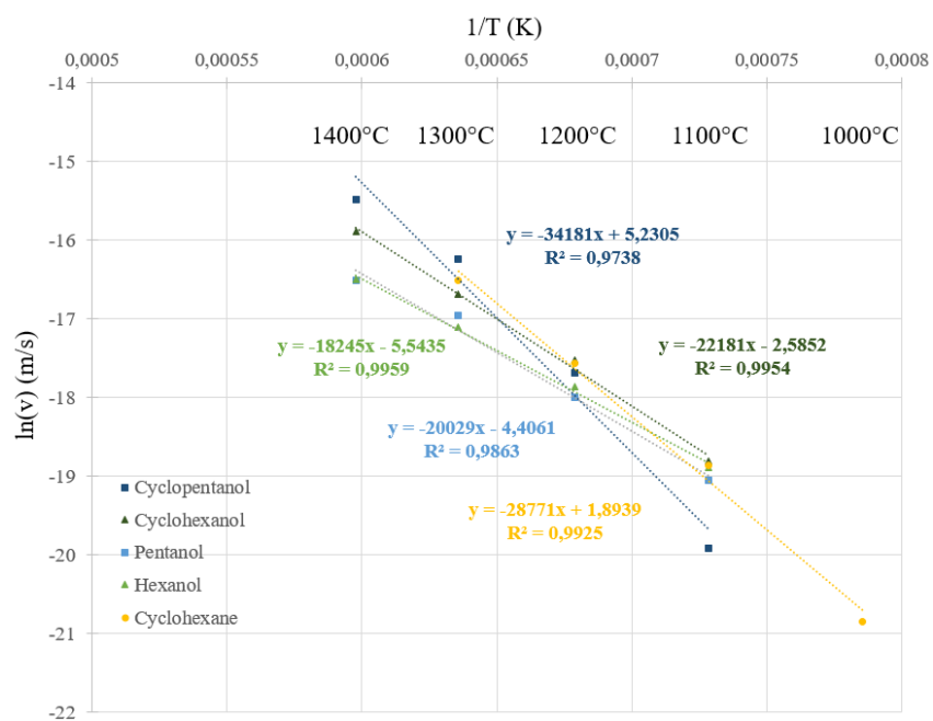
FIGURE III.3.10 – Tracé de la loi d'Arrhénius pour les alcools cycliques : comparaison avec leurs équivalents linéaires
