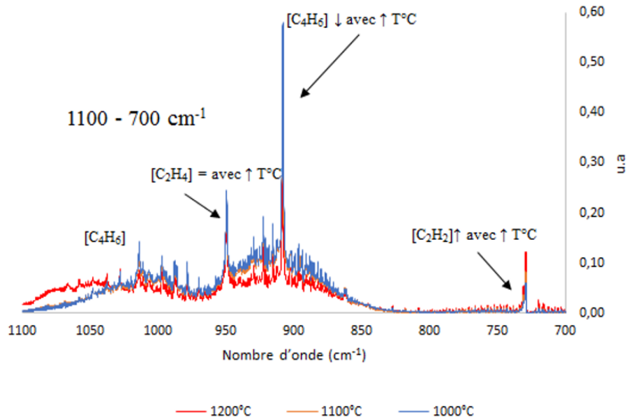
FIGURE III.1.7 – Spectres FTIR montrant l’influence de la température sur la concentration des espèces gazeuses prélevées entre 700 et 1100 \text{cm}^{-1} (normalisation par rapport au pic le plus intense du cyclohexane)
