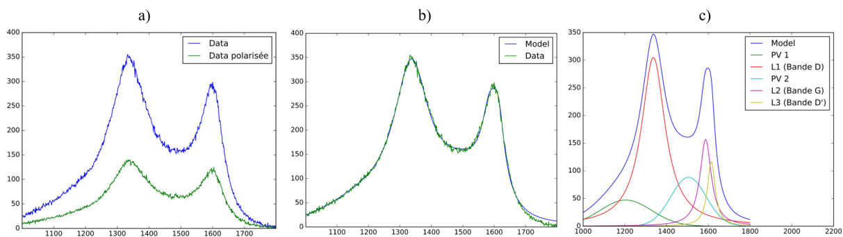
FIGURE E.2 – Dépôt de PyC à 1200°C à partir de cyclohexane a) Spectres RMS avec et sans polariseur, b) Fit du spectre RMS sans polariseur et c) dé-convolution du spectre RMS sans polariseur
