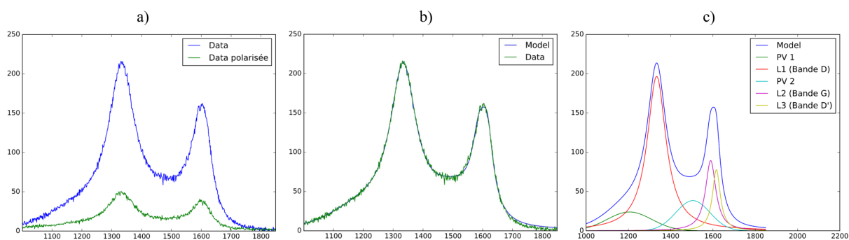
FIGURE E.24 – Dépôt de PyC à 1400°C à partir de pentanol a) Spectres RMS avec et sans polariseur, b) Fit du spectre RMS sans polariseur et c) dé-convolution du spectre RMS sans polariseur
