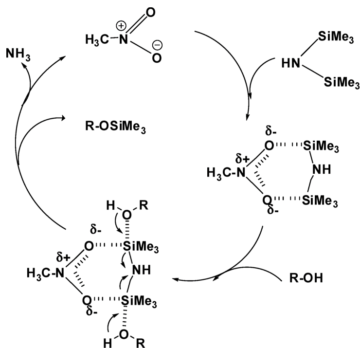
FIGURE IV.1.1 – Mécanisme réactionnel proposé par Kadam et Kim [Kadam_2010]
