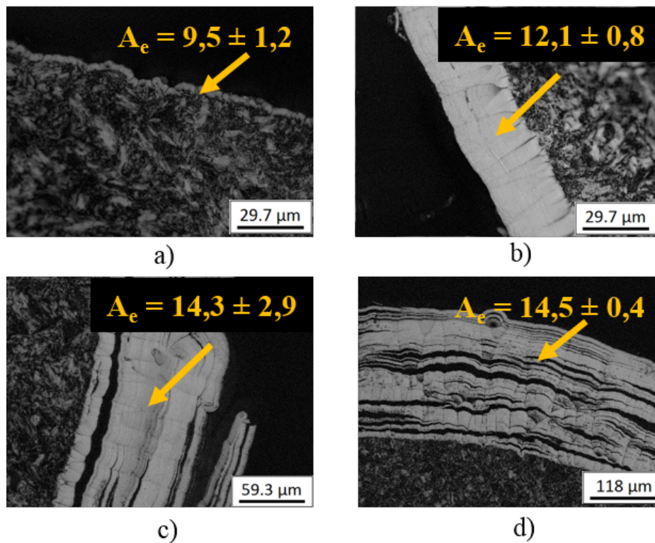
FIGURE D.7 – Cartographie d’anisotropie obtenues pour les dépôts réalisés durant 25 min à partir de cyclopentanol à : a) 1100°C, b) 1200°C, c) 1300°C et 1400°C
