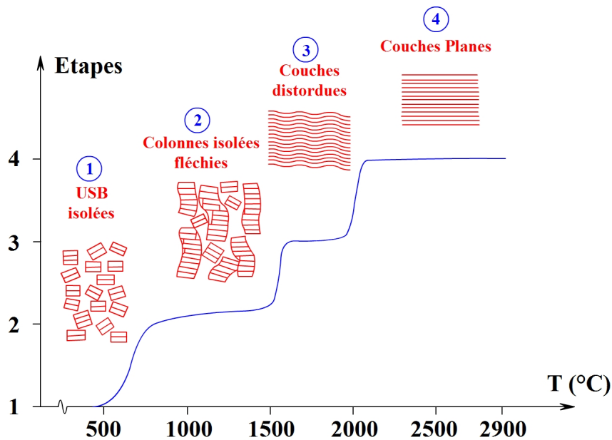
FIGURE I.2.3 – Différents stades d'organisation structurale du carbone graphitisable en fonction de la température de traitement thermique [Oberlin_1984]
