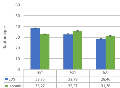
(b) Dépôt réalisé à partir de EtOTMS à 1100°C
