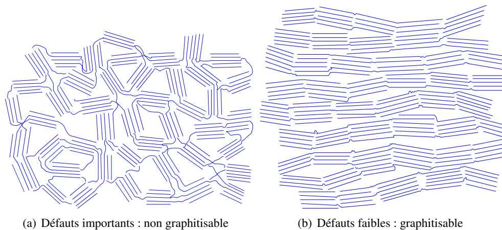
FIGURE I.2.4 – Schématisation d'un carbone non graphitisable (a) et graphitique (b) [D'après Franklin_1951]
