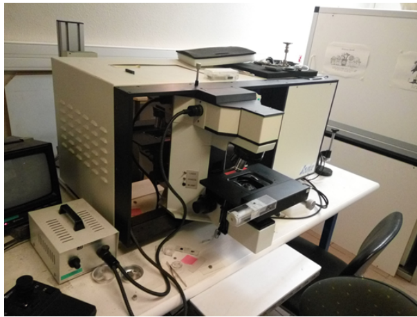
FIGURE II.3.6 – Photographie du spectroscope Raman Horiba-Jobin Yvon Labram HR équipé d'un laser polarisé d'une longueur d'onde de 632 nm
