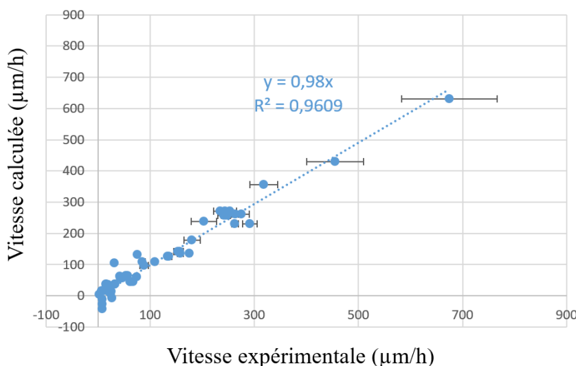
FIGURE III.3.22 – Représentation graphique de l’évolution de la vitesse mesurée expérimentalement en fonction de la vitesse modélisée pour les alcools cycliques et leur homologue linéaire
