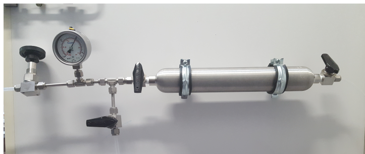
FIGURE II.2.3 – Photographie de la cartouche de gaz installée en sortie du réacteur de caléfaction
