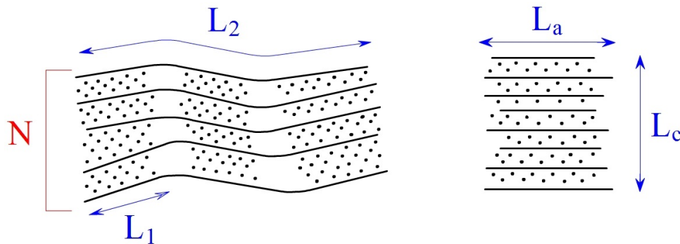
FIGURE I.2.1 – Représentation schématique d'un domaine cohérent (à gauche) et d'une USB (à droite)[Bourrat_1986, Fillon_2000, Franklin_1950]
