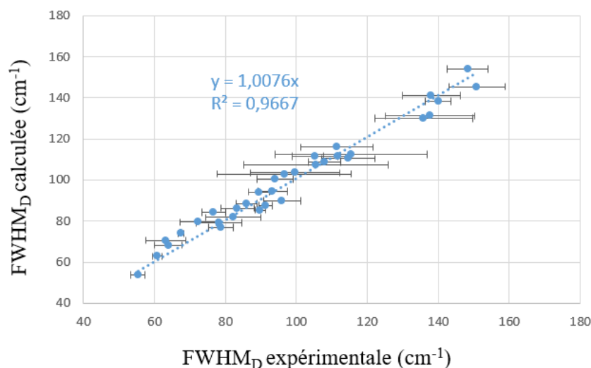
FIGURE III.3.35 – Représentation graphique de l'évolution de FWHM_D mesurée expérimentalement en fonction de FWHM_D modélisée pour tous les alcools
