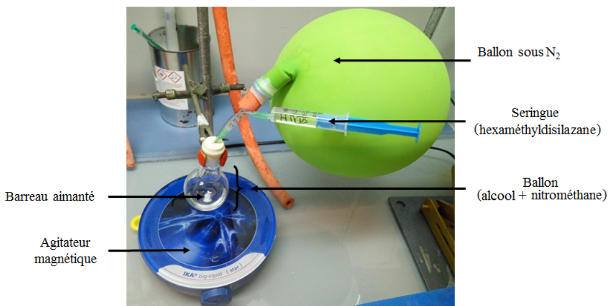
FIGURE IV.1.2 – Photographie du montage expérimental de la synthèse de précurseurs organosiliciés
