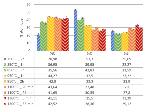
(e) Histogrammes de composition chimique relatifs à Pr(OTMS) 3
