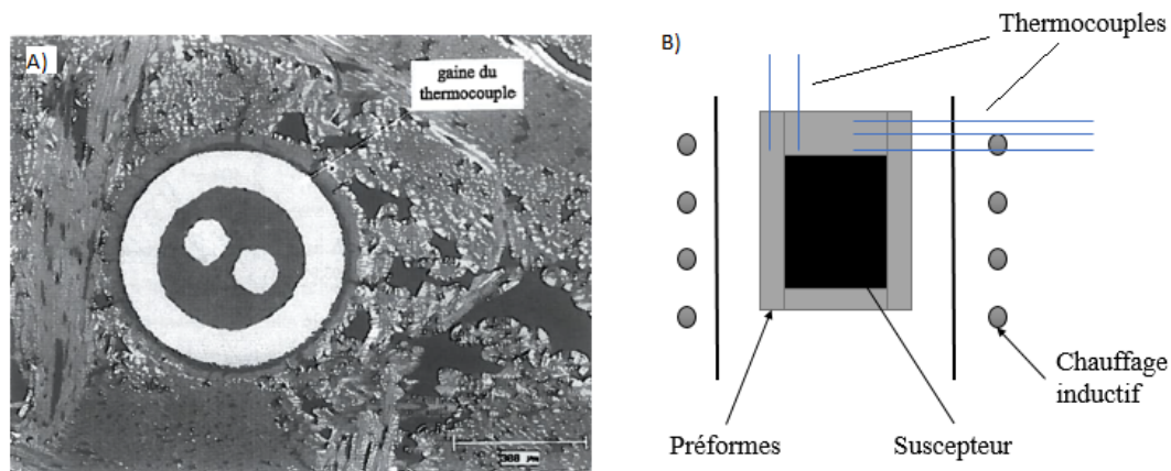
FIGURE I.3.1 – A) Cliché MEB d'un thermocouple dans une préforme densifiée par caléfaction et B) Schéma montrant la localisation des thermocouples dans une préforme lors d'une densification sur le kalamazoo [Beaugrand_2000]
