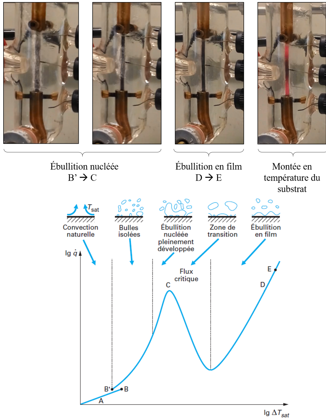
FIGURE I.1.8 – Courbe de Nukiyama représentant les différents régimes d'ébullition [Lallemand_2005] et photographies illustrant chacun de ces régimes en caléfaction
