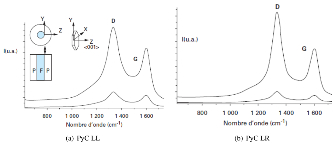
FIGURE I.2.7 – Spectres Raman de premier ordre typiques des pyrocarbones LL (a) et LR (b) déposés de façon concentrique autour d'une fibre [Technique de l'ingénieur PyC_2015]
