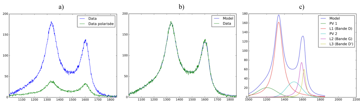
FIGURE E.27 – Dépôt de PyC à 1300°C à partir d'hexanol a) Spectres RMS avec et sans polariseur, b) Fit du spectre RMS sans polariseur et c) dé-convolution du spectre RMS sans polariseur
