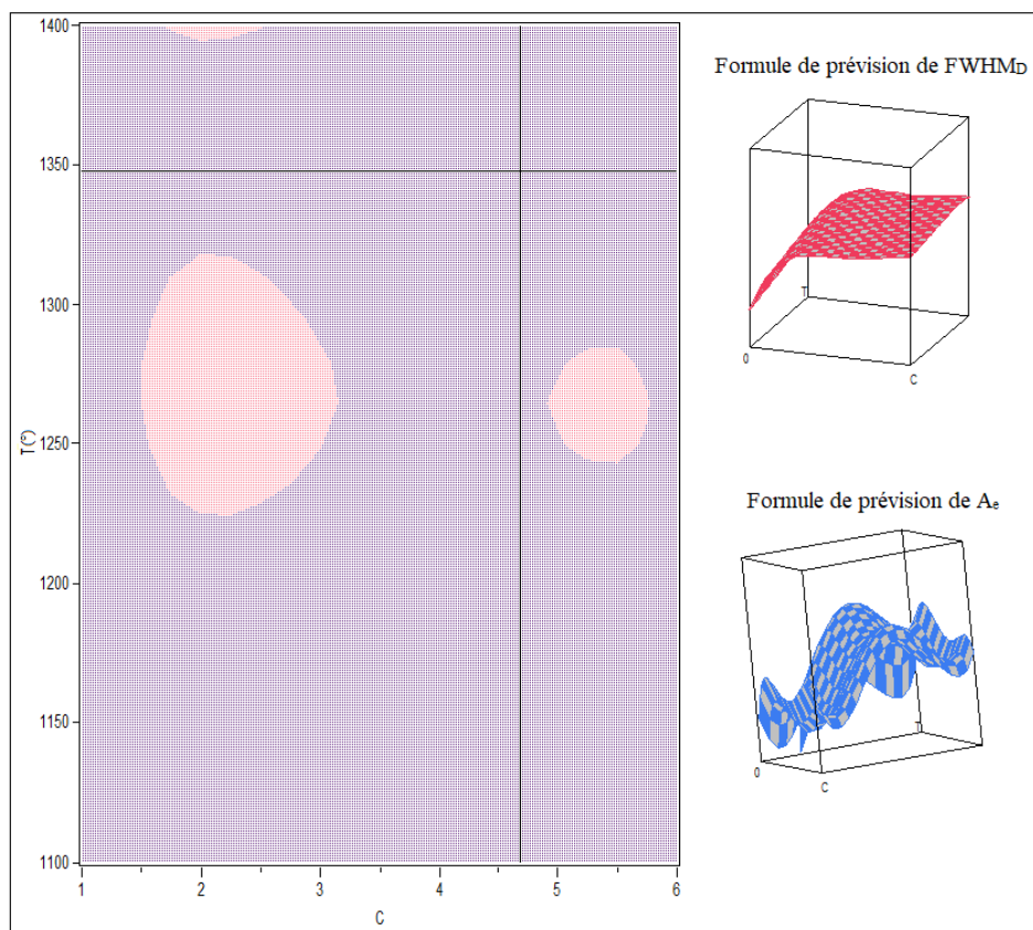
FIGURE III.3.8 – Diagramme d’existence du PyC LRe en considérant les A_e et FWHM_D de la littérature
