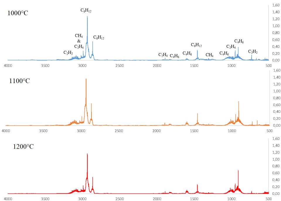
FIGURE III.1.6 – Spectres FTIR des gaz collectés à 1000, 1100 et 1200°C après de 5 min d’élaboration
