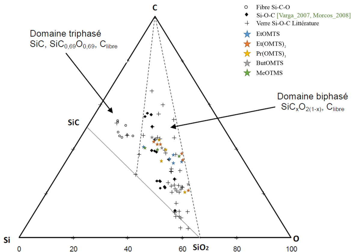
FIGURE IV.2.18 – Compositions chimiques déterminées par EDS reportées sur le diagramme de phase ternaire Si-O-C à la température de 298 K
