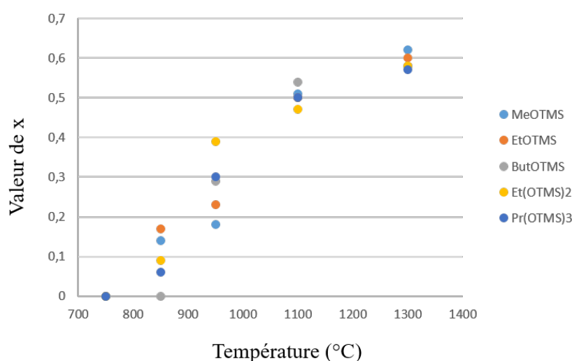
FIGURE IV.3.1 – Évolution de la valeur de x dans la phase \text{SiC}_x\text{O}_{2(1-x)} en fonction de la température du dépôt et du précurseur considéré
