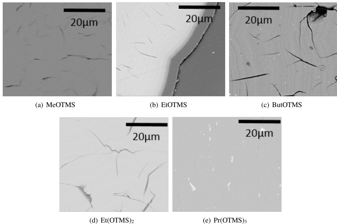
FIGURE IV.2.5 – Clichés MEB montrant les dépôts obtenus à 1300^{\circ}\text{C} pendant 5 min pour chaque précurseur
