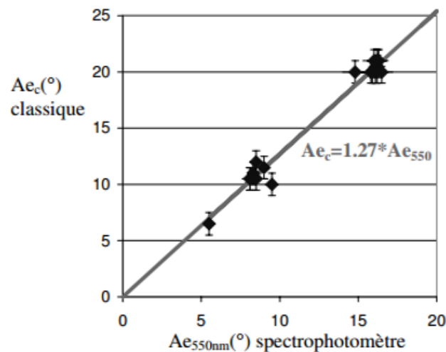
FIGURE II.3.4 – Courbe montrant la fonction Ae_{empirique} = f(Ae_{550\text{ nm}}) obtenue par J.M Vallerot [Vallerot_2004]
