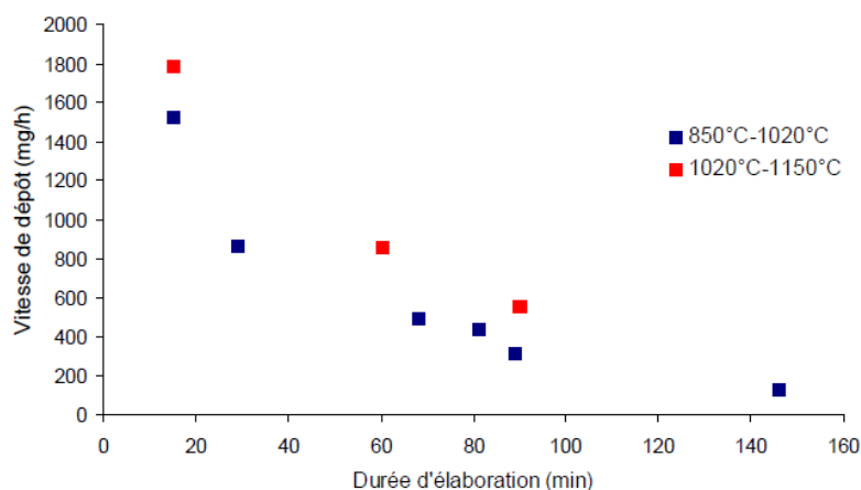
FIGURE I.3.8 – Vitesses de croissance des dépôts (en mg/h) élaborés sur les fibres de carbone en fonction de la durée d'élaboration pour les différentes gammes de températures explorées (850°C-1020°C et 1020°C-1150°C) [Serre_2013]
