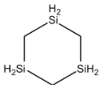
FIGURE IV.3.9 – Schéma moléculaire de 1,3,5 Trisilacyclohexane
