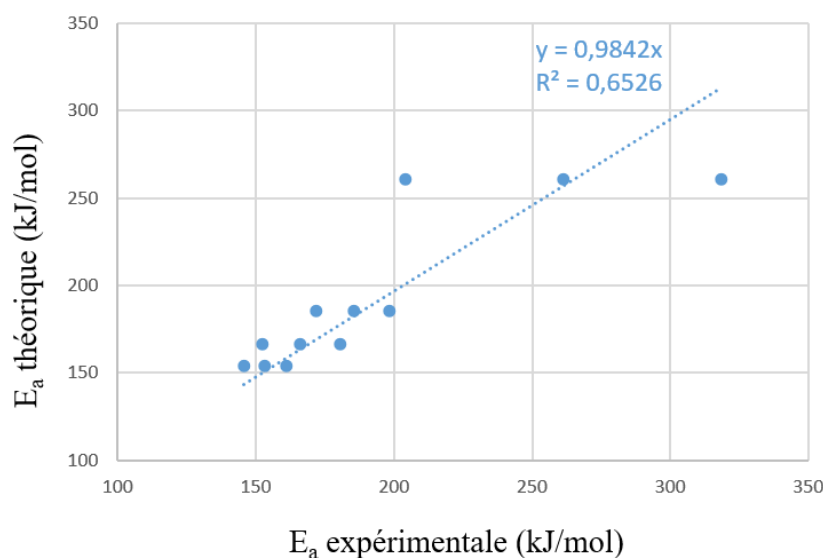
FIGURE III.3.18 – Représentation graphique de l'évolution de l'énergie d'activation mesurée expérimentalement en fonction de l'énergie d'activation modélisée pour le cas des alcools cycliques et leurs homologues linéaires
