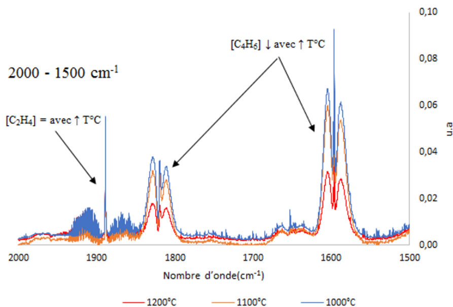
FIGURE III.1.8 – Spectres FTIR montrant l'influence de la température sur la concentration des espèces gazeuses prélevées 1500 et 2000 \text{cm}^{-1} (normalisation par rapport au pic le plus intense du cyclohexane)
