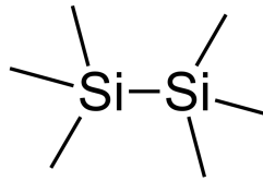
FIGURE I.3.13 – Schématisation de la molécule d'hexaméthylsilane
