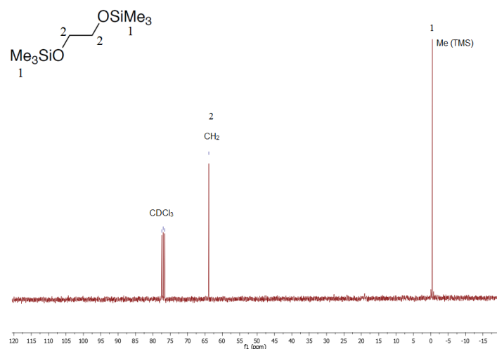
FIGURE IV.1.4 – Spectre RMN ^{13}\text{C} de 1,2-bis(triméthylsiloxy)éthane avec les paramètres du Tableau IV.1.3 entrée 1
