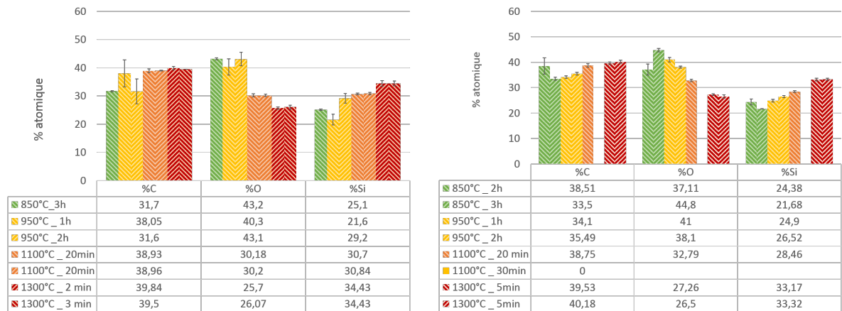
(a) Histogrammes de composition chimique relatifs à MeOTMS (b) Histogrammes de composition chimique relatifs à EtOTMS
