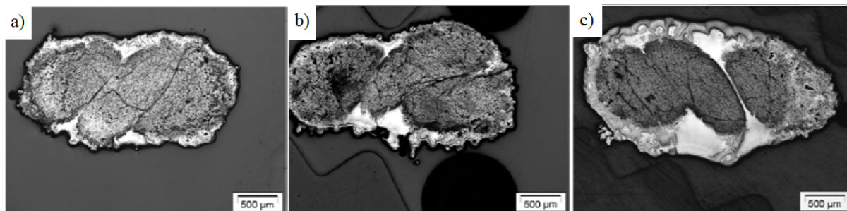
FIGURE I.3.7 – Clichés MO des dépôts élaborés par caléfaction à partir de MTS à 850°C pour une durée de 30 min (a), à 850°C pour une durée de 90 min (b), et à 850°C pour une durée de 150 min (c) [Serre_2013]
