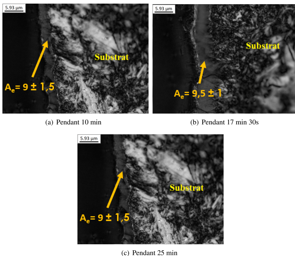
FIGURE III.1.3 – Cartographies d'anisotropie montrant l'influence de la durée de dépôt sur la valeur de l'angle d'extinction ( A_e ) pour les dépôts réalisés à 1100°C
