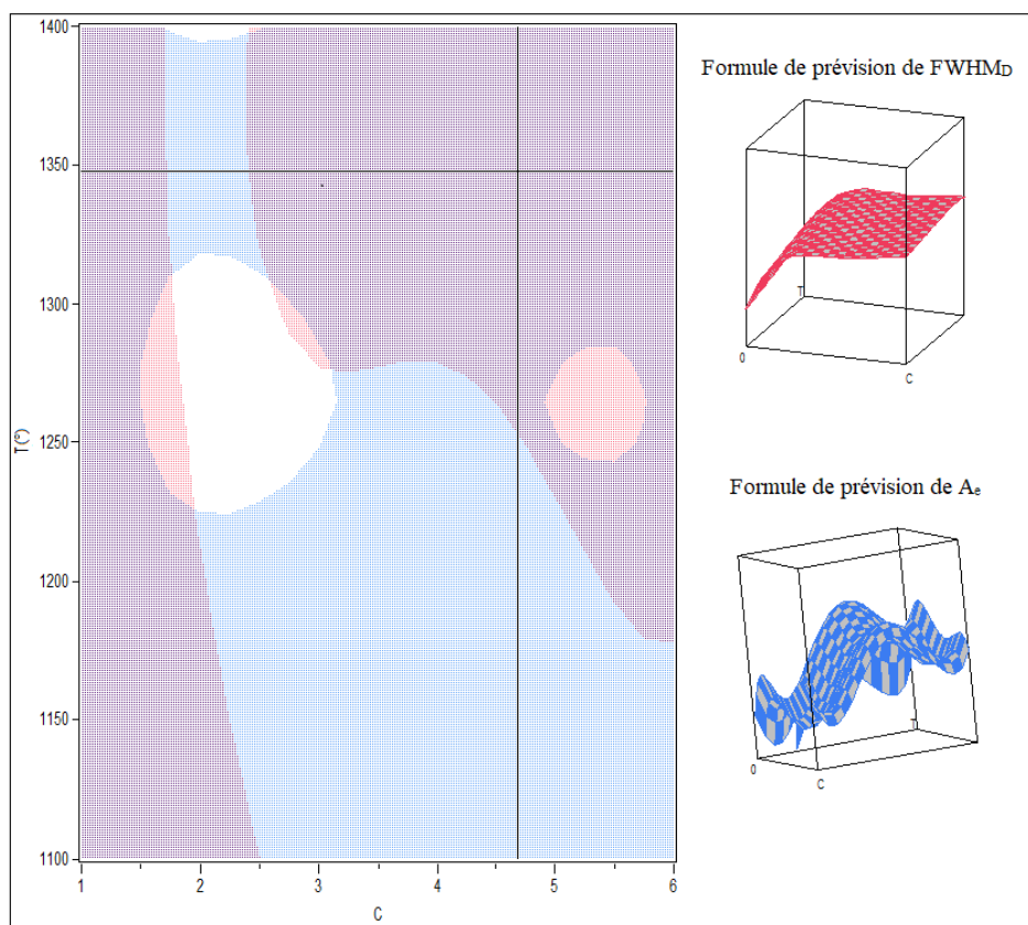
FIGURE III.3.7 – Diagramme d’existence du PyC LR en considérant les A_e et FWHM_D de la littérature
