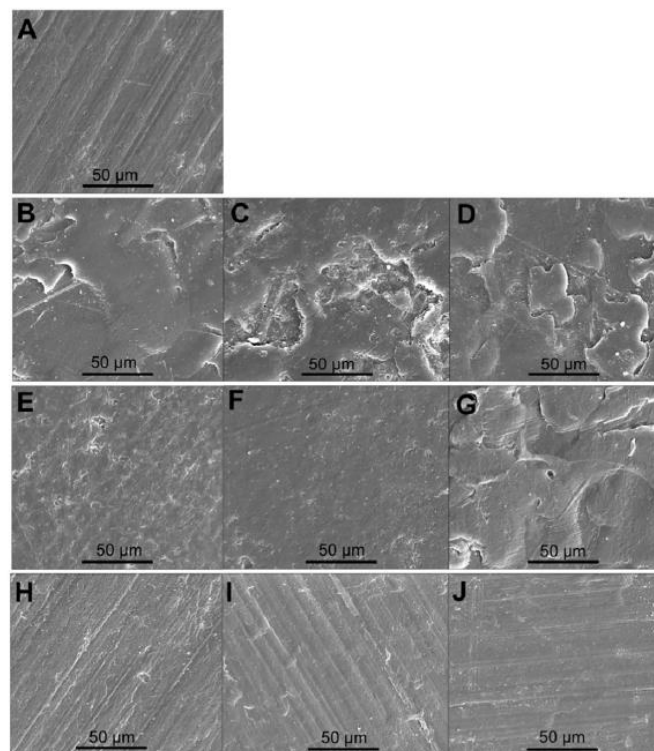
Fig. 4. FESEM Micrographs, mode SE, of the materials at magnification of 2000× (A) PU, (B) STlc1-Ber PU 1 wt%, (C) STlc1-Ber PU 3 wt%, (D) STlc1-Ber PU 5 wt%, (E) STlc2-Ber PU 1 wt%, (F) STlc2-Ber PU 3 wt%, (G) STlc2-Ber PU 5 wt%, (H) NTlc-Ber PU 1 wt%, (I) NTlc-Ber PU 3 wt% and (J) NTlc-Ber PU 5 wt%.
