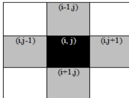
Fig. 51: Von Neumann
