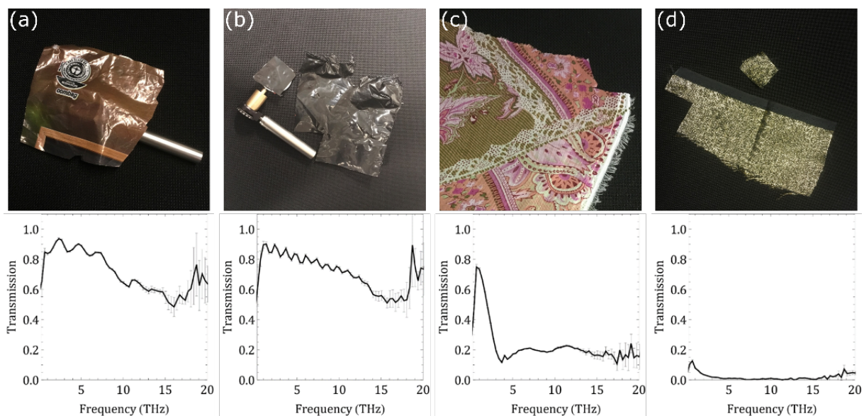
FIGURE 1.8 – Résultats de spectroscopie THz obtenus à DTU. Photographies (haut) et spectres de transmission (bas) de divers matériaux couvrants : (a,b) feuilles de plastique, (c) coton d'épaisseur 1 mm, (d) fibres métalliques. Ces dernières éteignent totalement le signal THz mesurable.
