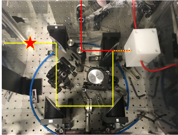
FIGURE 1.11 – Photographie du dispositif ABCD, contenant les quatre miroirs paraboliques, le filtre en silicone, le porte-échantillon et un miroir plan pour orienter le faisceau de la ligne à retard. Le champ à haut voltage est produit entre deux plaques métalliques contenues dans le cube d’isolant blanc. Les filtres et détecteur sont placés à l’arrière du cube. Le plasma est représenté par une étoile rouge, le faisceau THz est représenté en jaune et le faisceau sonde en rouge.
