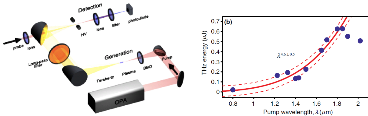
FIGURE 4.2 – (Gauche) Schéma expérimental, comprenant la partie génération et détection des champs THz, utilisé par Clerici et al. (Droite) Énergie THz en fonction de la longueur d'onde laser obtenue par le schéma précédent. Source : Clerici [31].
