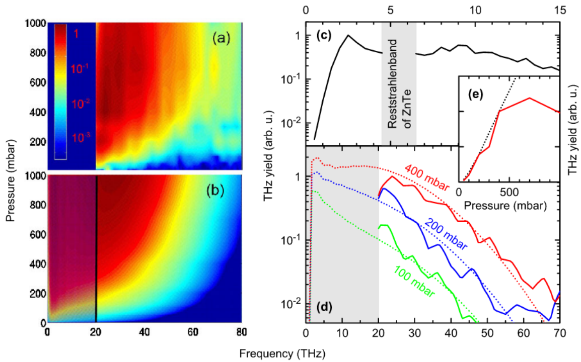
FIGURE 2.20 – (a,b) Spectres expérimentaux (a) et numériques (b) en fonction de la pression du gaz. (c,d) Spectres expérimentaux (traits pleins) et numériques (pointillés) pour différentes pressions. Les zones grisées indiquent des intervalles en fréquence inaccessibles expérimentalement. Source : Babushkin [13].
