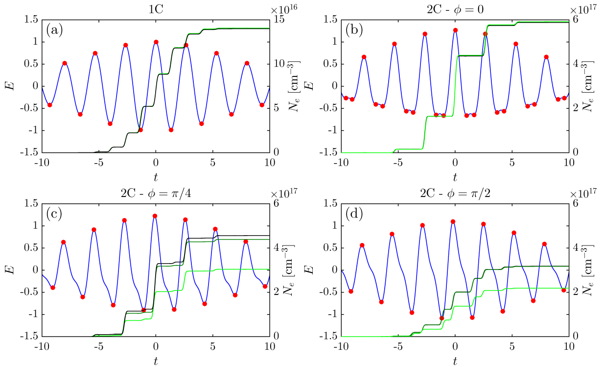
FIGURE B.1 – Détail de champs laser (courbes bleues) à deux couleurs. Les points rouges localisent les extrema du champ laser. Les courbes noires et vertes indiquent la densité électronique calculée numériquement avec le taux d’ionisation QST appliqué à O_2 (courbes noires), ou analytiquement avec ce même taux d’ionisation aux instants t_n calculés avec les équations (4.7) (courbes vert clair) ou (B.8) (courbes vert foncé). (a) Une couleur. (b) Deux couleurs avec une phase relative nulle. (c) Deux couleurs avec une phase relative de \pi/4 . (d) Deux couleurs avec une phase relative de \pi/2 .
