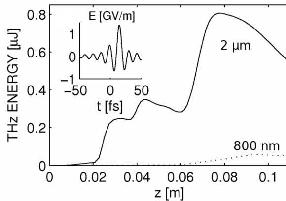
FIGURE 4.1 – Rendement THz d'un filament à deux couleurs avec un FH à 2 \mu\text{m} dans de l'argon à pression p = 6.44 bar (courbe solide). La courbe pointillée correspond à l'énergie THz émise par un filament à 800 nm dans de l'argon à 1 bar, les autres paramètres laser étant inchangés. L'insert montre le champ THz sur l'axe de propagation à z = 7 cm. Source : Bergé [17].
