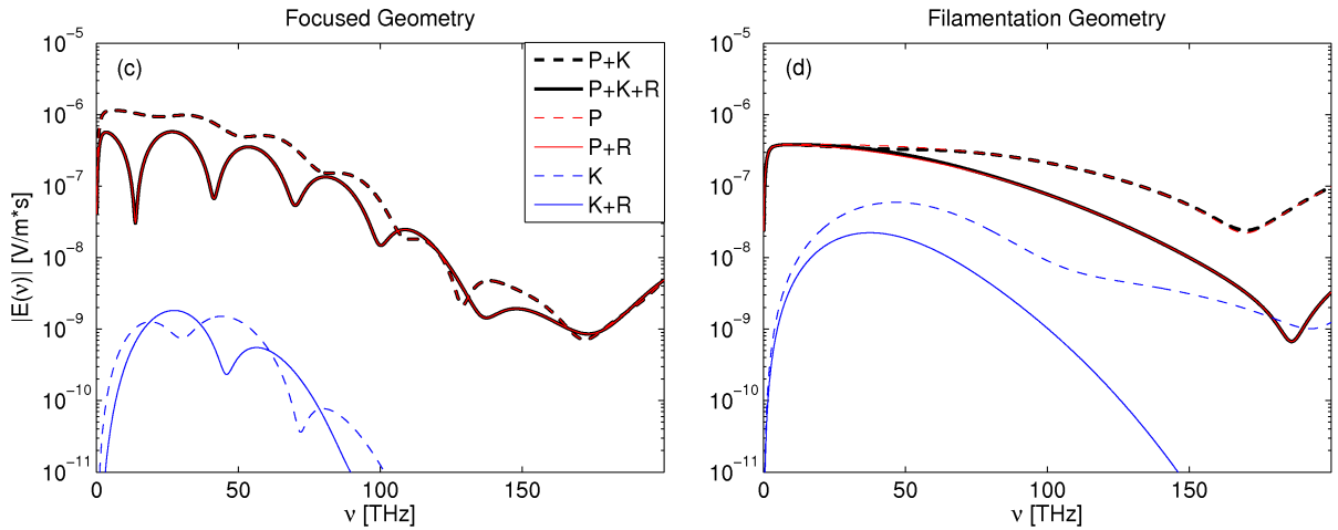
FIGURE 2.17 – (c,d) Spectres THz obtenus en prenant les profils temporels issus de simulations 3D en géométrie (c) focalisée ( f = 2.5 cm, pour une largeur de faisceau initiale de 0.5 mm) ou (d) de filamentation et en appliquant localement les différentes sources issues des photocourants (P), de l'effet Kerr (K) et de l'effet Raman (R). Les impulsions initiales sont à deux couleurs, de durée 60 fs en régime focalisé et 40 fs pour le faisceau collimaté. Les intensités maximales atteintes sont d'environ 100 \text{ TW/cm}^2 .
