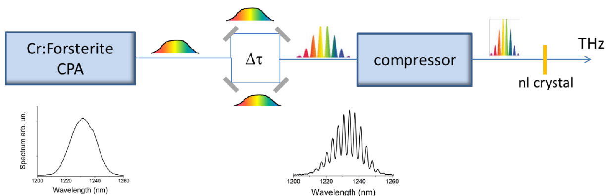
FIGURE 3.2 – Schéma expérimental et spectres associés pour la génération de rayonnement THz par mélange de deux impulsions chirpées dans un cristal organique. L'impulsion laser amplifiée d'un laser CPA Cr:forsterite est divisée et retardée au moyen d'un interféromètre de type Mach Zehnder avant sa recompression sur quelques picosecondes ou moins. La fréquence de battement des deux impulsions chirpées est sélectionnée en faisant varier le retard. Le spectre du fondamental est indiqué en insert, ainsi qu'un exemple de spectre contenant la fréquence de battement ce qui forme un train d'impulsions dans le domaine temporel. Ce train d'impulsions est utilisé pour la production de champs THz à bande étroite à partir d'un cristal organique nonlinéaire. Source : Vicario [101].
