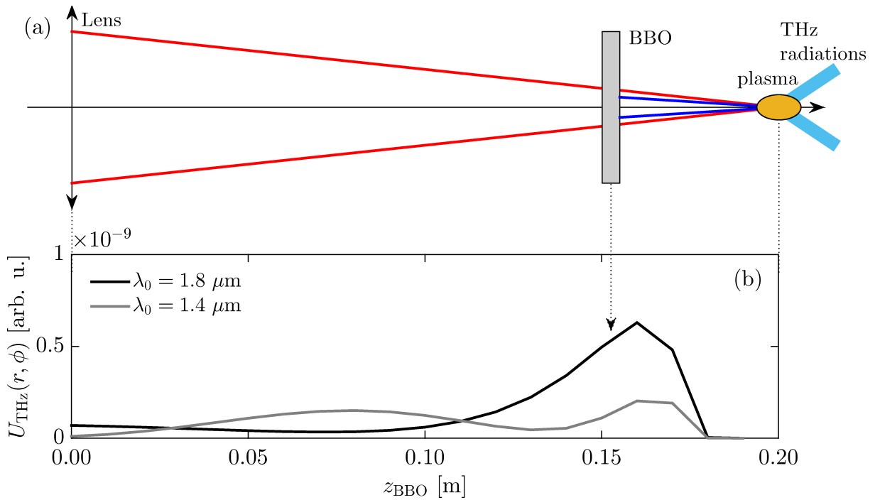
FIGURE 4.23 – (a) Schéma du montage comprenant la lentille de focalisation, le cristal BBO générant le SH et le plasma. (b) Rendements THz donnés par le modèle LC lorsque la position du BBO est variée le long de l’axe de propagation entre la lentille et le plasma, pour deux longueurs d’onde FH.
