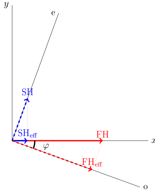
FIGURE 4.22 – Projections de FH et SH sur les axes ordinaires et extraordinaires du cristal \beta -BBO de type I.
