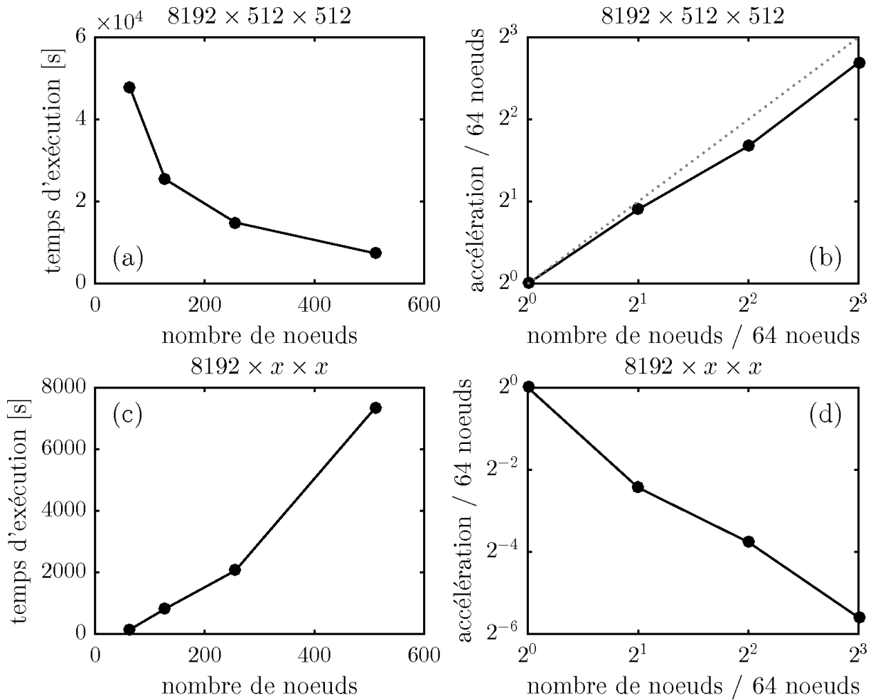
FIGURE C.2 – Rapidité d'exécution du code CUP3D parallélisé hybride MPI/OpenMP sur la machine Occigen. Les simulations testées ont 8192 points en temps, et 64 à 512 points dans chaque dimension spatiale transverse. La référence est prise à 64 nœuds, qui contiennent chacun 24 cœurs. Le nombre de nœuds est ensuite augmenté à 128, 256 et 512. (a) Temps d'exécution des simulations ayant 512 points transverses en fonction du nombre de nœuds et (b) accélération correspondante par rapport au cas à 64 nœuds. (c) Temps d'exécution des simulations ayant un nombre de points transverses identiques au nombre de nœuds utilisés et (d) accélération correspondante par rapport au cas à 64 nœuds.
