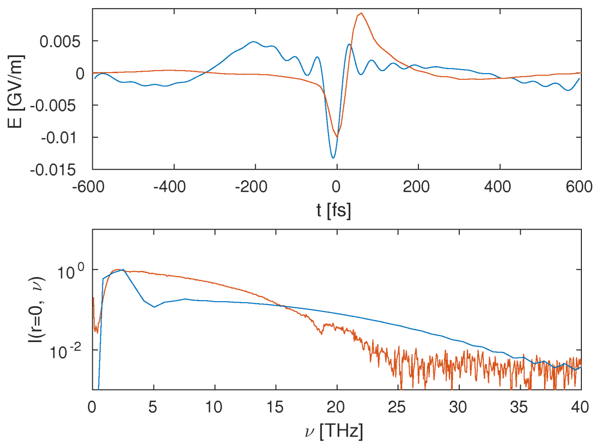
FIGURE 2.22 – Champs (haut) et spectres (bas) THz au point focal obtenus expérimentalement à DTU au cours du projet ALTESSE (courbes rouges), et avec des simulations UPPE 3D (courbes bleues).
