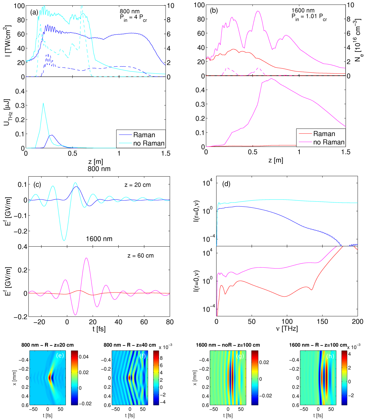
FIGURE 4.6 – Simulations UPPE 3D de filaments à deux couleurs. (a) Haut : Intensité maximum (courbes solides, axe de gauche) et densité électronique maximale (courbes tiretées, axe de droite) d'un filament d'un mètre de long avec des FH à 800 nm (courbes bleues/cyans) et 1600 nm (courbes rouges/magentas) ( r = 3.4\% ). Les courbes claires (cyan/magenta) se réfèrent à une propagation sans nonlinéarité Raman, les courbes foncées (bleu/rouge) l'incluent. Bas : Rendement énergétique THz correspondant, le long de l'axe de propagation ( \nu < 80 THz). (c,d) Champs THz sur l'axe et aux distances de propagation indiquées et intensités spectrales associées proches de la distance d'énergie THz maximum. (e-h) Champs THz dans le plan (x, t) , avec (R) et sans (no R) effet Raman.
