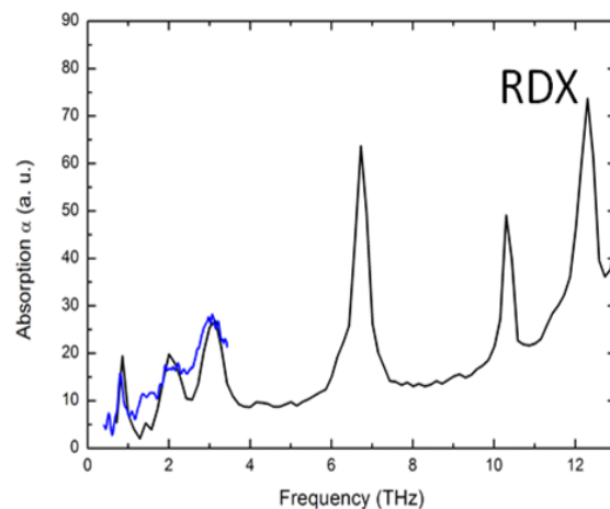
FIGURE 1.5 – Spectres d’absorption d’un explosif, le RDX, obtenus via une antenne photo-conductrice (courbe bleue) ou une source plasma-laser (courbe noire). Source : DTU/ISL.
