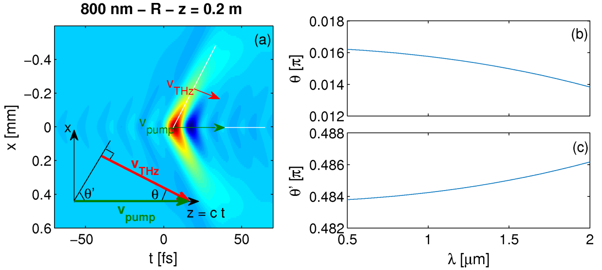
FIGURE 4.7 – (a) Géométrie des vitesses de groupe pour les ondes THz ( v_{\text{THz}} ) et de pompe ( v_{\text{pump}} ). (b) Angle Tcherenkov \theta et (c) angle d'émission associée \theta' = \pi/2 - \theta en fonction de la longueur d'onde de pompe calculés à partir de la dispersion linéaire de l'air (Peck et Reeder [74]).
