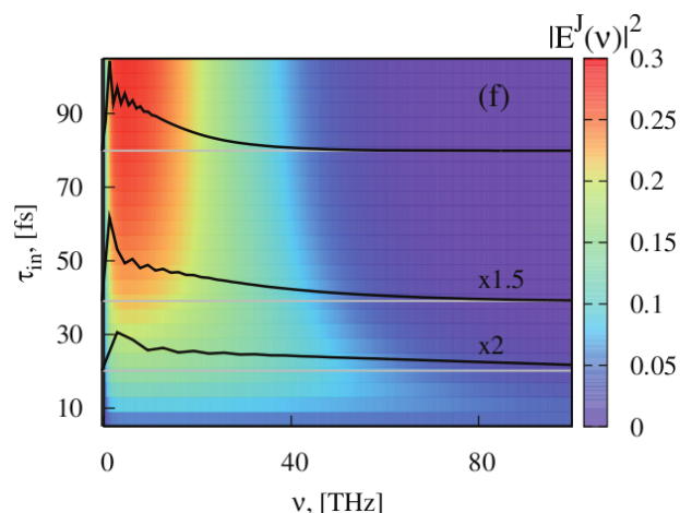
FIGURE 2.16 – Evaluations LC (couleur) et simulations UPPE (courbes noires) d’impulsions laser à deux couleurs en fonction de la durée à mi-hauteur \tau_{\text{in}} à intensité pic fixée. Source : Babushkin [14].
