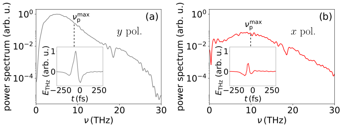
FIGURE 1.20 – Spectres THz expérimentaux obtenus à DTU par la méthode ABCD dans le cas où le champ laser est polarisé suivant (a) le grand axe de l'ellipse (selon y ) ou (b) le petit axe de l'ellipse (selon x ) dessinée par le profil transverse du faisceau laser. Les profils temporels des champs THz sont montrés en insert. La position de la fréquence plasma issue de la densité électronique maximale est indiquée en pointillés.
