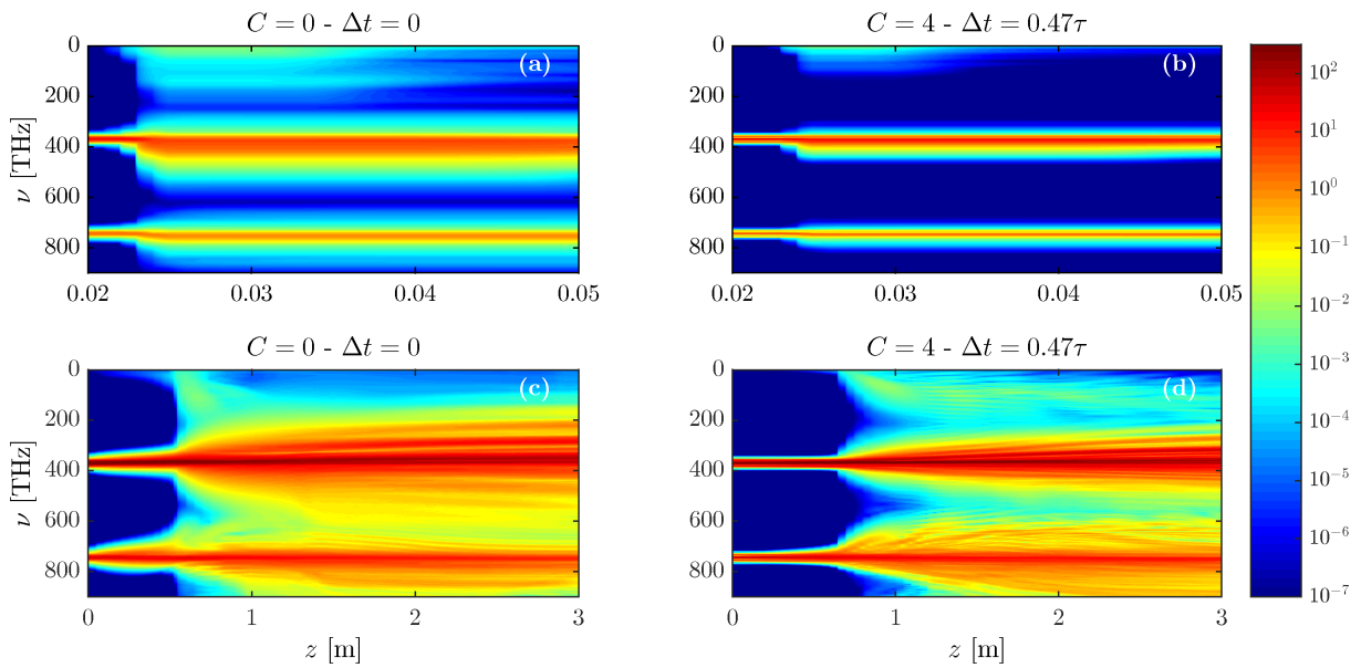
FIGURE 3.8 – Spectres le long de l’axe de propagation pour les impulsions simulées en figure 3.6 avec (a) C = 0, \Delta t = 0 et (b) C = 4, \Delta t = 0.47\tau en régime focalisé. (c,d) Même information avec les configurations de la figure 3.7 en régime de filamentation. L’émission THz aux petites fréquences est amplifiée dans cette dernière configuration.
