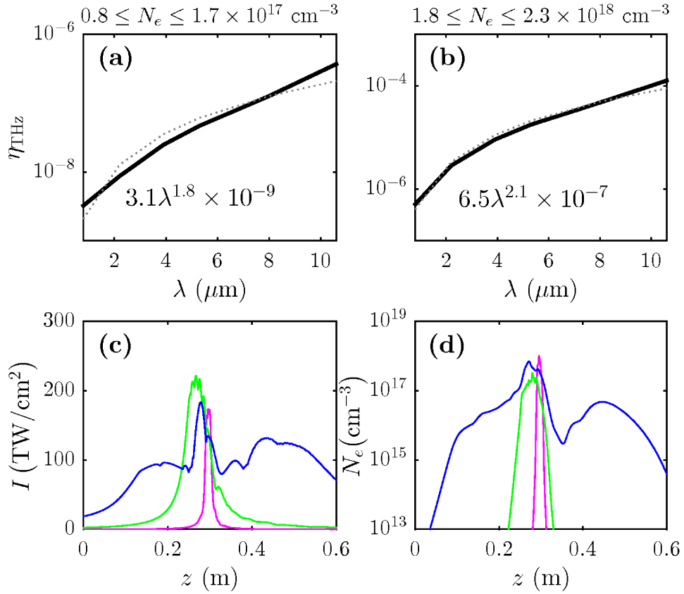
FIGURE 4.10 – (a,b) Efficacité de conversion laser-THz évaluée dans le domaine \nu < 10 THz à partir de l'équation (2.91) avec les deux fluences d'entrée (a) 5 \text{ J/cm}^2 et (b) 10 \text{ J/cm}^2 ( \phi_1 = 0 , \phi_2 = \pi/2 ) générant des densités électroniques variant peu avec FH (voir valeurs indiquées au-dessus). Les courbes grises pointillées sont des fits en \lambda_0^\alpha . (c,d,e) Résultats de simulations UPPE 3D de filaments à deux couleurs du proche au lointain infrarouge. (c) Intensité maximum le long de z utilisant la dispersion HITRAN "hiver" pour des longueurs d'ondes FH de 0.8 (courbe magenta), 3.9 (courbe verte) et 10.6 \mu\text{m} (courbe bleue). (d) Densités électroniques maximales associées.
