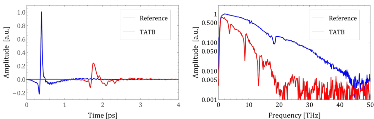
FIGURE 1.12 – (Gauche) Champs THz expérimentaux obtenus par la méthode ABCD sans échantillon (courbe bleue) ou avec un échantillon contenant un explosif (TATB) (courbe rouge). (Droite) Spectres en transmission obtenus par transformée de Fourier des champs.
