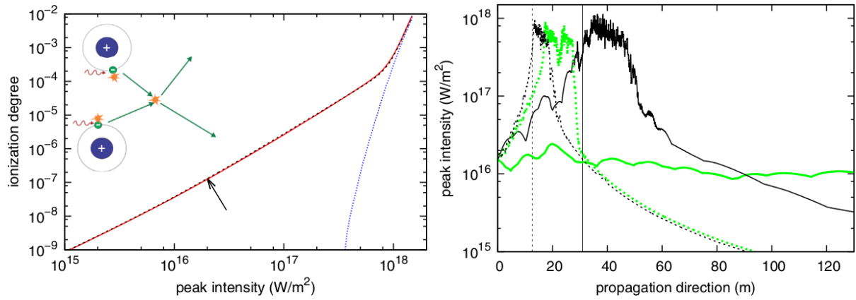
FIGURE 4.16 – (Gauche) Taux d'ionisation résultant de simulations microscopiques complètes (courbe rouge) et résultat du fit associé (courbe noire tiretée, voir équation (4.15)). La courbe pointillée bleue montre le taux QST. L'insert est un schéma de l'ionisation coulombienne à plusieurs corps. Les électrons liés de différents atomes interagissent pour créer une polarisation suffisante libérant des électrons aux basses intensités et aux longueurs d'onde élevées. (Droite) Résultats de simulations UPPE à 4 \mu\text{m} (courbes pointillées) et 10 \mu\text{m} (courbes solides), avec (courbes vertes) et sans MBI (courbes noires). Source : Schuh [86].
