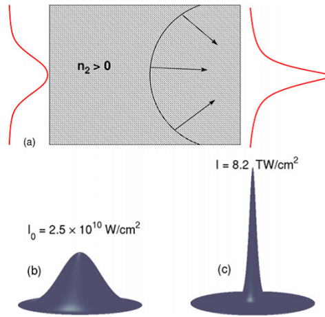
FIGURE 2.2 – (a) Schéma de l’auto-focalisation par effet Kerr. Si un milieu possède un indice non linéaire n_2 positif, alors le faisceau peut s’auto-focaliser. (b,c) Intensités (b) avant et (c) après auto-focalisation. Source : Bergé [18].
