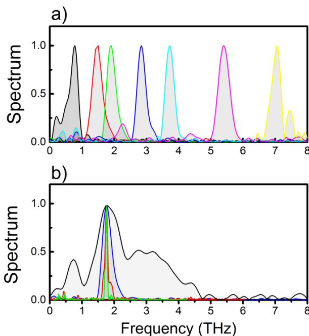
FIGURE 3.3 – Spectres THz obtenus par mélange de deux impulsions chirpées dans un cristal organique (DSTMS). (a) Influence du retard (de l'ordre de la picoseconde pour des impulsions de durée 4 ps) entre les deux impulsions sur la fréquence centrale des spectres. Plus le retard est important, plus la fréquence centrale est élevée. (b) Influence du chirp sur la largeur des spectres THz. Le chirp est varié de telle sorte que la durée des impulsions est augmentée de 120 fs à 20 ps, ce qui permet d'atteindre dans ce dernier cas une fine largeur de bande de 45 GHz. Source : Vicario [101].
