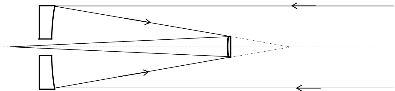
Fig. 32 Schéma optique : télescope Cassegrain
