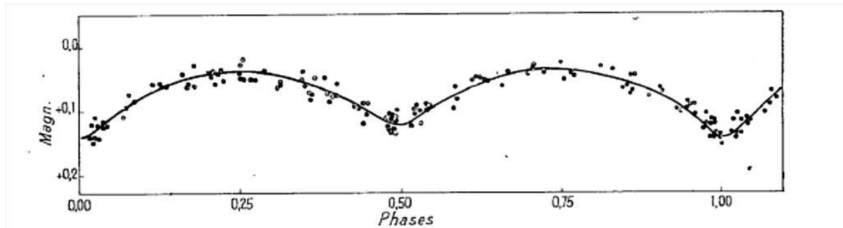
Fig. 49 Courbe de lumière de Omicron Herculis 30
