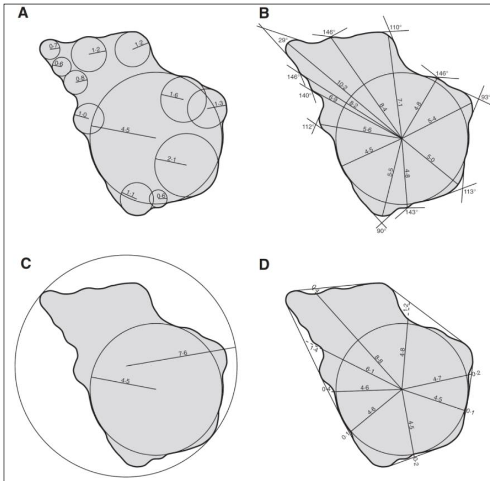
Figure 25. Schémas illustratifs des méthodes de calculs des indices d'émoissé (Blott et Pye, 2008).
