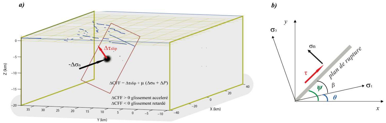
Figure II.8 : a) Représentation de la variation de la contrainte de Coulomb \Delta CFF sur une faille réceptrice, la zone de nucléation est supposée là où la \Delta CFF atteint sa valeur maximale, le rectangle en rouge représente le plan de faille sous forme d'une dislocation rectangulaire , b) Représentation des paramètres géométriques des contraintes principales \sigma_1 et \sigma_3 (modifiée après Stein et al , 1992), \sigma_n et \tau représentent les contraintes normale et tangentielle (ou de cisaillement) selon le critère de Coulomb, \psi représente l'angle entre l'axe des x et le plan de rupture, \theta est l'orientation de la contrainte principale \sigma_1 suivant l'axe des x .
