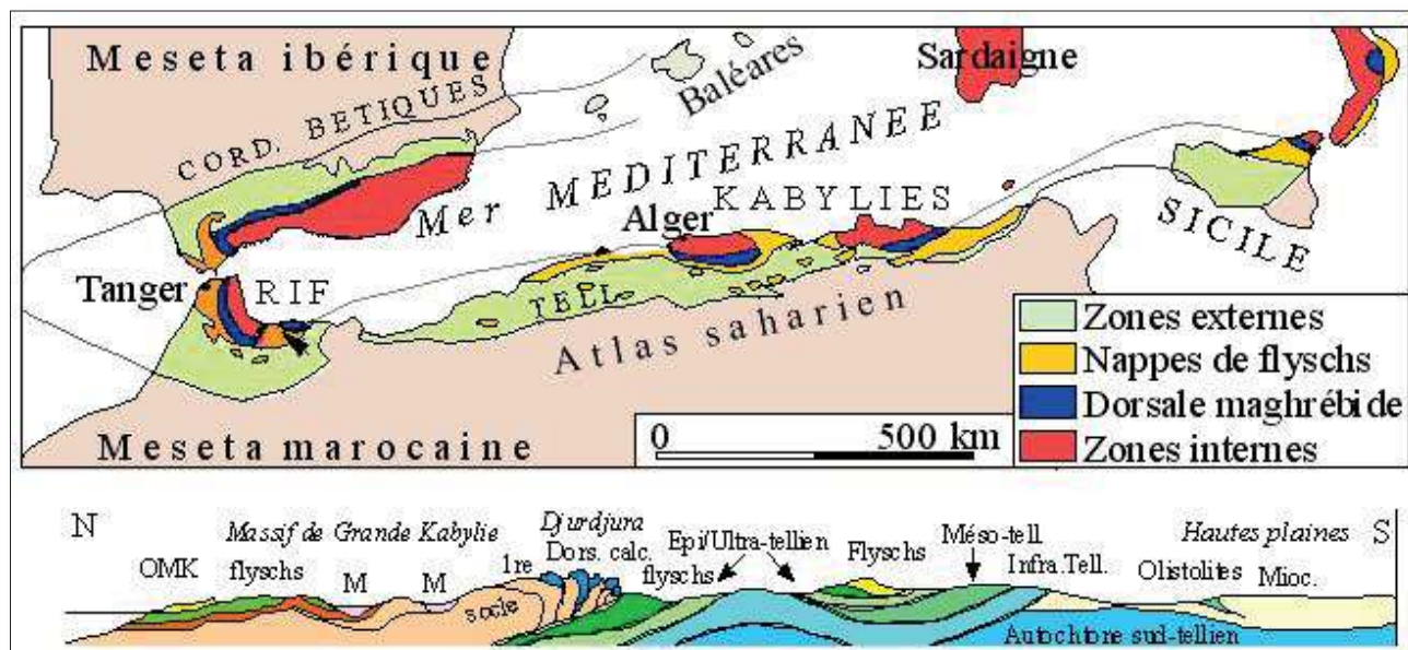
Figure I.2 : Carte structurale schématique de la chaîne des Magrébides montrant la disposition des zones internes et externes et coupe simplifiée sur la transversale de la grande Kabylie, (d'après Delga & Fontboté, 1960).
