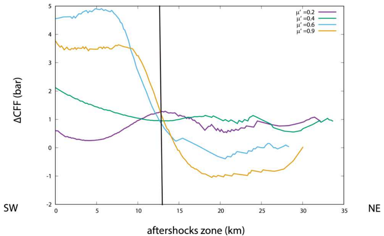
Figure V.7 : relation entre l'occurrence des répliques , variation de la contrainte de Coulomb cumulée et la variation pression des pores associé au séisme d'El Asnam de 1980 : a) localisation des répliques du tremblement de terre d'El Asnam, les fortes répliques ( M > 3.5 ) sont représentées par des cercles en marron, les faibles répliques ( M \leq 3.5 ) sont représentées par des cercles en rouge, le profil de mesure \Delta CFF passant par le maximum des répliques est représentées par une ligne verte, la droite coupant le profil de mesure \Delta CFF représente la situation du segment B de la faille ( voir Figure 9) par rapport aux autres segments, l'étoile en jaune représente l'épicentre du séisme, b) \Delta CFF le long du profil passant
