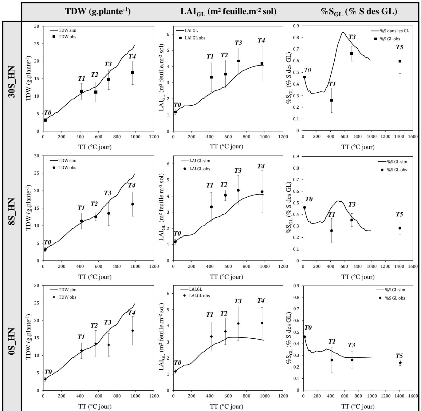
Figure IV.B.3.3 : Observations (symboles) et simulations obtenues avec le modèle SuMoToRI (lignes continues) de la biomasse totale (incluant les FC, TDW, g.plante -1 ), de l'indice de surface foliaire des feuilles vertes (LAI GL , sans dimension, m 2 feuille.m -2 sol) et de la teneur en S des feuilles vertes (%S GL , % de S des GL) pour les 3 conditions d'apport en S en une fois à GS32 (415 °C jour après vernalisation) et non limitantes en N (HN). 0S_HN : 0 U S à GS32, 8S_HN : 8 U S à GS32 et 30S_HN : 30 U S à GS32. Les feuilles vertes (GL) correspondent au pool des feuilles sénescentes, matures et jeunes. Les valeurs observées correspondent à la moyenne ± ET (n = 5, sauf pour 30S_LN où n = 4). T0 : 0 °Cj, T1 : 415 °Cj, T2 : 569 °Cj, T3 : 709 °Cj, T4 : 970 °Cj, T5 : 1412 °Cj. Les valeurs observées des temps T2 et T4 n'étant pas disponibles pour les %S GL , il a été ajouté la valeur observée au temps T5 (1412°Cj) afin de visualiser son évolution future.
