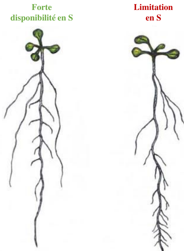
Figure II.27 : Réponses du système racinaire d' Arabidopsis thaliana à une forte disponibilité ou à une limitation en S. Les plantules ont été cultivés dans des milieux riches ou pauvres en S. Une forte limitation en S peut modifier fortement la croissance des racines primaires et latérales, modifiant ainsi l'architecture globale des racines. D'après López-Bucio et al. (2003).
