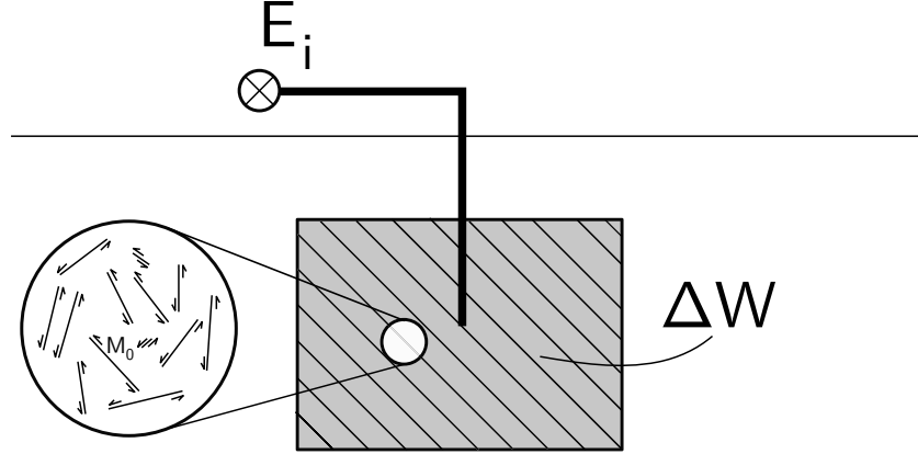
FIGURE 5.1 – Schéma simplifié des transferts d'énergie se produisant au niveau d'un réservoir géothermique au cours d'une injection hydraulique. Le rectangle gris représente notre système (le réservoir géothermique) dans lequel s'effectuent les transformations d'énergie. Il est fourni à ce système une énergie d'injection, E_I , transférée en énergie élastique libérée par rupture, \Delta W . Chacune des fractures engendrées est caractérisée par son moment sismique, M_0 .
