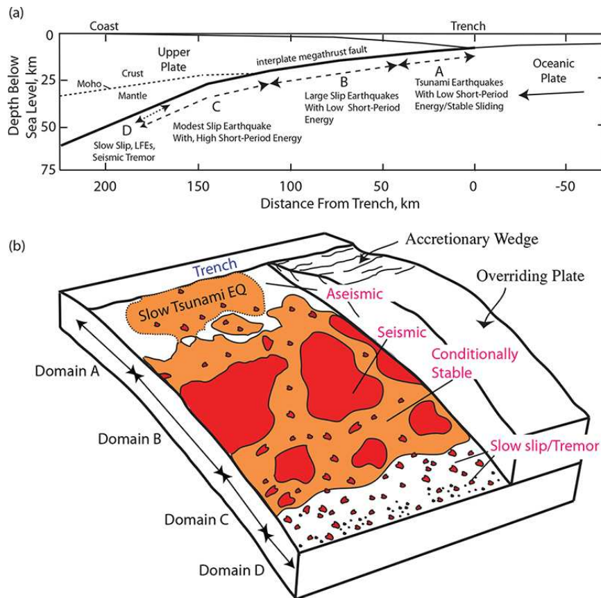
FIGURE 1.9 – (a) Coupe schématique de la zone de subduction située au large de la côte Nord d'Honshu où s'est produit le séisme de Tohoku en 2011. Quatre domaines, A, B, C, et D, sont caractérisés suivant les comportements de rupture observés. Au delà de ces zones, le glissement apparaît stable laissant place à de rares événements ne générant pas de séismes. (b) Modèle schématique de l'environnement frictionnel associé aux zones A, B, C et D définies dans (a). Source : [Lay, 2016].
