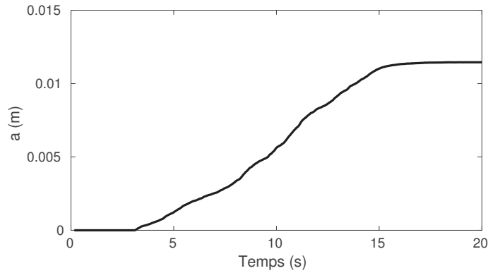
FIGURE 2.20 – Représentation de la position moyenne du front \bar{a}(t) pour la même expérience que celle utilisée pour la représentation des forces et déplacements des Figures 2.3 et 2.4.
