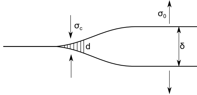
FIGURE 1.10 – Modèle d’une zone de cohésion pour une rupture en mode I. La faille s’ouvre sous la contrainte \sigma_0 . Le déplacement induit par la rupture est noté \delta et la zone de cohésion de longueur d est soumise à une contrainte de cohésion \sigma_c . (d’après [Udías et al., 2014])
