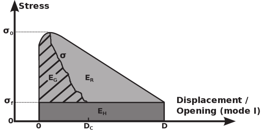
FIGURE 1.6 – Budget énergétique par unité de surface d'un séisme ou d'une fracture : E_R correspond à l'énergie radiée, E_G , à l'énergie de fracture et E_H , à l'énergie de friction. A l'initiation du séisme, la contrainte sur la faille, \sigma_0 , diminue jusqu'à une valeur constante, \sigma_f . (modifié d'après [Kanamori and Brodsky, 2004])
