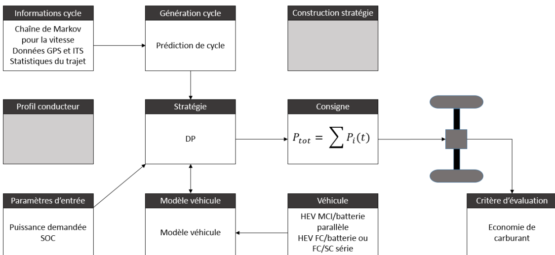
FIGURE 1.40 – Gestion énergétique de Johannesson et al. [54]
