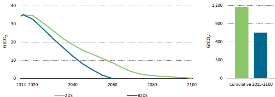
FIGURE 2 – Objectif d'émissions de CO 2 annuelles (à gauche) et cumulées (à droite) pour le siècle actuel
