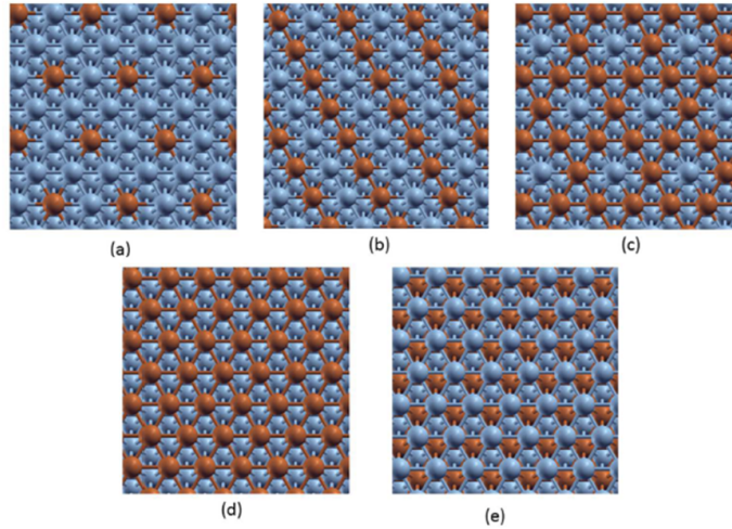
Figure B.1: vues de dessus des cellules utilisées pour représenter les surfaces bimétalliques de NiM. Composition de la couche supérieure: (a) 25% de M et 75% de Ni; (b) 50% de M et 50% de Ni; (c) 75% de M et 25% de Ni; (d) 100% M. Le système (e) a une couche supérieure complète de Ni et une deuxième couche de M. Les sphères grises et oranges représentent respectivement les atomes de Ni et de M.
