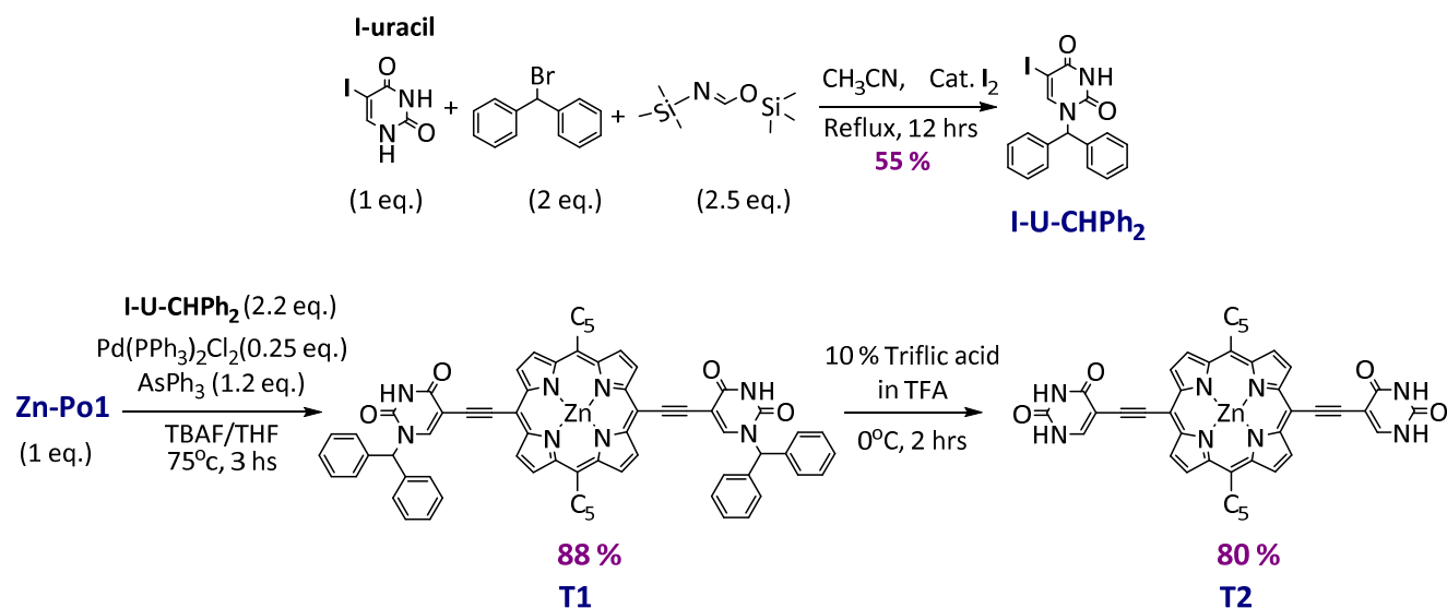
Figure 7: Synthèse de T1 and T2 .
