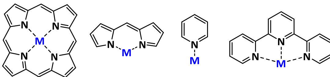
Figure 1: Structure de ligands coordonnants: porphyrine, dipyrriine, pyridine, terpyridine (de gauche à droite).
