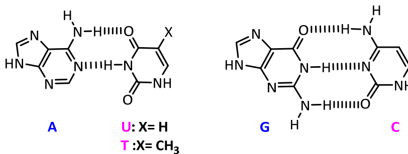
Figure 3: les appariements dits de Watson-Crick : A-T et G-C
