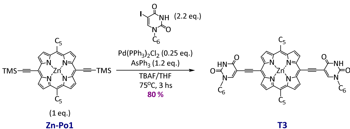
Figure 8: Synthèse de T3 .
