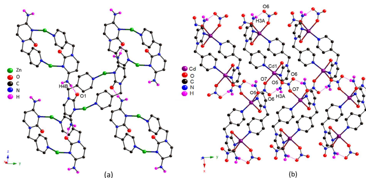
Figure 19: Une portion de la structure obtenue à partir de C-Py en présence de (a) \text{Zn(II)} (les anions ont été omis par souci de clarté) et (b) \text{Cd(II)}
