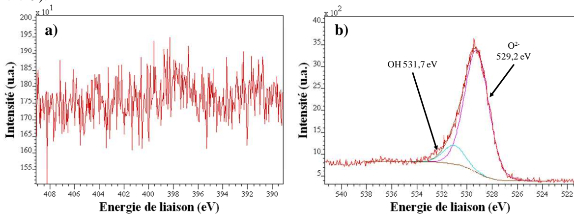
Figure II.1.19 : Spectres XPS (a) de l'azote et (b) de l'oxygène présents en surface des nanoparticules
