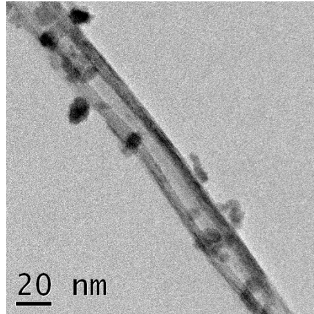
Figure 6 : Cliché MET de nanotubes d'oxyde de titane décorés par des USPIO
