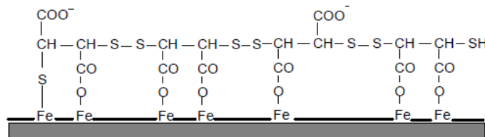
Figure II.2.16 : Représentation schématique des ponts disulfures formés à la surface de particules de magnétite modifiées en surface par du DMSA d'après (Roger et al. 1999).
