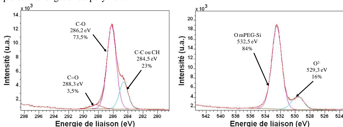
Spectres XPS et désomation avec leurs proportions relatives du carbone et de l'oxygène de nanoparticules avec du mPEG 2000 -Si
