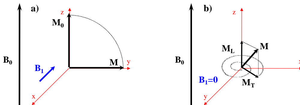
Figure I.2.3 : (a) Déplacement du champ M_0 en M perpendiculairement à B_0 sous l'action d'un champ magnétique radiofréquence B_1 . (b) A l'arrêt de B_1 , le champ M va rejoindre sa position d'équilibre en retrouvant sa composante longitudinale M_L maximale et sa composante transversale M_T nulle.
