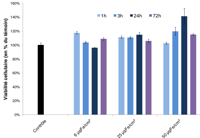
Figure III.1.6 : Mesure de la viabilité cellulaire des macrophages de type RAW à différentes concentrations de nanoparticules d'oxyde de fer pour quatre temps d'incubation. Les résultats sont donnés en pourcentage par rapport à la viabilité du contrôle (n = 6 sur deux expériences indépendantes).
