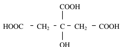
Figure II.2.2 : Formule semi-développée de l'acide citrique
