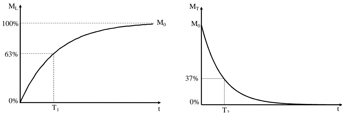
Figure I.2.4 : (a) Evolution en fonction du temps de l'aimantation longitudinale ( M_L ) après une impulsion B_1 (b) Evolution en fonction du temps de l'aimantation transversale ( M_T ) après une impulsion B_1 . Les temps T_1 et T_2 sont respectivement le temps que va mettre M_L à atteindre 63% de sa valeur à l'équilibre et le temps que M_T va mettre à diminuer jusqu'à 37% de sa valeur maximale sous excitation.
