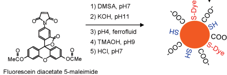
Figure II.2.15 : Procédé de couplage d'un fluorophore par le biais des fonctions thiols à des nanoparticules d'oxyde de fer d'après (Bertorelle et al. 2006).
