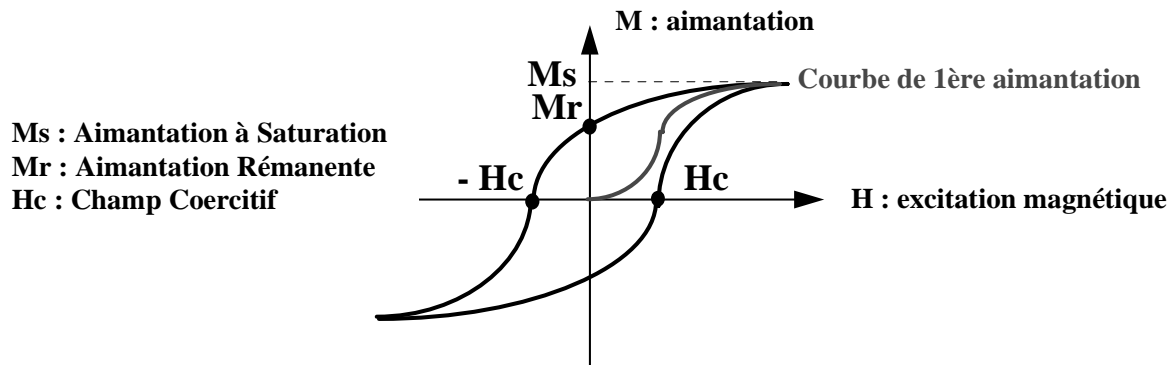
Cycle d'hystérésis d'un composé ferri ou ferromagnétique.
