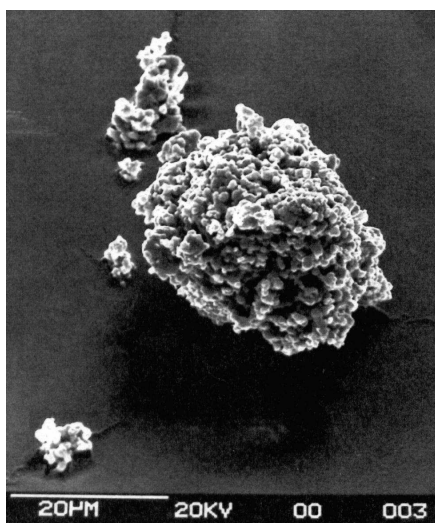
Cliché MEB d'un grain de BaTiO 3 : agrégat de 30 µm environ
