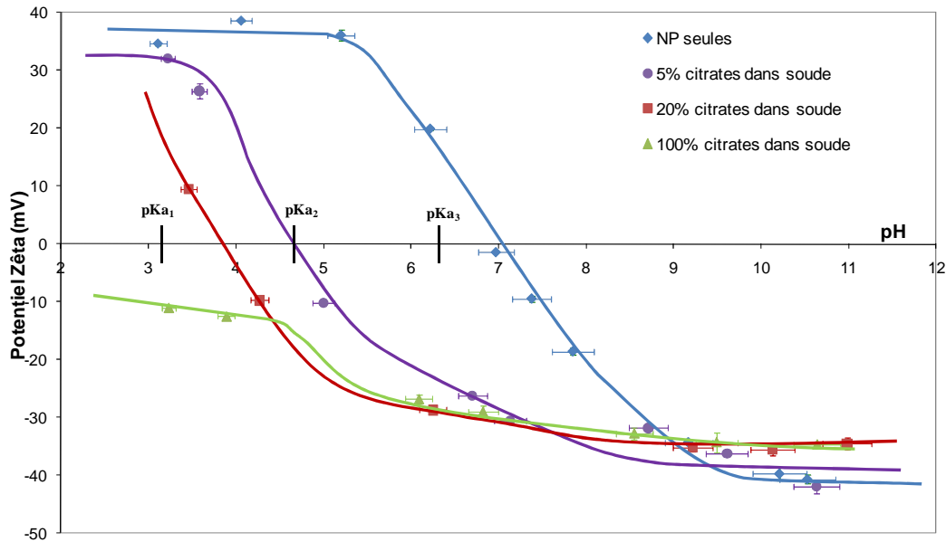
Figure II.2.10 : Potentiels Zêta en fonction du pH dans NaCl 10^{-2}M des nanoparticules de magnétite de référence et modifiées avec 5%, 20% et 100% d'acide citrique préparés dans la soude.
