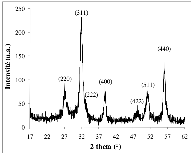
Figure II.1.8 : Diffractogramme des nanoparticules synthétisées par la méthode Massart, \lambda = 1,3922 \text{ \AA}
