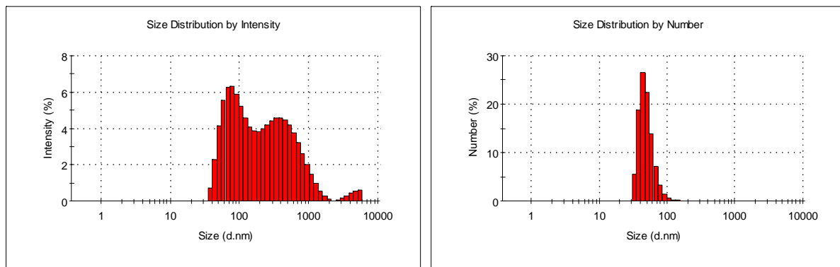
Figure II.1.11 : A gauche taille en intensité des nanoparticules par DLS; à droite taille en nombre. Les diamètres au-delà de 2 \mu\text{m} sont des pollutions non éliminées car les suspensions n'ont pas été filtrées avant analyse.
