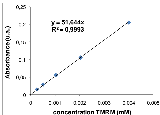
Figure II.2.43 : Courbe de calibration pour différentes concentrations de l'absorbance de la rhodamine maléimide en fonction de sa concentration en mM.
