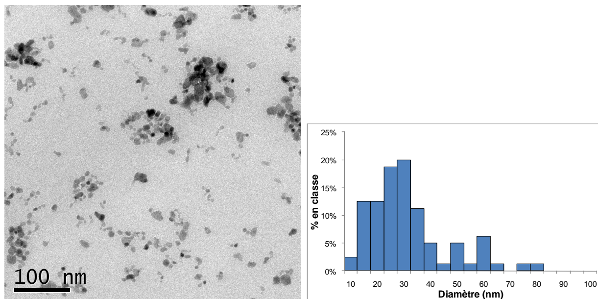
Figure II.2.36 : Cliché MET et comptage MET sur une centaine d'agrégats de nanoparticules greffées par du mPEG 2000 -Si et fonctionnalisées par de la Rhodamine-APTES (NP 0,5RITC )
