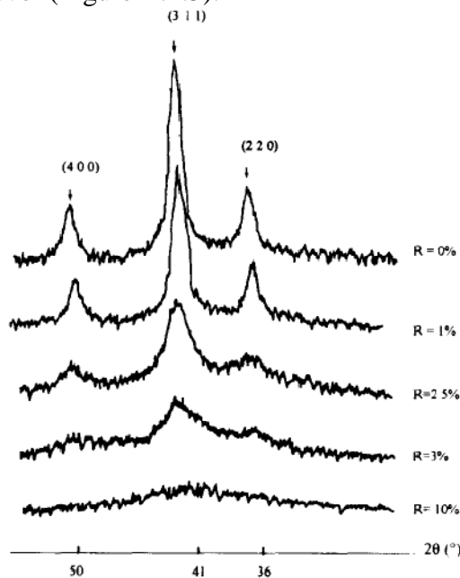
Figure II.2.5 : Diffractogrammes des rayons X de poudre de magnétite synthétisées avec des ratios de citrates R différents ( \lambda = 1,7905 \text{ \AA} ) d'après (Bee et al. 1995)
