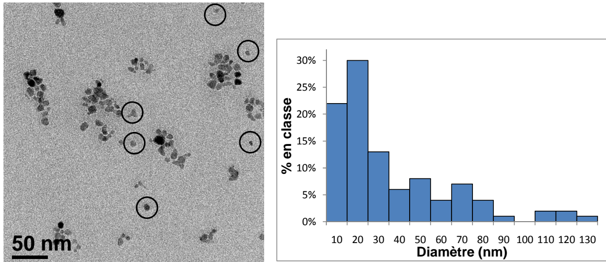
Figure II.1.14 : Cliché MET d'agrégats de magnétite optimisés et comptage des agrégats de magnétite optimisés. Les cercles représentent particules élémentaires présentes dans la suspension.
