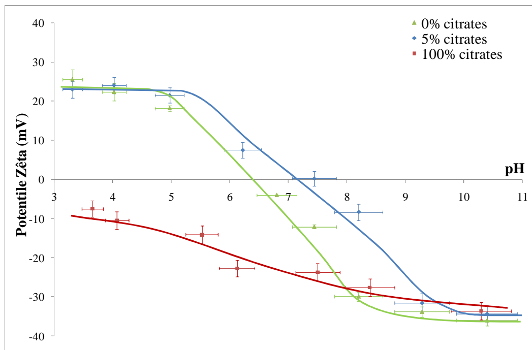
Figure II.3.8 : Courbes de potentiels Zêta en fonction du pH à 10^{-2}M de NaCl pour les nanoparticules de magnétite synthétisées en continu avec respectivement : ▲ 0% de citrates ; ● 5% de citrates et ■ 100% de citrates.
