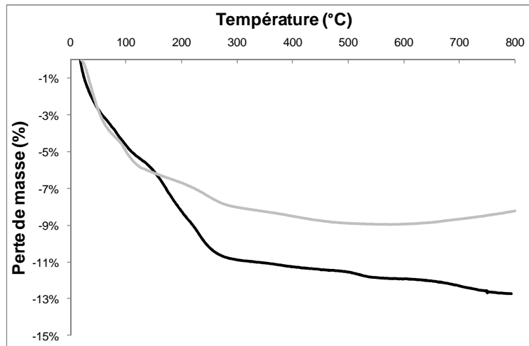
Figure II.2.7 : Analyse thermogravimétrique des nanoparticules citratées à 5% dans la soude (noir) et des nanoparticules nues (gris). Les mesures ont été effectuées sous flux de N_2/O_2 (0,12/0,04 mL.min -1 ) avec une rampe de montée en température de 2°C.min -1 . La dérive de la balance a été corrigée.
