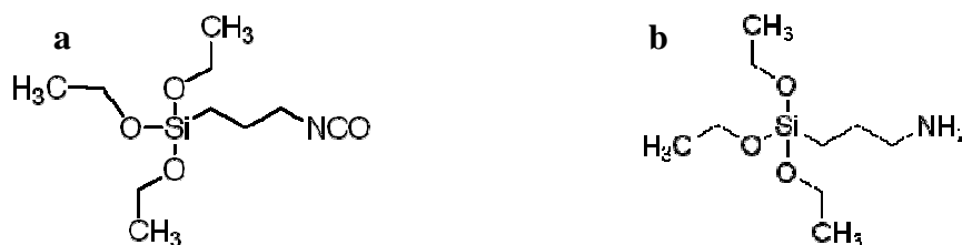
Figure II.2.23 : Formules semi-développées de l'ICPTES (a) et de l'APTES (b)
