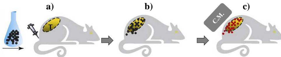
Figure I.1.7 : Mécanisme d'hyperthermie à base de nanoparticules d'oxyde de fer (cercles gris) chez la souris. (a) Les oxydes de fer sont injectés à la souris. (b) Ces nanoparticules sont concentrées dans l'organe ciblé. (c) Un champ magnétique (C.M.) est appliqué et échauffe les nanoparticules (cercles rouges) d'après (Corchero et al. 2009).
