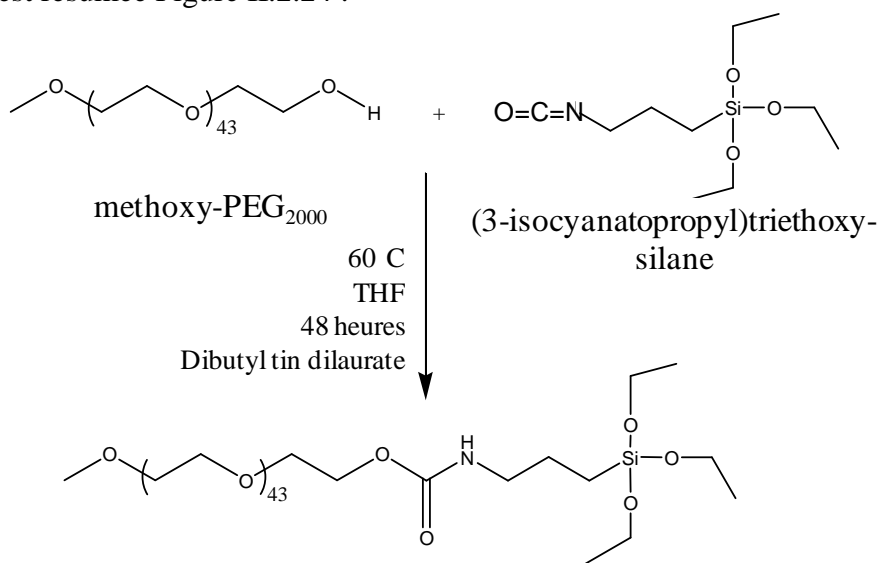
Figure II.2.24 : Réaction de l'ICPTES sur le mPEG 2000 pour obtenir du mPEG 2000 silanisé
