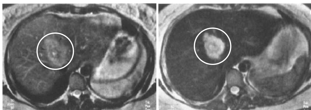
Figure I.2.10 : Détection de tumeurs hépatiques (cercles blancs) chez l'homme en IRM à 1 T. (a) Image en pondération T_2 acquise sans utilisation d'USPIO (b) Image en pondération T_2 acquise avec utilisation d'USPIO (Sinerem®) d'après (Mergo et al. 1998)
