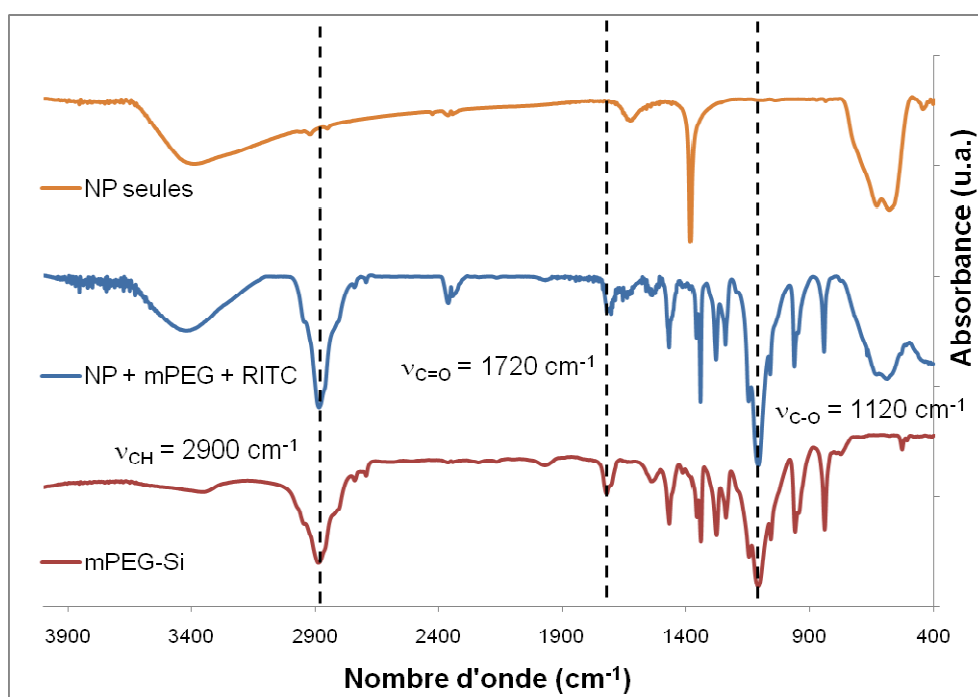
Figure II.2.37 : Analyses infrarouges de la magnétite seule, modifiée avec le mPEG-Si et de la rhodamine et du mPEG-Si seul. Les mesures ont été effectuées dans des pastilles de KBr.
