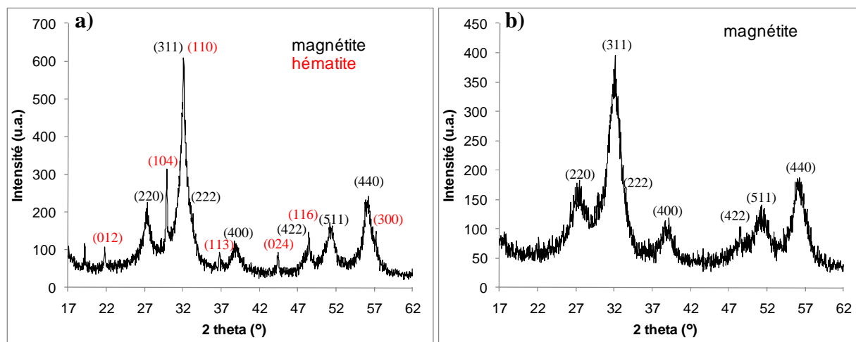
Figure II.3.6 : Diffractogrammes des rayons X de nanoparticules synthétisées en voie hydrothermale continue avec respectivement un ratio molaire en citrates par rapport au fer de, (a) 5% et (b) 100% ( \lambda = 1,3922 \text{ \AA} ).
