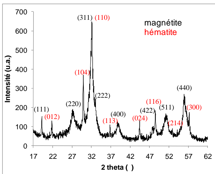
Figure II.3.4 : Diffractogramme des nanoparticules synthétisées par voie hydrothermale à 150^\circ\text{C} , 25 \text{ MPa} et 60 \text{ mL}\cdot\text{min}^{-1} ( \lambda = 1,3922 \text{ \AA} ).
