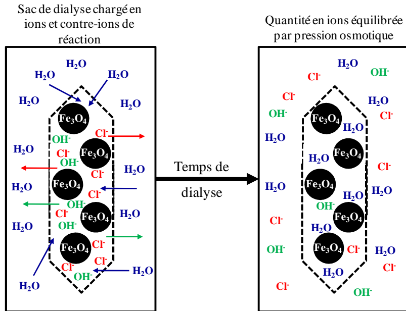
Figure II.1.4 : Schéma de dialyse. Les ions de la solution après synthèse vont être éliminés par les pores de la membrane de dialyse et de l'eau va rentrer dans le sac de dialyse. Les concentrations en ions des solutions à l'intérieur et à l'extérieur de la membrane vont s'équilibrer. Plusieurs changements d'eau de dialyse sont nécessaires pour éliminer la majorité des contre-ions de réaction.
