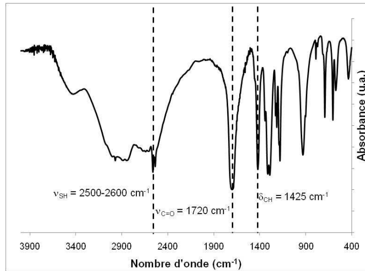
Figure II.2.14 : Analyse infrarouge du DMSA sous forme de poudre préparée dans des pastilles de KBr.
