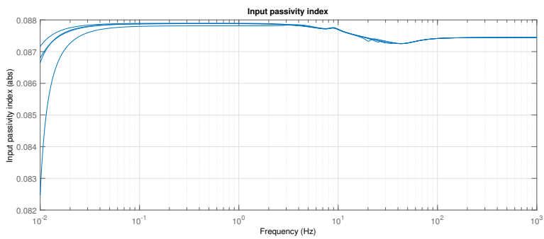
FIGURE 3.31 – Indice de passivité en entrée de \mathcal{Z}_{r_h}^{cl}
