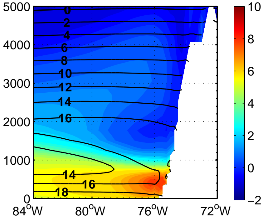
b) WRF
