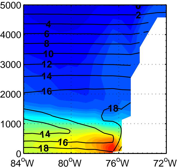
a) ERA-Interim
