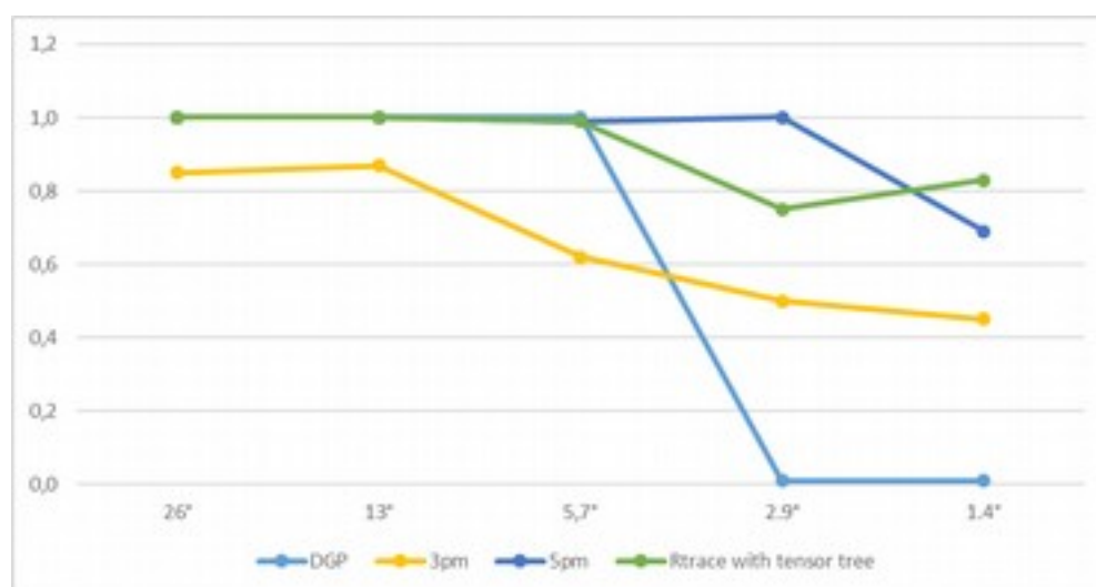
Figure 77: Comparaison des différents DGP en fonction de l'amplitude de l'angle de pic.
