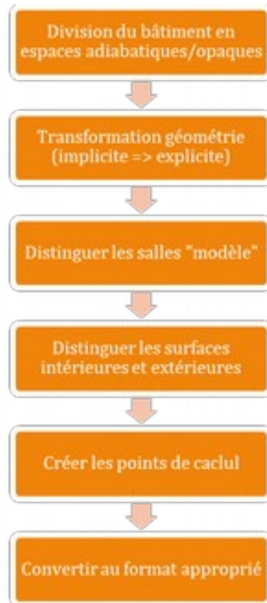
Figure 74: Méthodologie de transformation d'un BIM en format IFC en format compatible avec les logiciels de simulation.
