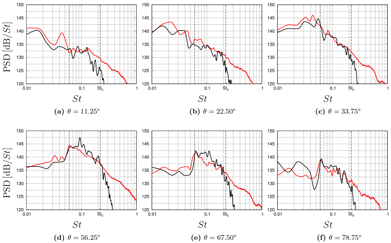
Figure 5.14: PSD des signaux de pression sur l'antenne AZ1 aux angles 11.25 \leq \theta \leq 78.75 . — : données expérimentales avec \Delta St = 5 \times 10^{-3} ; — : simulation NS-Euler avec \Delta St = 8 \times 10^{-3} ; --- : St = 0.06 et fréquence de coupure théorique St_c = 0.23 .
