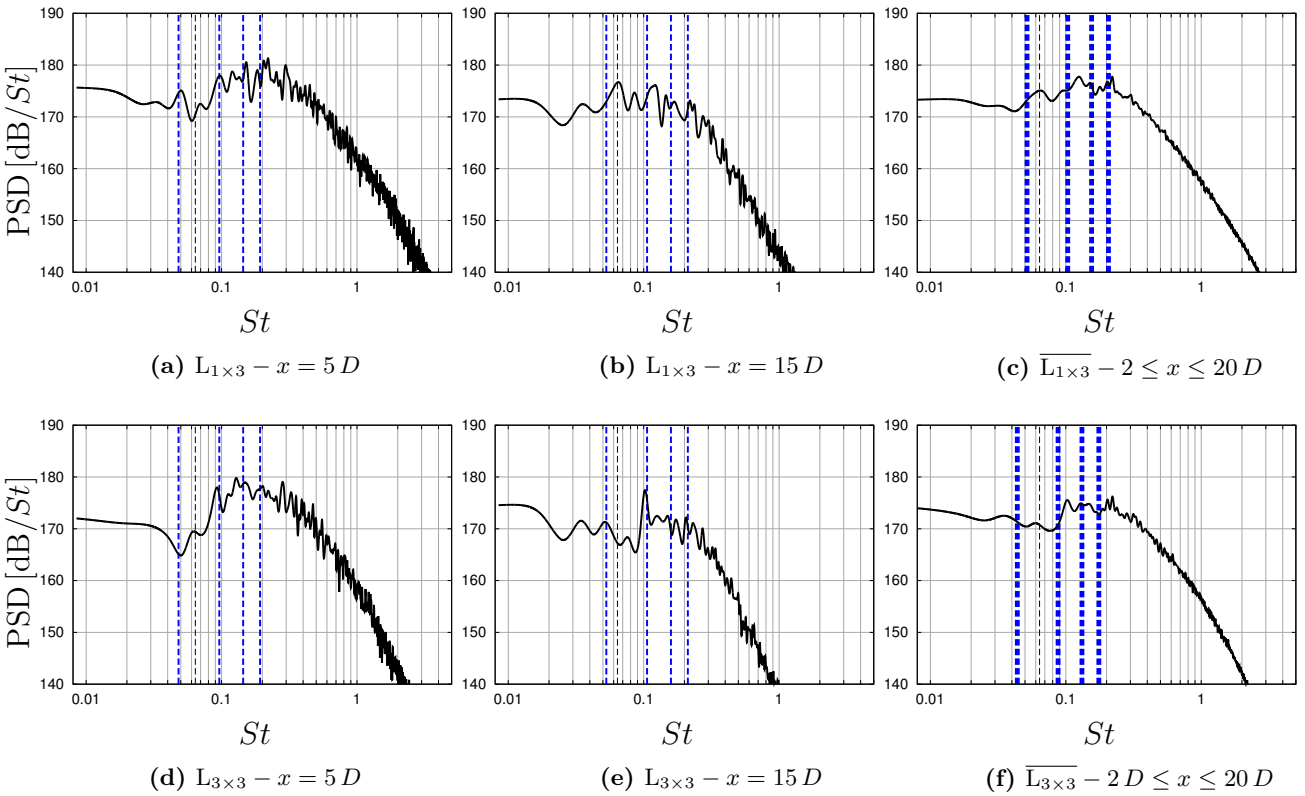
Figure 5.20: PSD de la pression dans le carneau sur les antennes L_{1 \times 3} et L_{3 \times 3} aux positions x = 5D , 15D et PSD moyenne sur toute la longueur 2D \leq x \leq 20D . — : simulation NS-Euler avec \Delta St = 8 \times 10^{-3} ; --- : modes transversaux m \in [1, 2, 3, 4] de la section carrée; --- : St = 0.064 .
