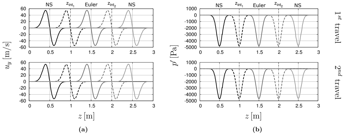
Figure 3.12: profils longitudinaux de (3.12a) vitesse et (3.12b) pression du tourbillon isentropique convecté aux instants \text{—} : t = 0 ms ; \text{- - -} : t = 5 ms ; \text{—} : t = 10 ms ; \text{- - -} : t = 15 ms ; \text{—} : t = 20 ms.
