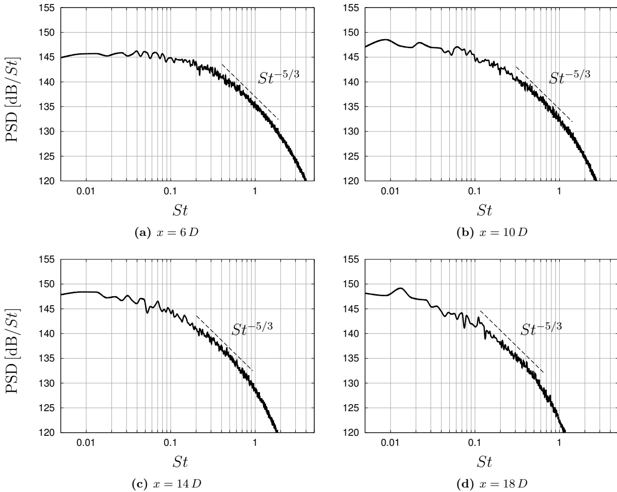
Figure 4.17: PSD de la vitesse axiale dans la couche de cisaillement sur l'antenne A aux positions (4.17a) x^* = 6 , (4.17b) x^* = 10 , (4.17c) x^* = 14 et (4.17d) x^* = 18 . — : simulation NS-Euler avec \Delta St = 4.5 \times 10^{-3} ; --- : pente en St^{-5/3} de la loi de Kolmogorov.
