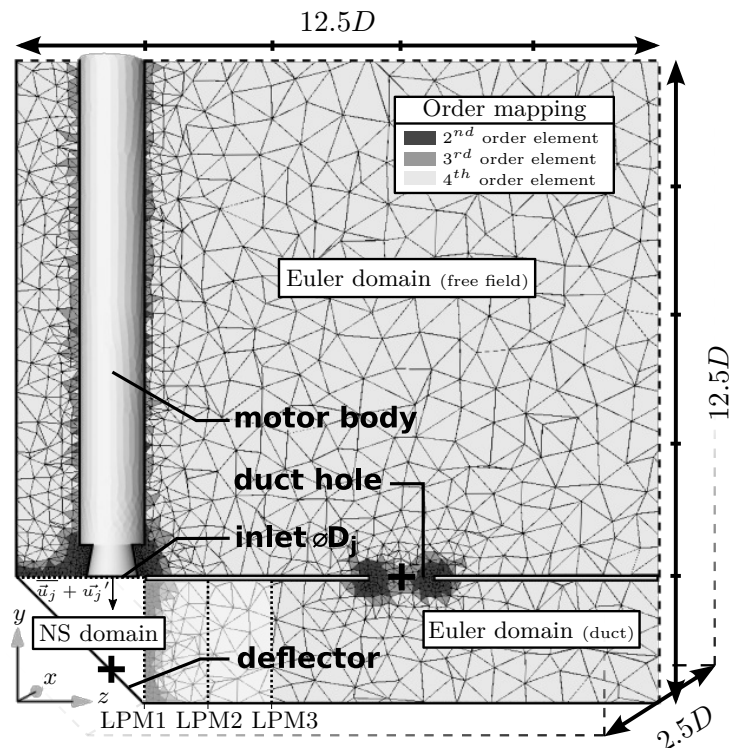
Figure 3.14: schéma du domaine de calcul du cas de carneau fictif et mappage d'ordre dans le domaine Euler. — : parois; - · - : condition de non-réflexion; · · · : interface de couplage pour les trois cas LPM1, LPM2 et LPM3; + : capteurs numériques.
