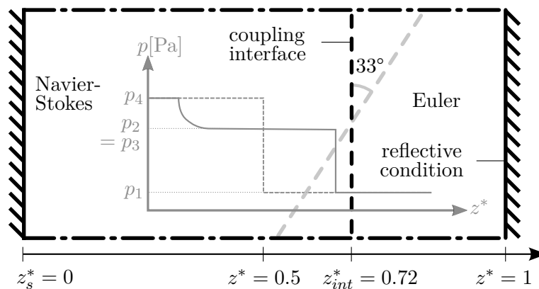
Figure 3.9: schéma du domaine de calcul du cas de tube à choc.
