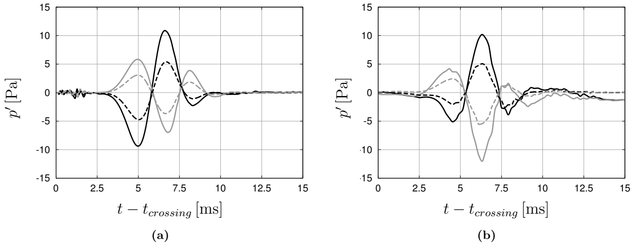
Figure 3.13: ondes de pression parasites générées au passage du tourbillon à l'interface (3.13a) Navier-Stokes→Euler en z_{int1} et (3.13b) Euler→Navier-Stokes en z_{int2} . \text{—} : A1 et B1 avec \Psi = 1 ; \text{- - -} : A1 et B1 avec \Psi = 0.5 ; \text{—} : A2 et B2 avec \Psi = 1 ; \text{- - -} : A2 et B2 avec \Psi = 0.5 .
