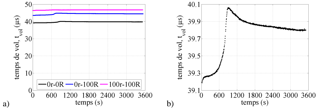
FIGURE 10.16 – Variation type du temps de vol au cours de l'essai d'arrachement : a) pleine échelle, b) échelle zoomée.
