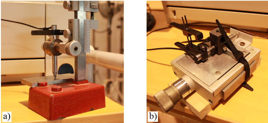
FIGURE E.2 – Instruments d'étalonnage des capteurs de déplacement : a) trusquin, b) vis de précision.
