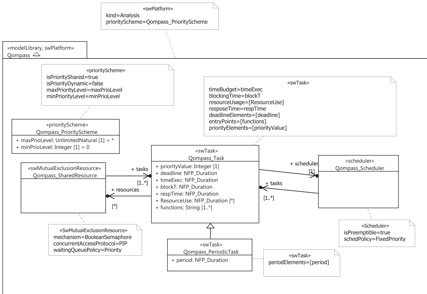
FIGURE B.1 – Modèle d'une configuration possible de la plateforme abstraite d'analyse associée à Qompass
