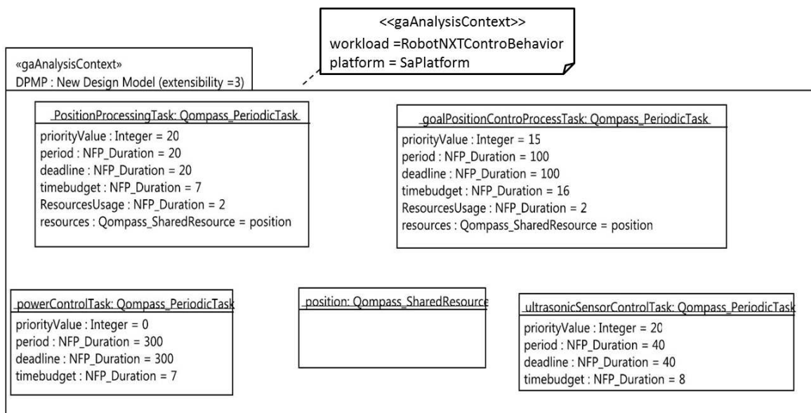
FIGURE 6.17 – Modèle de conception de l'application de contrôle de robot généré suite à l'application du patron DPMP
