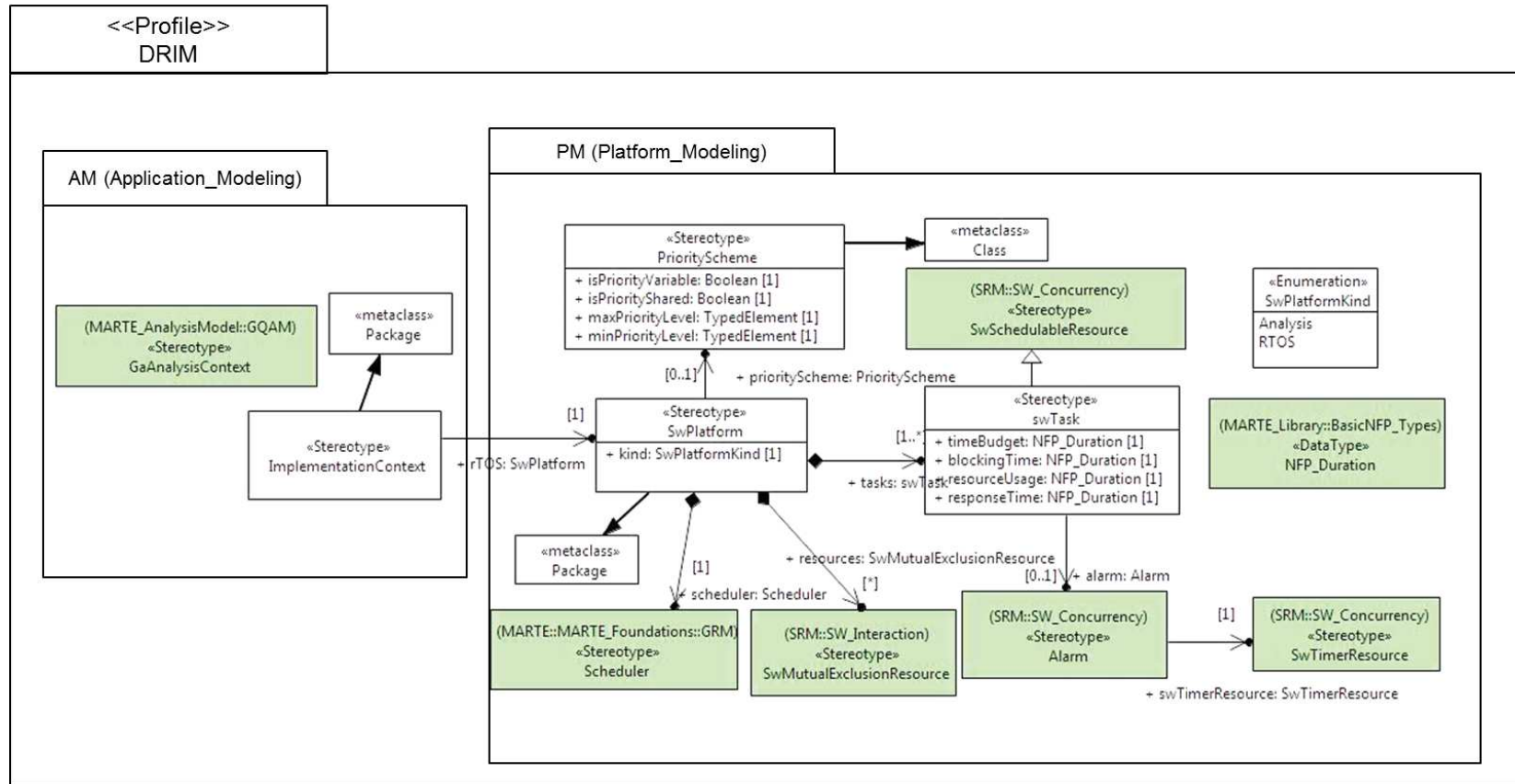
FIGURE 4.6 – Le profil DRIM : une extension du profil MARTE
