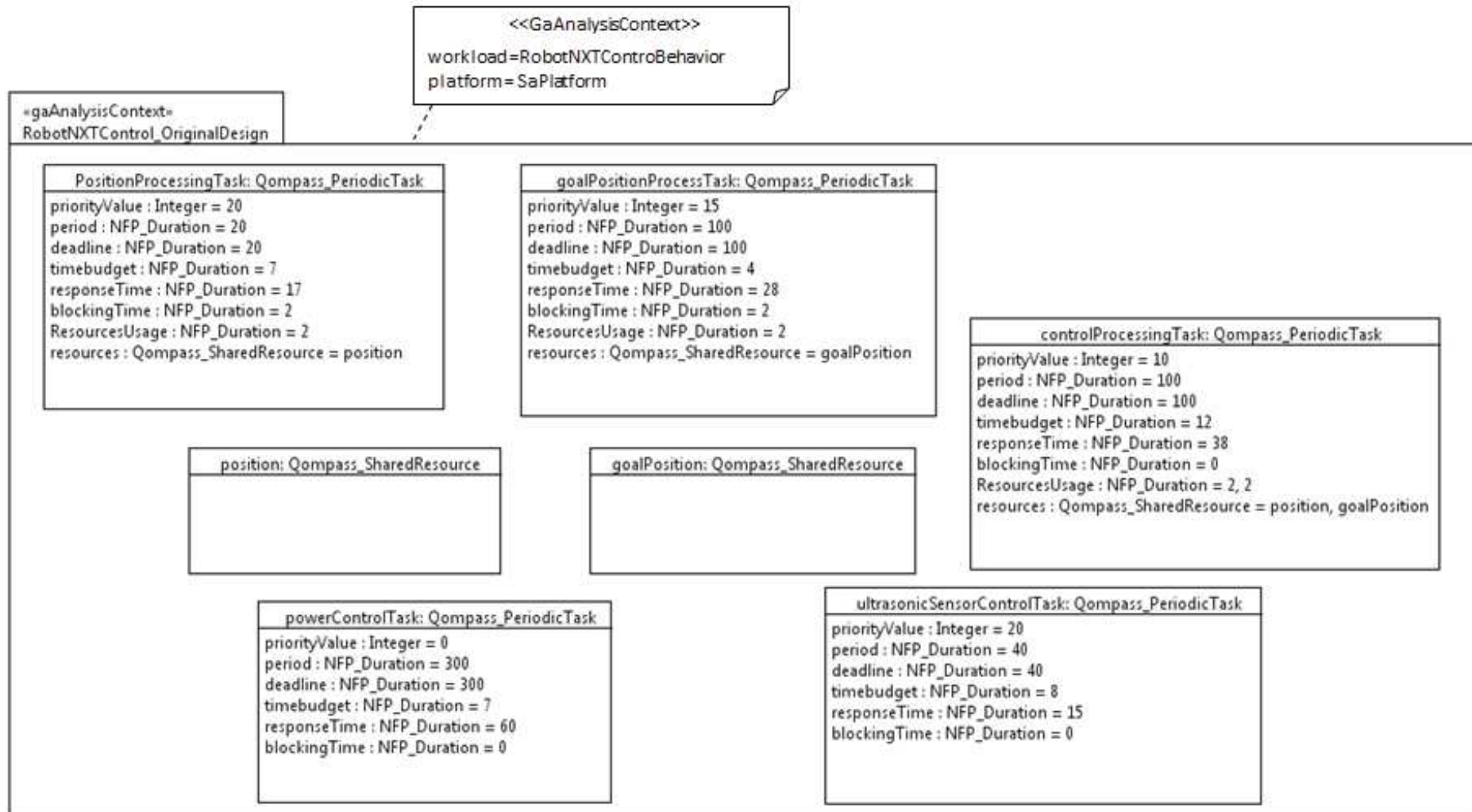
FIGURE 6.9 – Exemple de modèle de conception initial de l'application de contrôle du robot généré par Qompass-Architect
