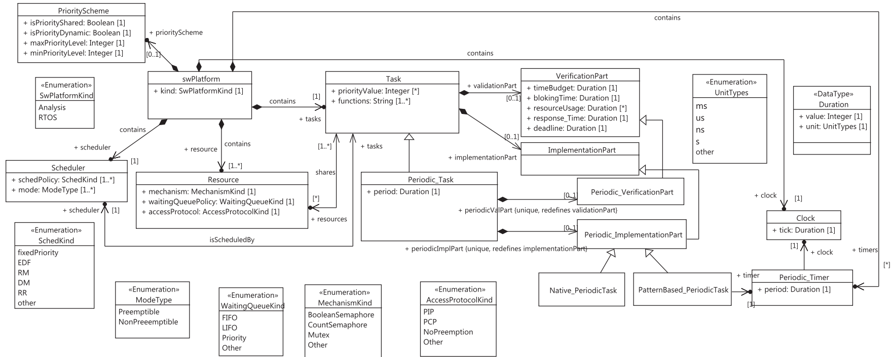
FIGURE 4.1 – Le méta-modèle DRIM pour la description des plateformes logicielles
