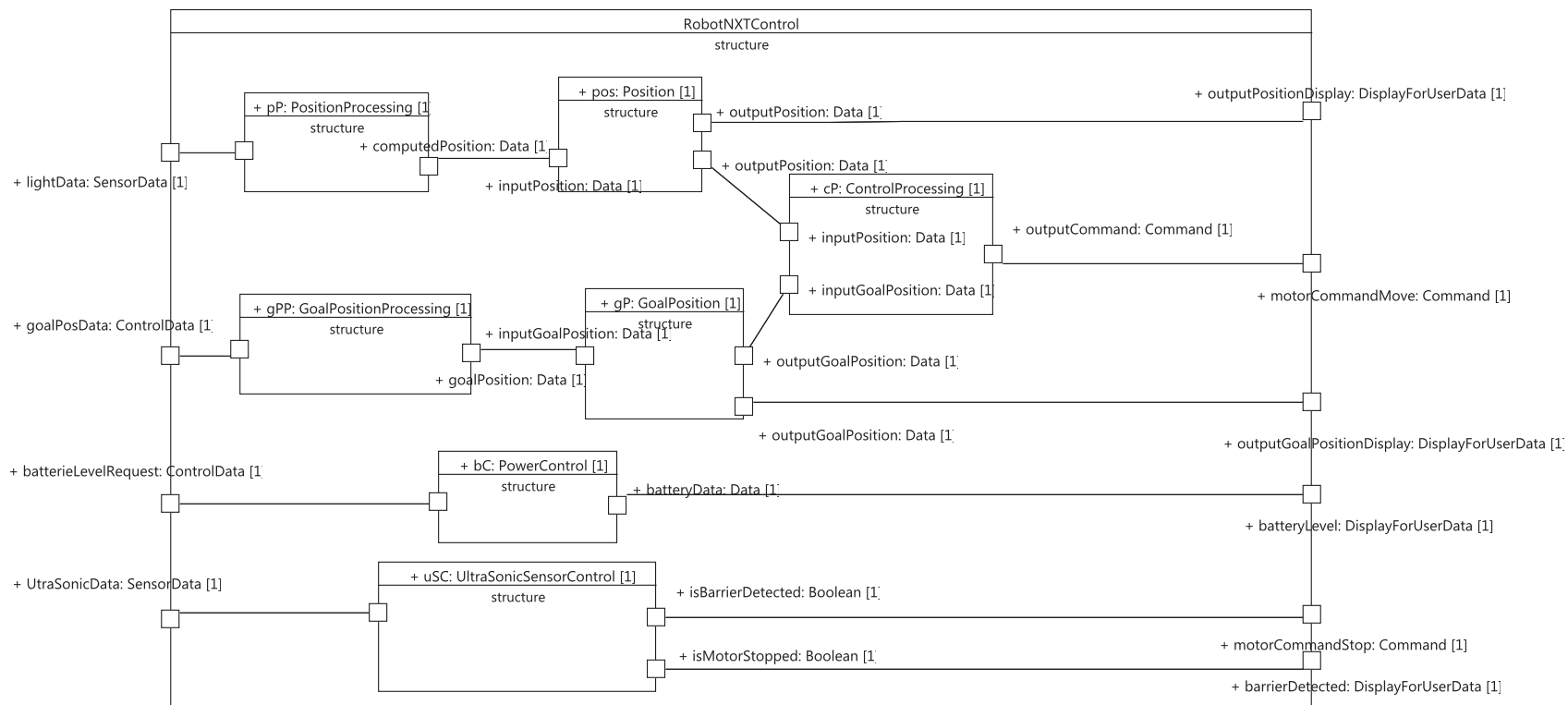
FIGURE 6.5 – Description fonctionnelle de l'application de contrôle de robot
