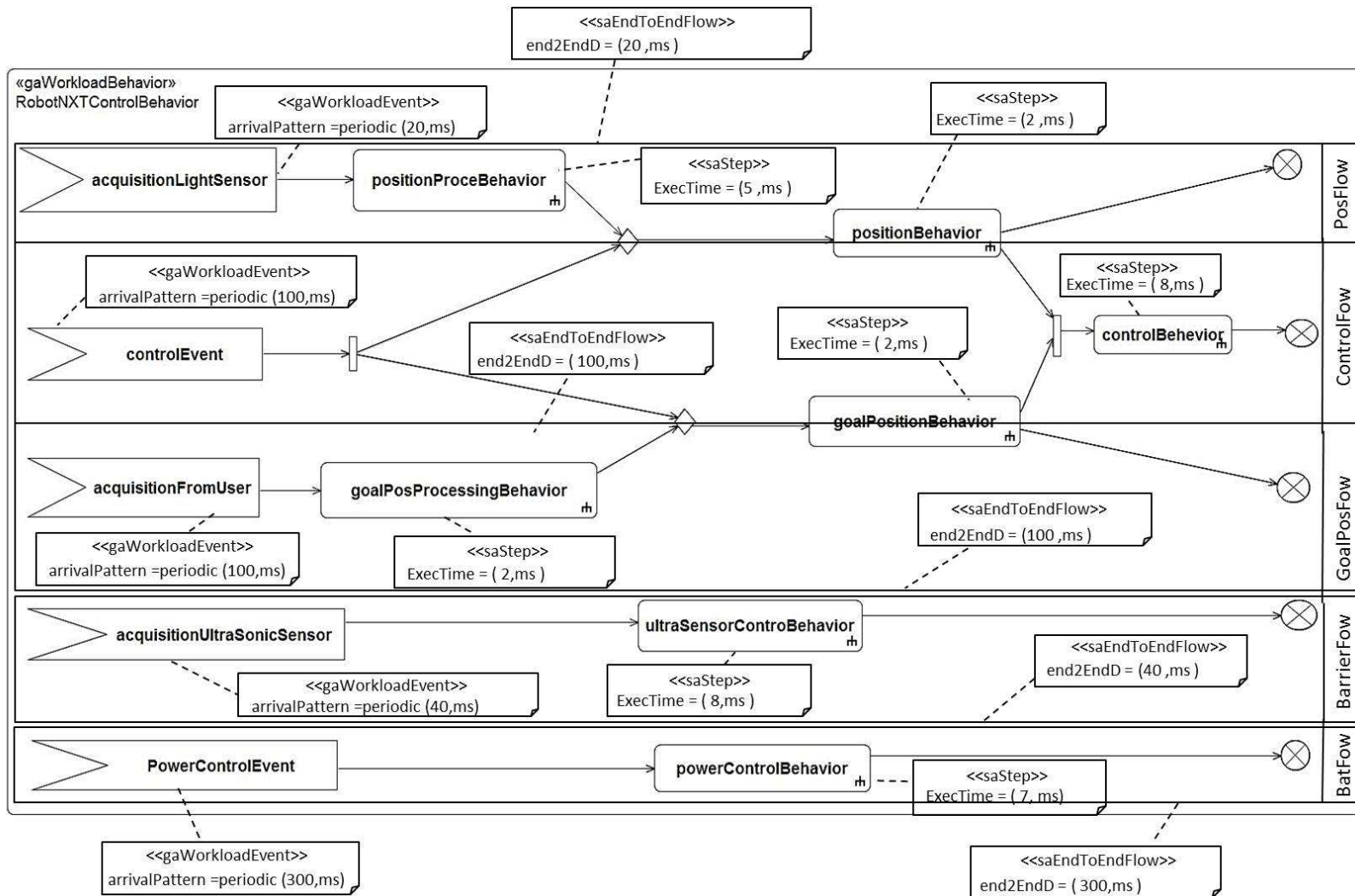
FIGURE 6.6 – Description comportementale niveau système de l'application de contrôle de robot
