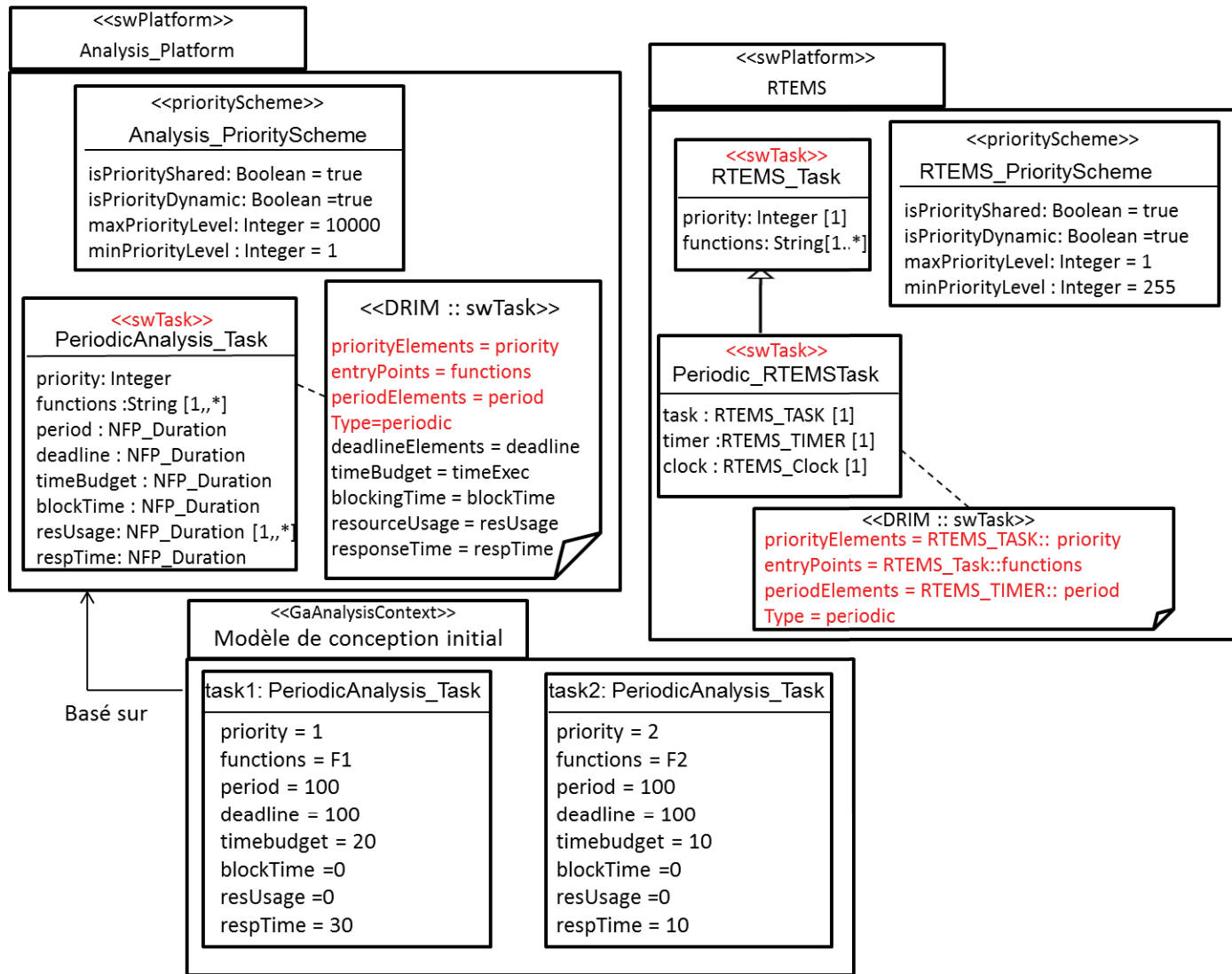
FIGURE 5.2 – Un exemple de modèle de conception, plateforme abstraite d'analyse et RTOS : entrées pour l'algorithme de portage
