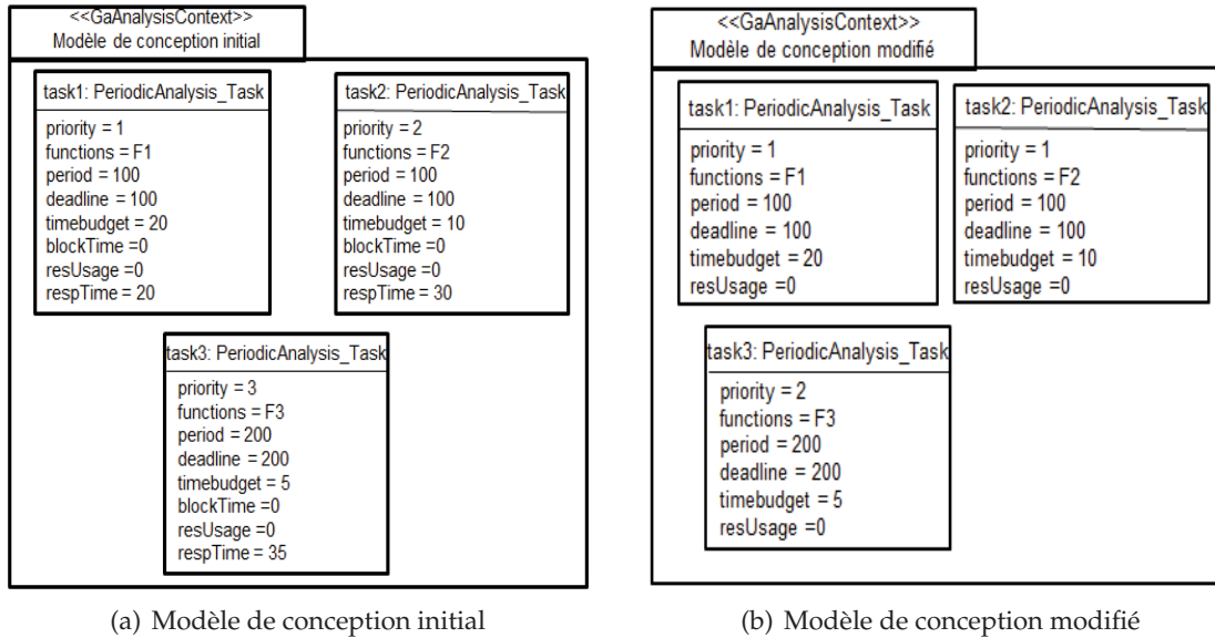
FIGURE 5.7 – Exemple d'application du patron NPAP
