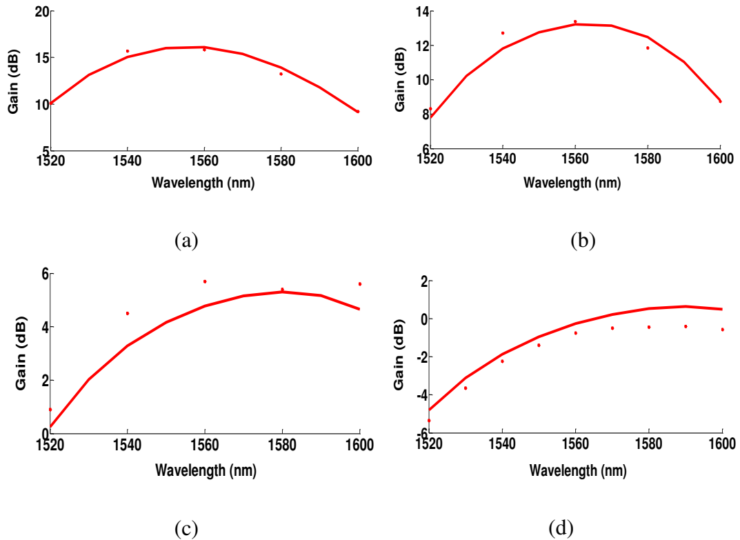
Figure R- 5 : Résultats de mesure (pointillés) et de simulation (ligne pleine) pour le gain du RSOA en fonction de la longueur d'onde avec un courant de polarisation de 70 mA et une puissance d'entrée de (a) -20 dBm (b) -10 dBm (c) de 0 dBm et (d) 4 dBm.
