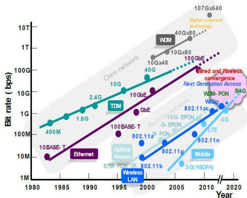
Figure R- 3 : Evolution du débit binaire dans les réseaux optiques cœur et d'accès.
