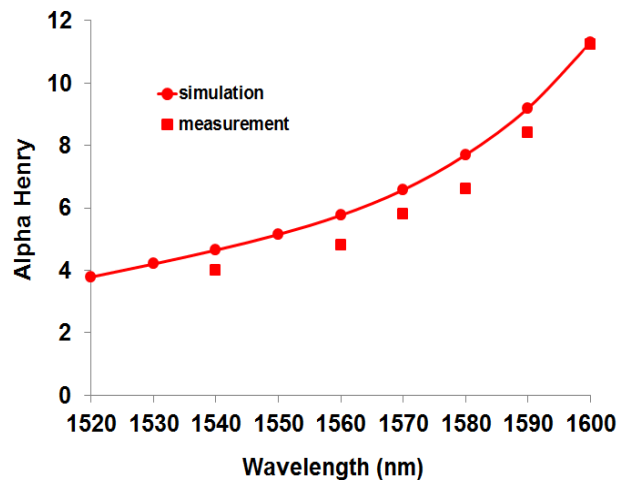
Figure R- 6 : Résultats de mesure et de simulation du facteur de couplage phase amplitude \alpha_H en fonction de la longueur d'onde avec un courant de polarisation de 80 mA et une puissance optique d'entrée de -7 dBm, le signal de pompe a une longueur d'onde de 1550 nm.
