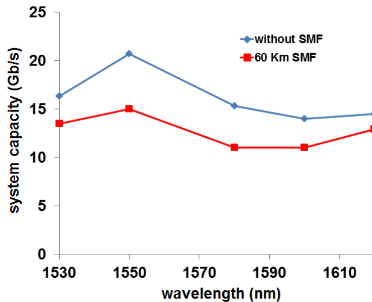
Figure R- 13 : Capacité de transmission en fonction de la longueur d'onde pour un signal converti AMOOFDM
