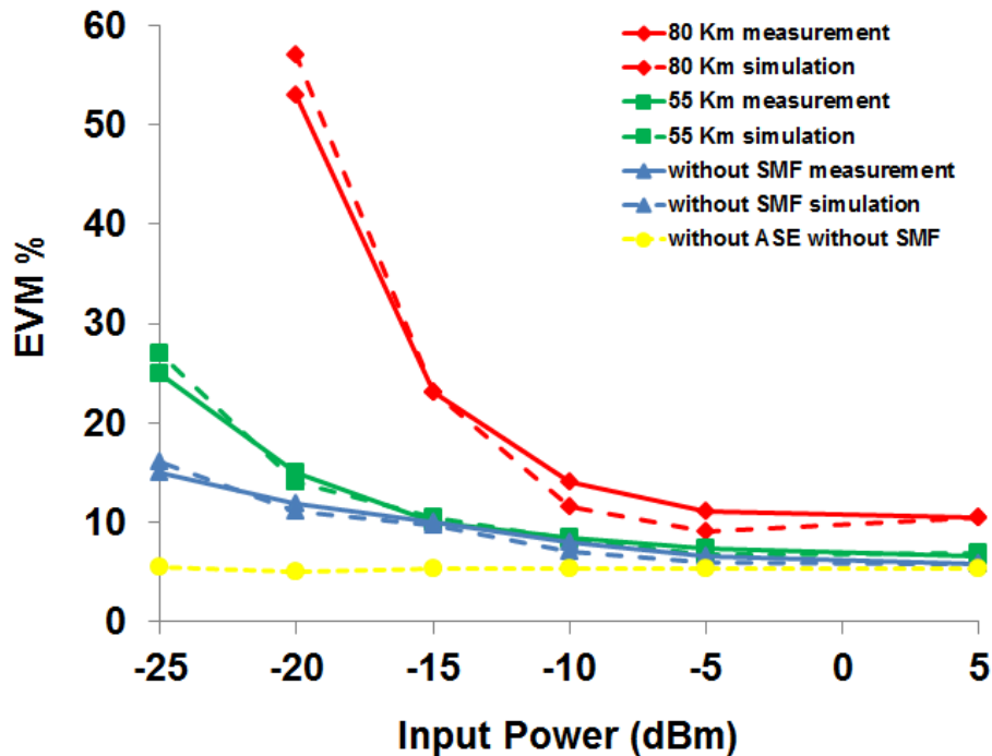
Figure R- 9 : EVM en fonction de la puissance d'entrée pour le signal 16 QAM - OOFDM pour différentes longueurs de fibre SMF. La largeur de la bande passante de signal est de 500 MHz, le RSOA est polarisé à 65 mA, le signal OOFDM est à 1570 nm, et le courant OFDM est de 7 mA.
