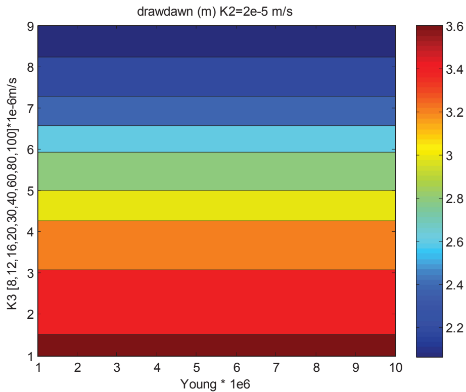
Figure 6. 20 : Variation du rabattement en fonction de K3, pour une valeur de K2 fixée. Le rabattement est en mètres.
