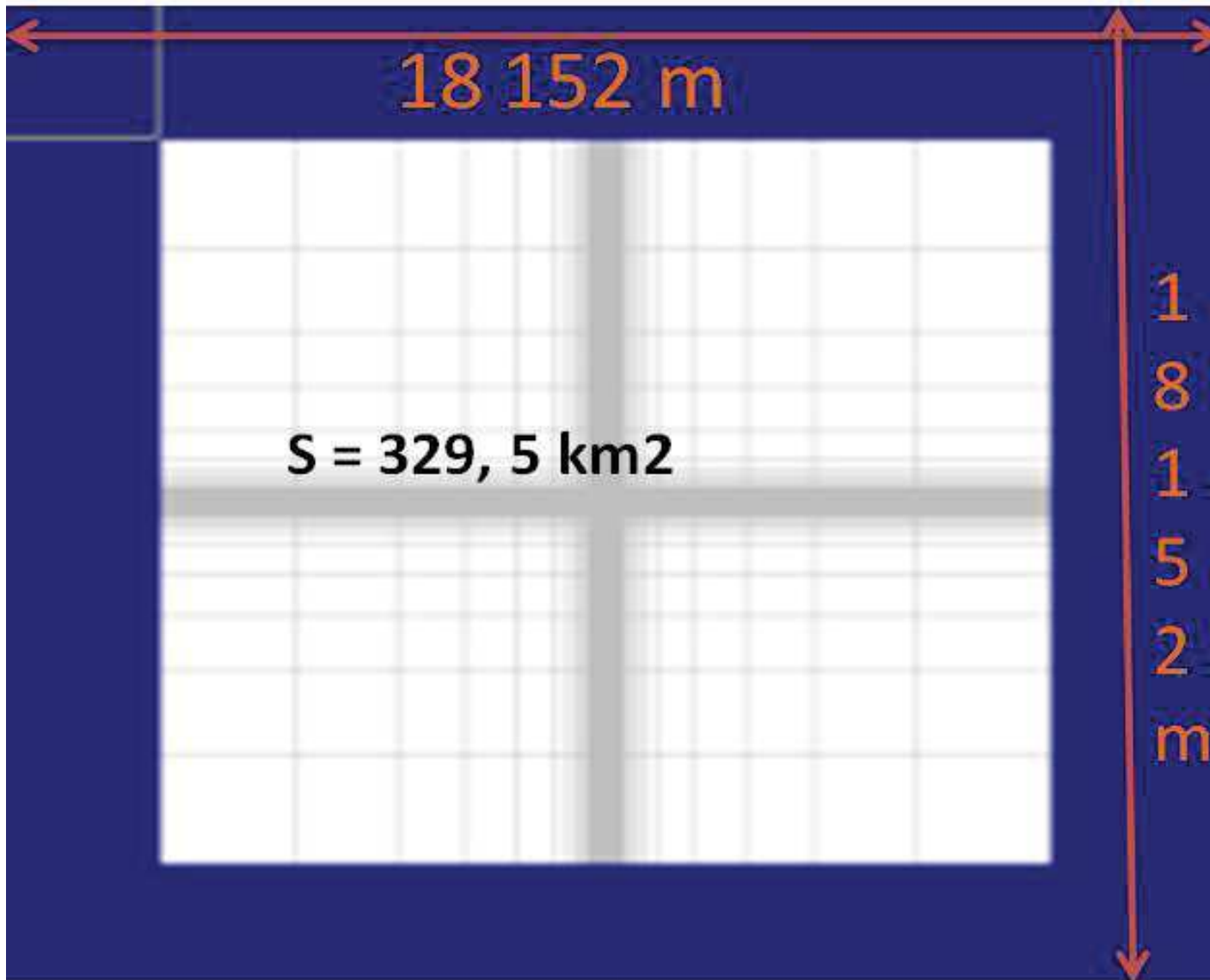
Figure 6.4 : Maillage rectangulaire à taille variable utilisé pour les modélisations.
