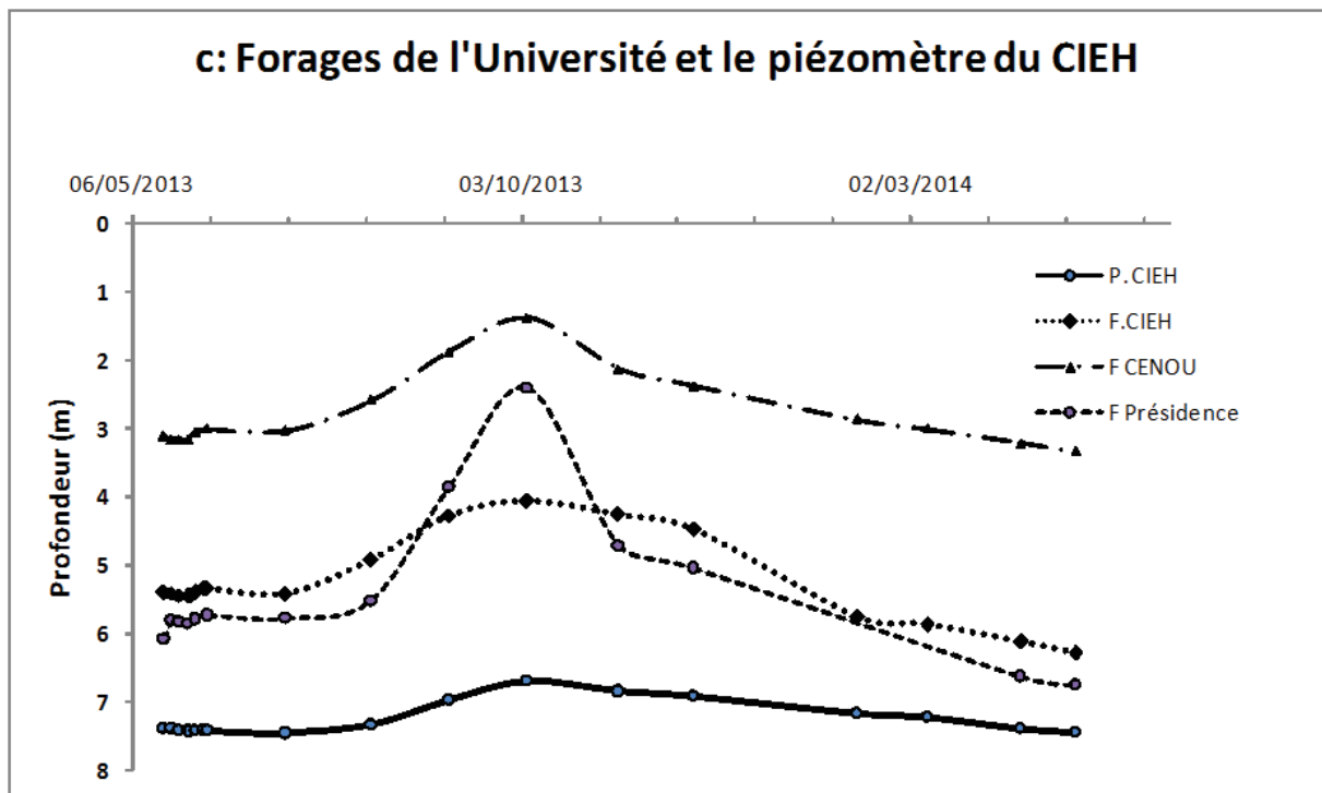
Figure 3.16 : Variations piézométriques sur l'année 2013 - 2014 dans trois parties de notre zone d'étude. a) la zone de Zogona : puits PP1,...PP7 ; b) le site de l'université : piézo CIEH, forage CIEH, forage Cenou et forage Présidence ; c) le parc Bangr Weogo: puits Rocaille et Pépinière. Pour chaque sous figure l'échelle verticale (hauteur piézométrique) est différente et le piézomètre du CIEH est figuré, à titre de comparaison.
