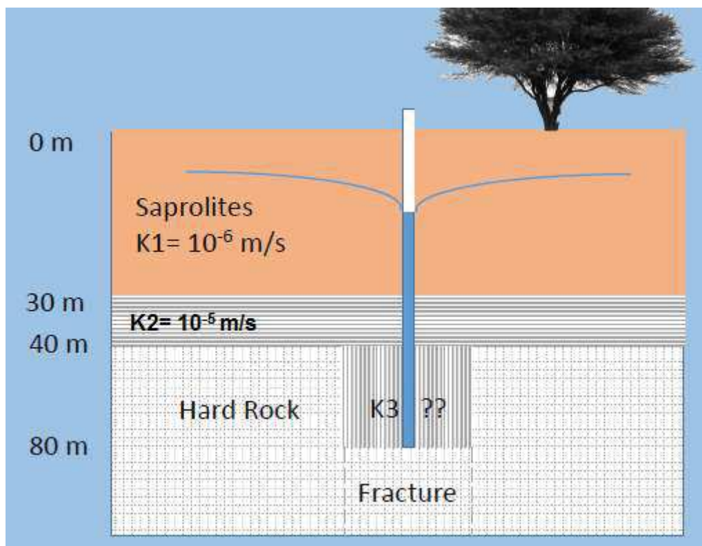
Figure 6.1 : Le modèle schématisé de l'aquifère de socle granitique. La géométrie de la couche fissurée est censée être connue par l'exploration géophysique. La largeur de la faille est supposée égale à 40 m.
