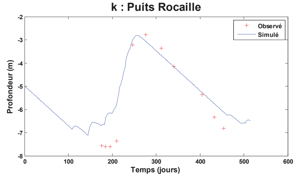
Figure 4.2 : Simulations des niveaux piézométriques pour les sites de l'Université de Ouagadougou (a, b, c, d); du quartier Zogona (e, f, g h, i) et du parc Bangr Weogo (j, k)
