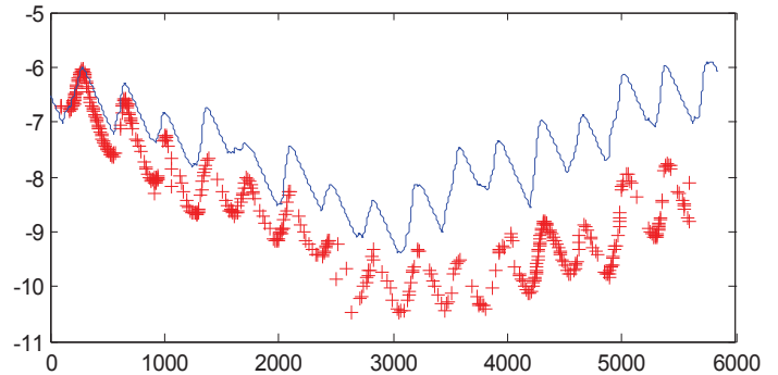
Sensibilité : Ruissellement - 5%
