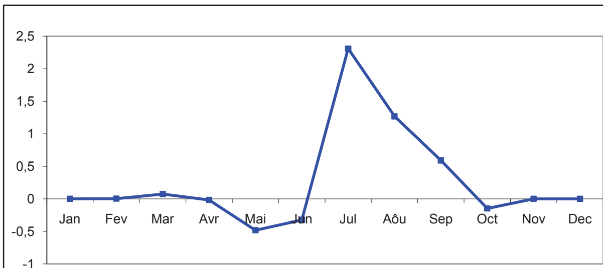
Figure 3. 9 : Variation des coefficients directeurs des droites linéaires des précipitations mensuelles.
