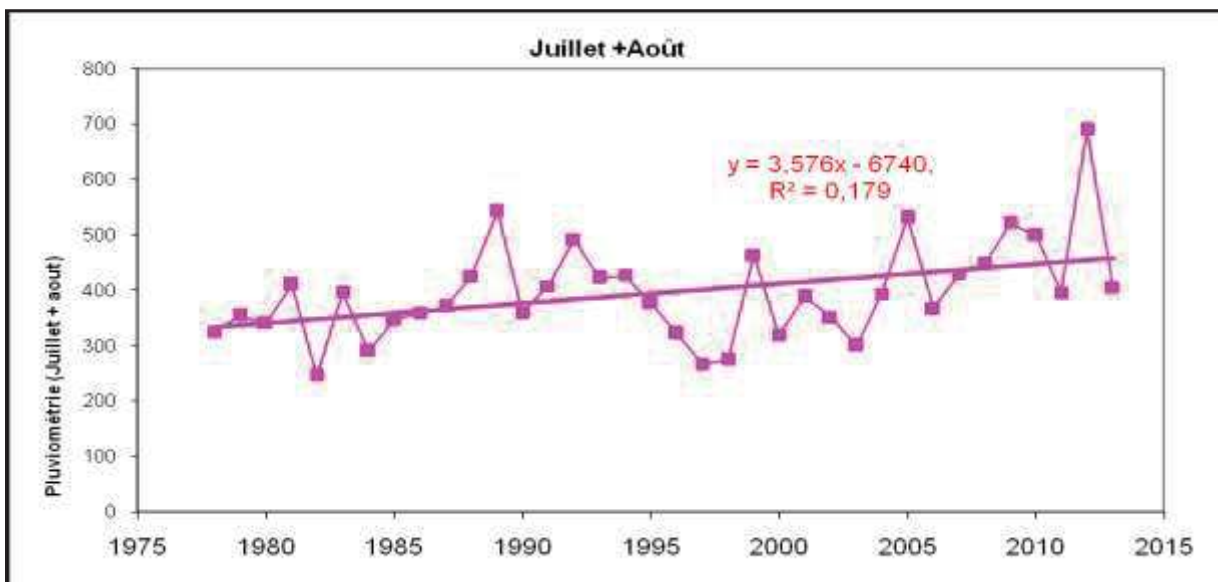
Figure 3. 7 : Précipitation cumulée des mois de Juillet et Août (1978-2013).
