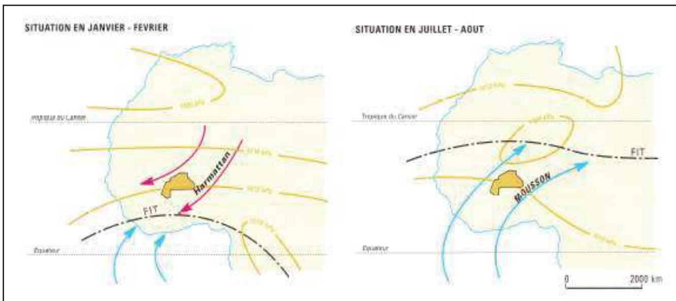
Figure 3.14 : le déplacement du FIT en Afrique de l'Ouest (source : Laclavère 1993).
