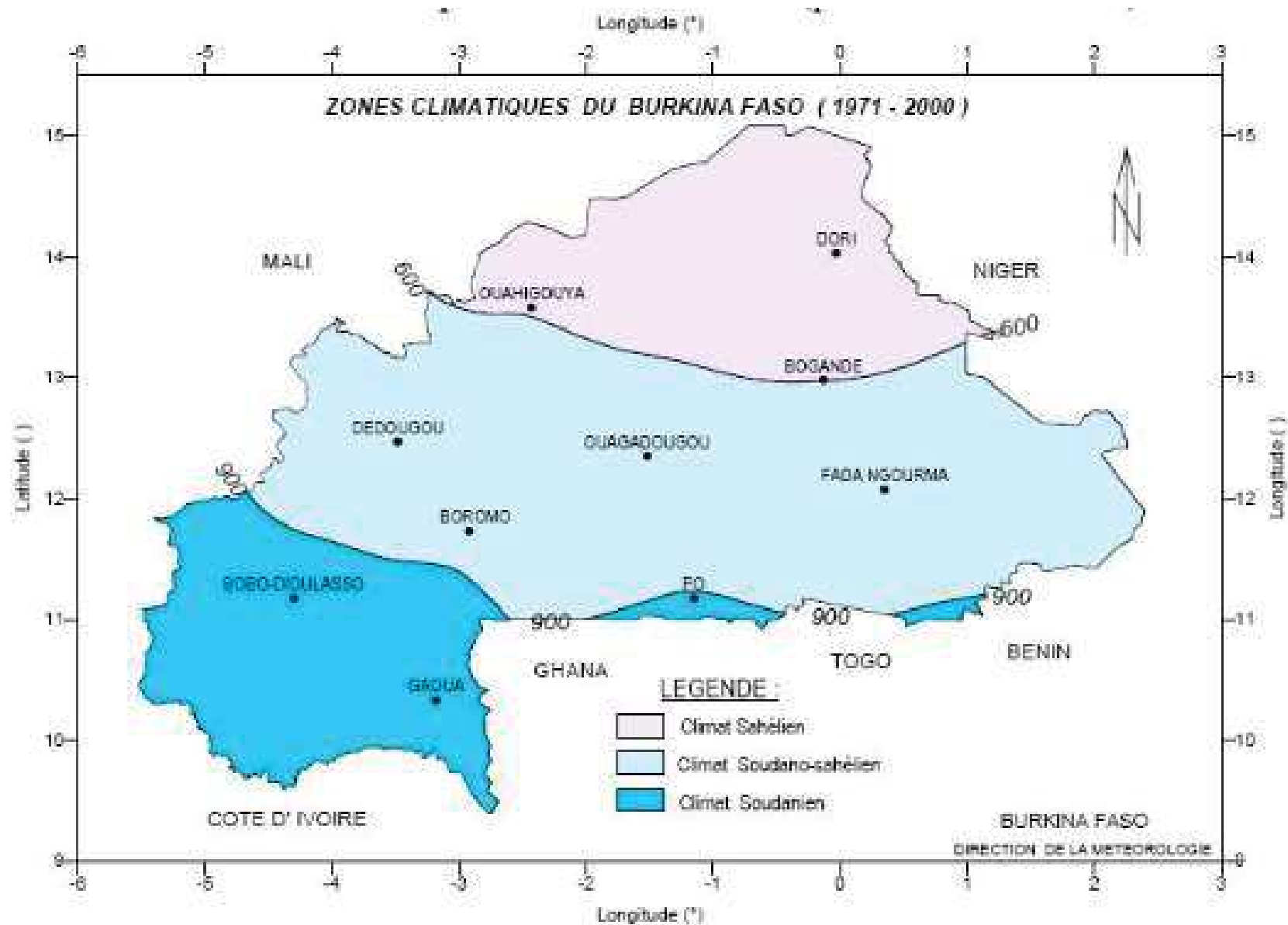
Figure 3.1: les zones climatiques du Burkina Faso (source direction de la météorologie Burkina Faso).
