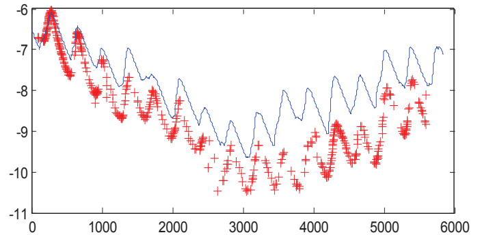
Sensibilité : Perte - 5%
