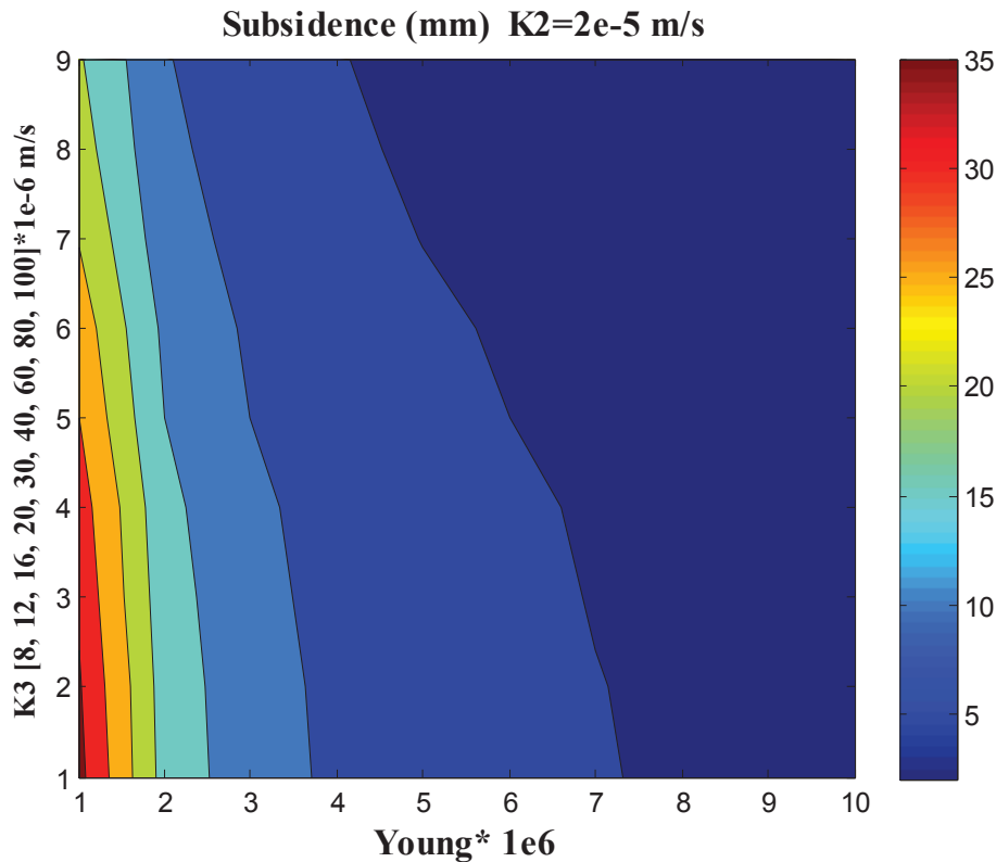
Figure 6.22 : Variation de la subsidence en (mm) en fonction du rapport K3 et du module d'Young en (Pa), pour une conductivité K2 fixée.
