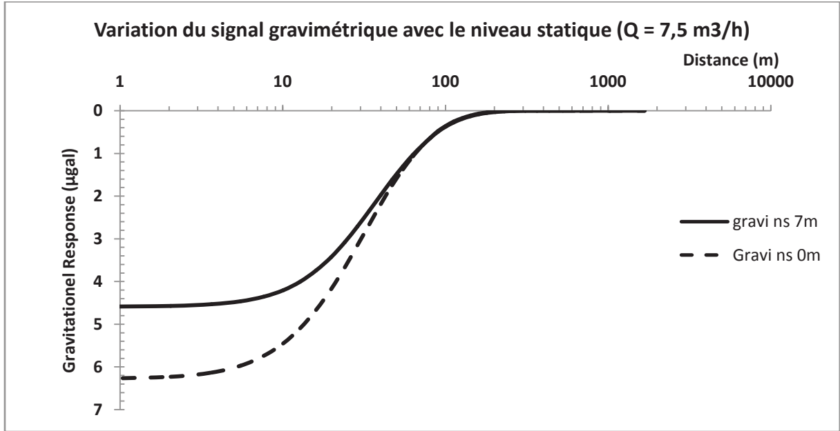
Figure 6.14 : Signal gravimétrique modélisé pour différents niveaux statiques avec pompage dans le milieu fissuré (cas 2).
