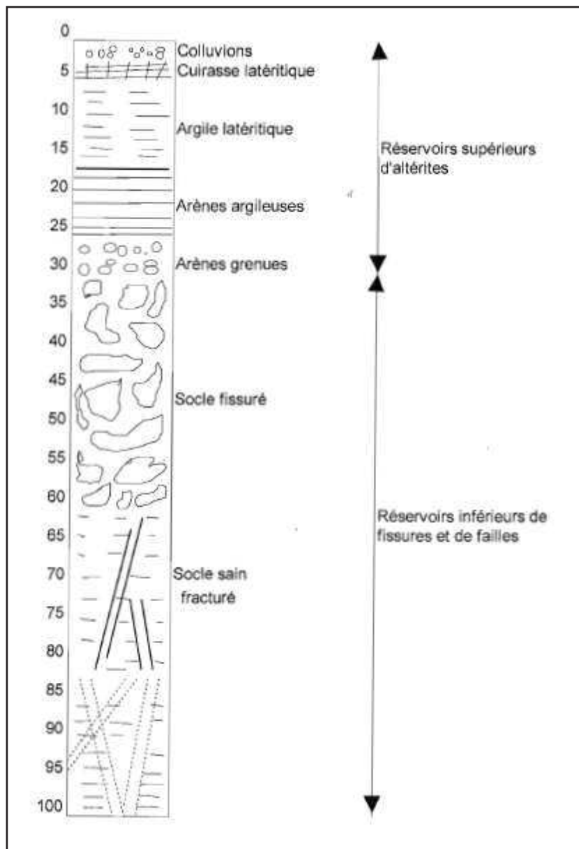
Figure 2. 4 : Schéma hydrogéologique type de l'ensemble altérites/socle au Burkina Faso (Source : Compaoré 1997).
