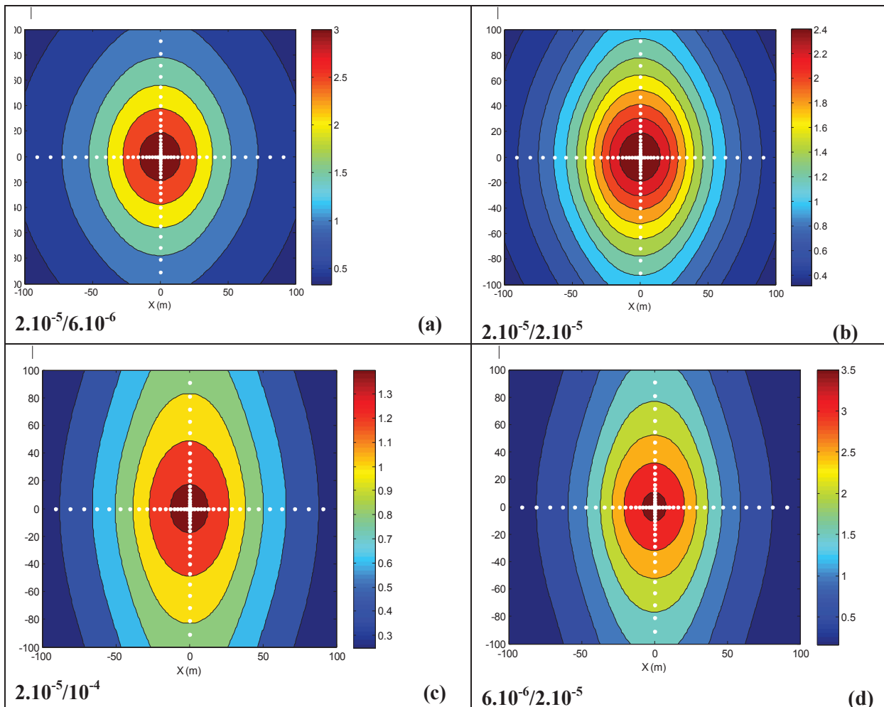
Figure 6. 19 : Rabattement en fonction du rapport ( K_2/K_3 ) des conductivités de la couche basale des altérites et celle de la faille. Les conductivités sont exprimées en m/s et le rabattement en m.
