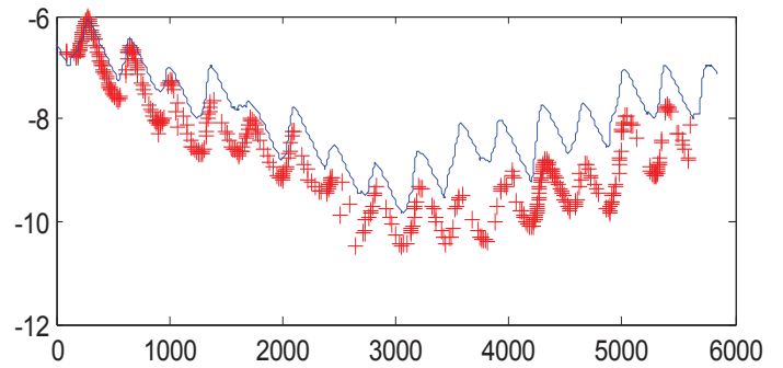
Sensibilité : Porosité - 5%
