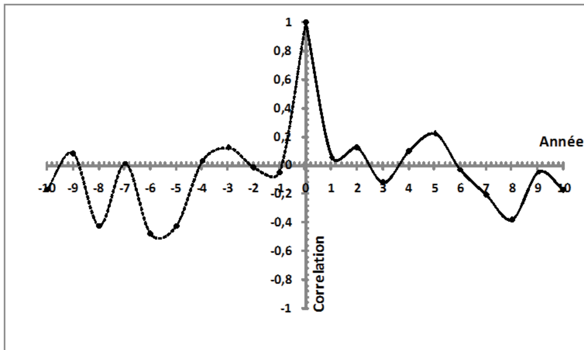
Figure 3.19: Autocorrélation des précipitations.
