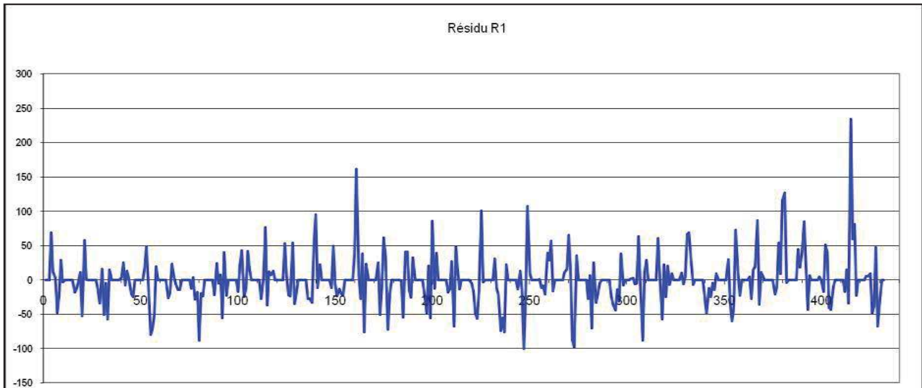
Figure .3. 12 : Ecart entre le modèle saisonnier et le modèle réel des précipitations mensuelles.
