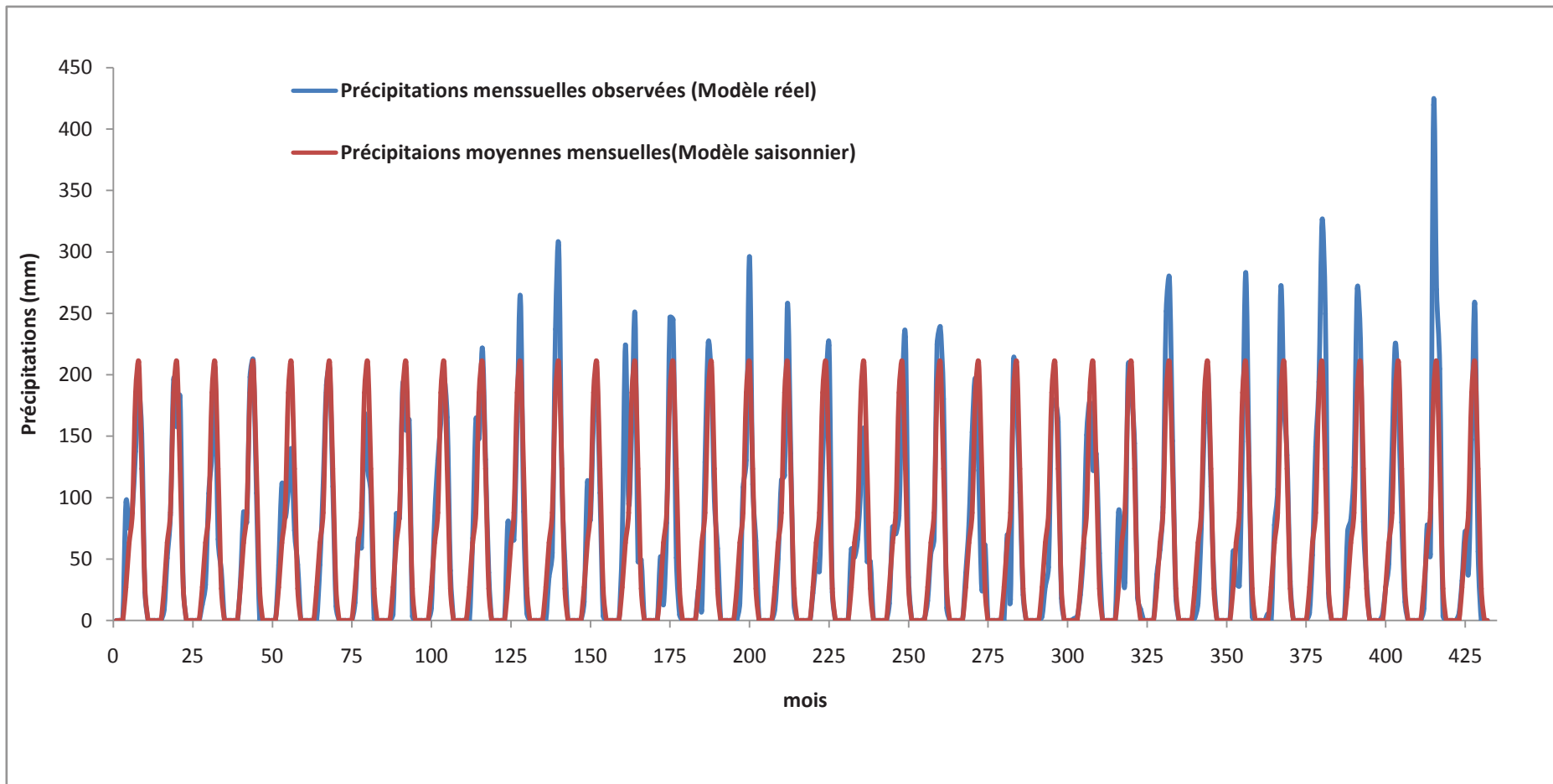
Figure .3.11 : Les modèles saisonnier et réel des précipitations mensuelles.
