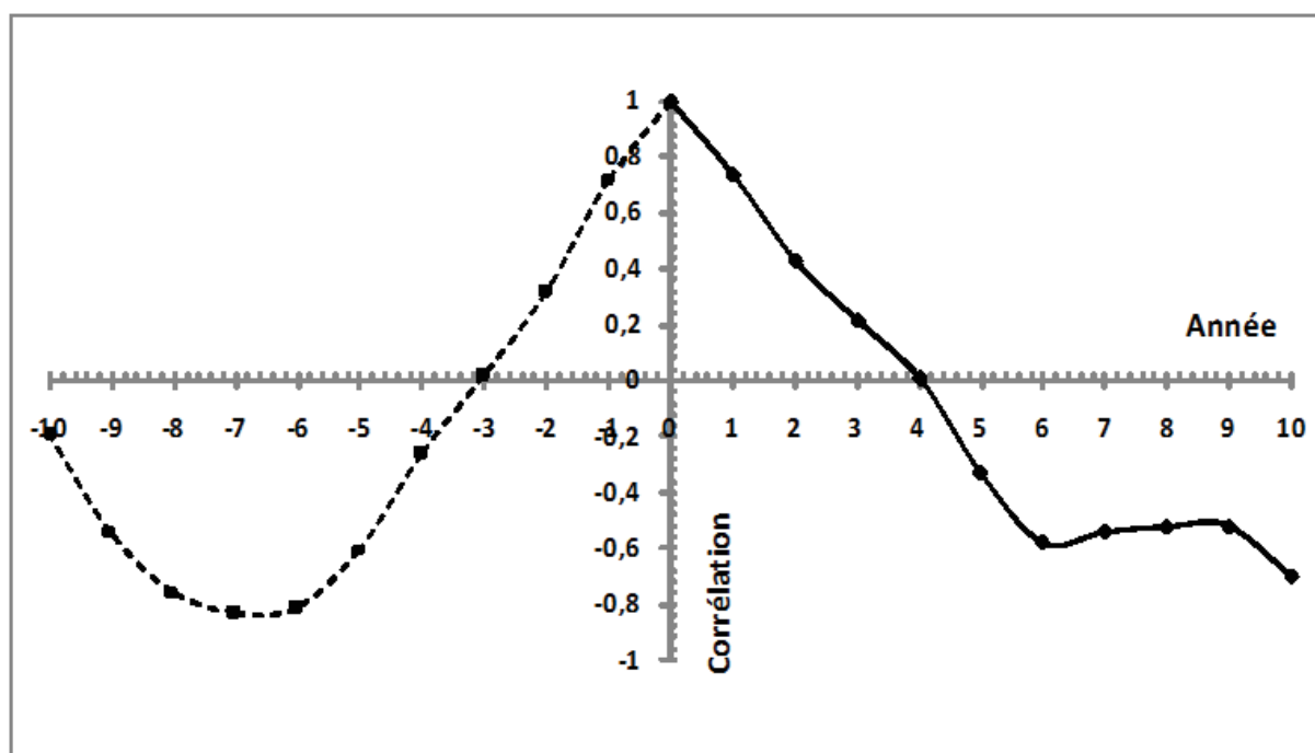
Figure 3.20 : Autocorrélation du niveau moyen du piézomètre du CIEH.
