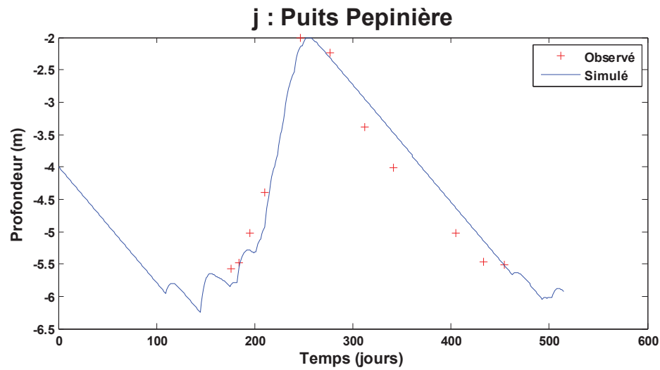
Figure 4.2 : Simulations des niveaux piézométriques pour les sites de l'Université de Ouagadougou (a, b, c, d); du quartier Zogona (e, f, g h, i) et du parc Bangr Weogo (j, k)
