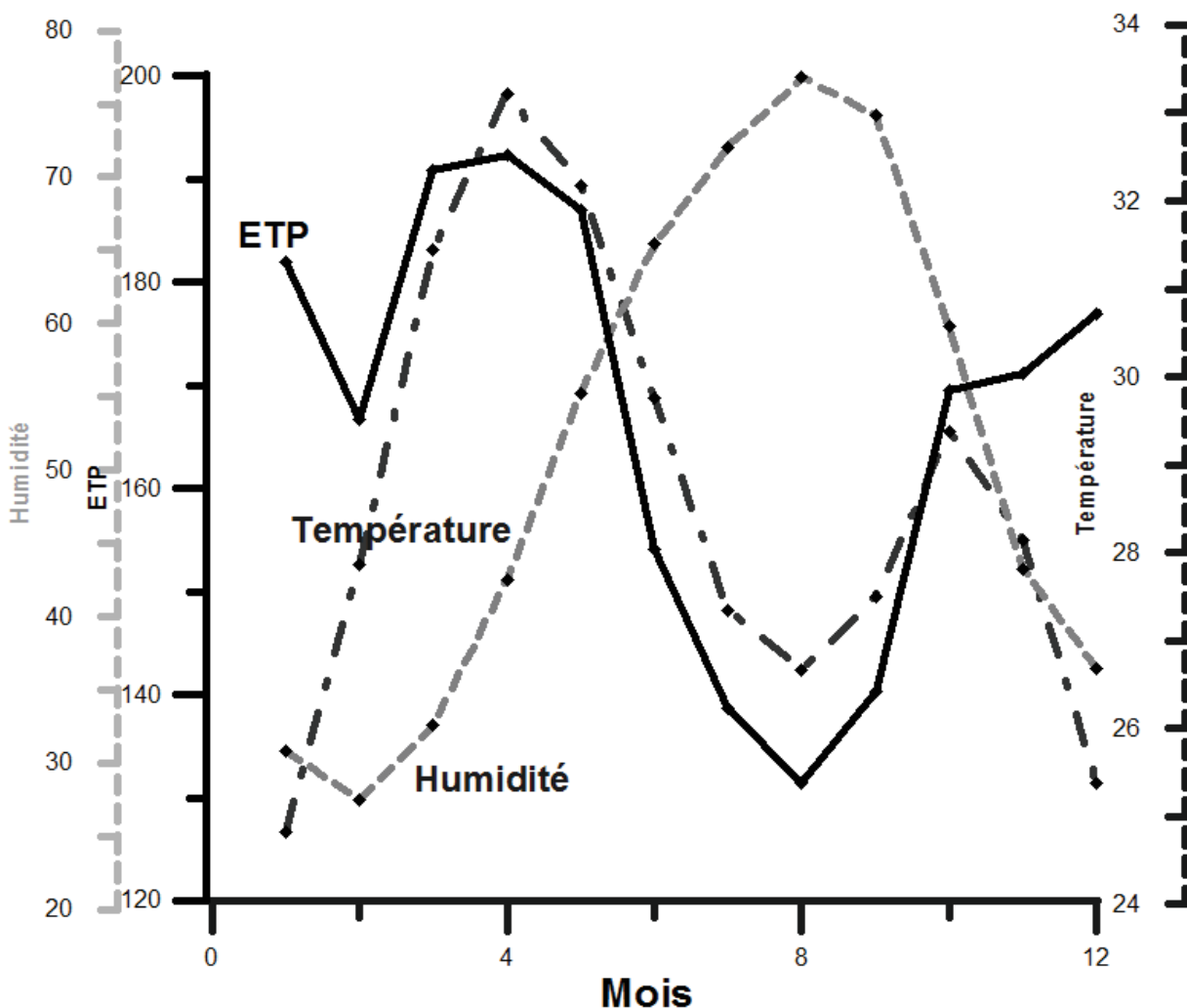
Figure 3. 13 : Variation mensuelle de la température (période : 1978 - 2012), de l'ETP (période : 1978 - 1990) et de l'humidité relative (période : 1961 - 1978) à Ouagadougou.
