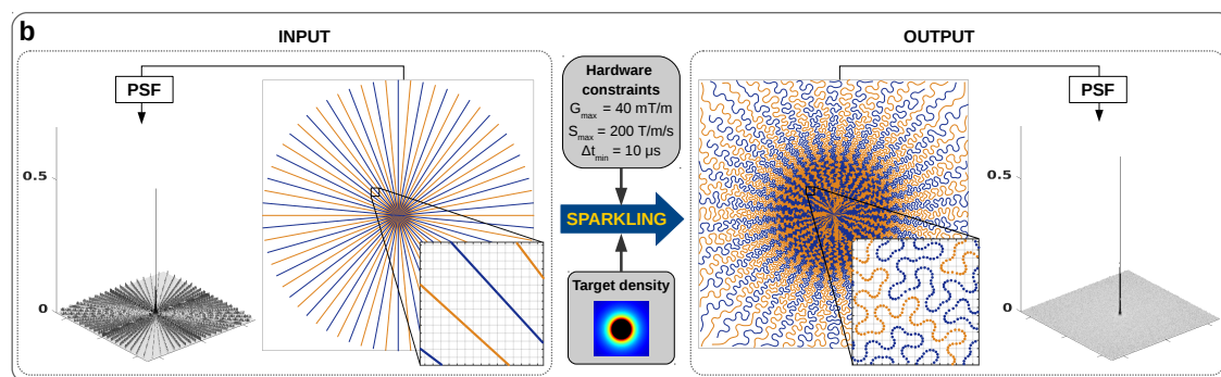
FIGURE 2: Génération des trajectoires SPARKLING. L'amplitude maximale du gradient et sont slew rate sont G_{max} = 40 \text{ mT/m} et S_{max} = 200 \text{ T/m/s} respectivement. La durée de chaque segment était de 30.72 ms. La méthode SPARKLING appliquée sur des lignes radiales pour une densité variable pour N = 512 et 34 segments symétriques ( AF = 15 , R = 2.5 ).
