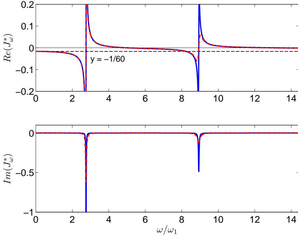
FIGURE 3.6 – Parties réelle et imaginaire de l’inertie de rotation apparente adimensionnelle de la plaque J_\omega^* en fonction de la pulsation adimensionnelle \omega/\omega_1 ; avec amortissement structural \eta = 0.5\% (—) , et \eta = 2\% (---)
