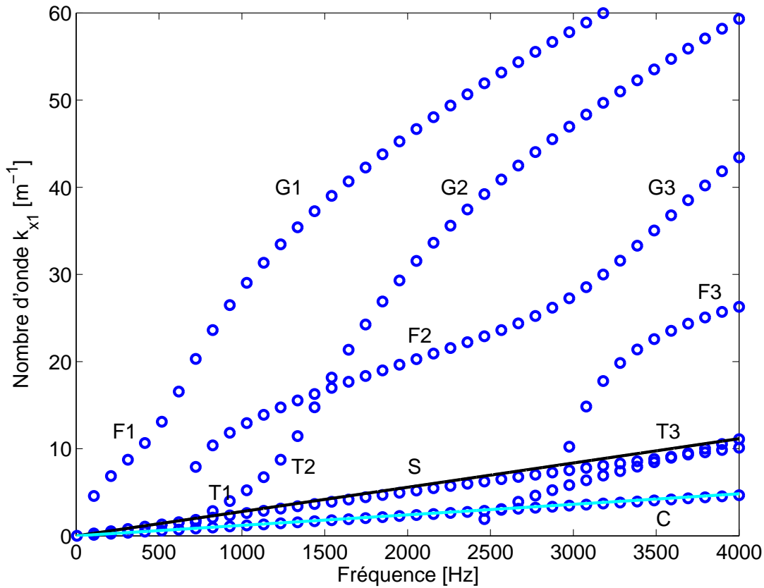
FIGURE 5.5 – Courbes de dispersion calculées par WFEM ( -+ ) et CWFEM ( \circ ), pour la plaque \mathcal{R}_1 . Nombres d'onde de cisaillement ( - ) et de compression ( - ) estimés par (5.1).
