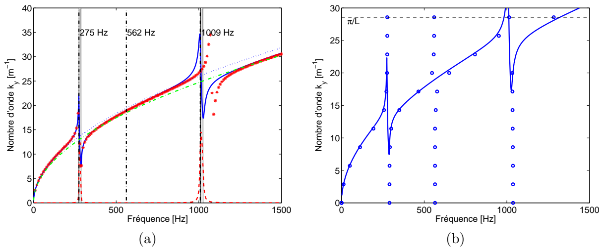
FIGURE 5.28 – Courbe de dispersion de flexion dans la plaque bi-raidie : (a) Nombres d'onde (partie réelle (—) et partie imaginaire (---)). Nombre d'onde de flexion dans le treillis \mathcal{G} seul (---), et dans le treillis avec masse de la plaque interne inerte ( \cdots ). Approximation plaque circulaire (*). Les intervalles de masse effective négative sont représentés en gris (■); (b) Courbe de dispersion analytique (—), et calcul éléments finis WFEM (○)
