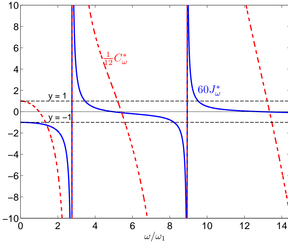
FIGURE 3.8 – Partie réelles de l’inertie de rotation apparente adimensionnelle normalisée \langle \frac{x_2}{D} \psi_\omega \rangle (—), et de la rigidité de torsion apparente adimensionnelle normalisée D^3 \partial_{x_2}^3 \psi_\omega |_{\frac{D}{2}} (---) en fonction de la pulsation adimensionnelle \omega/\omega_{t1}
