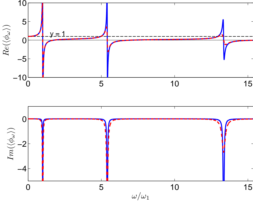
FIGURE 3.3 – Parties réelle et imaginaire de la masse apparente adimensionnelle \langle \phi_\omega \rangle de la plaque en fonction de la pulsation normalisée \omega/\omega_{s1} , avec amortissement matériel \eta = 0.5\% (—), et \eta = 2\% (---).
